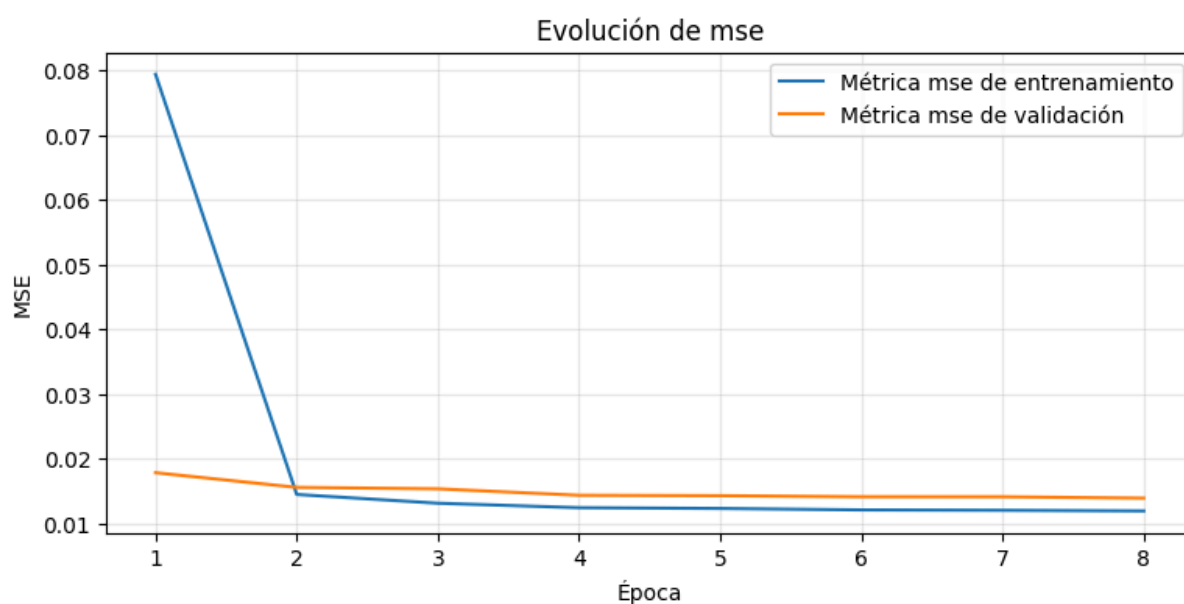
Figura 5.87. Evolución del MSE durante el entrenamiento del modelo basado en una capa Bidireccional
