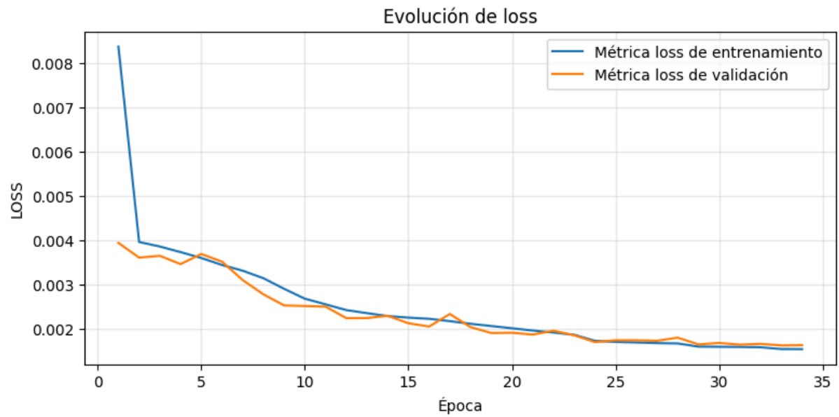
Figura 5.55. Evolución de la pérdida durante el entrenamiento del modelo convolucional U-Net
