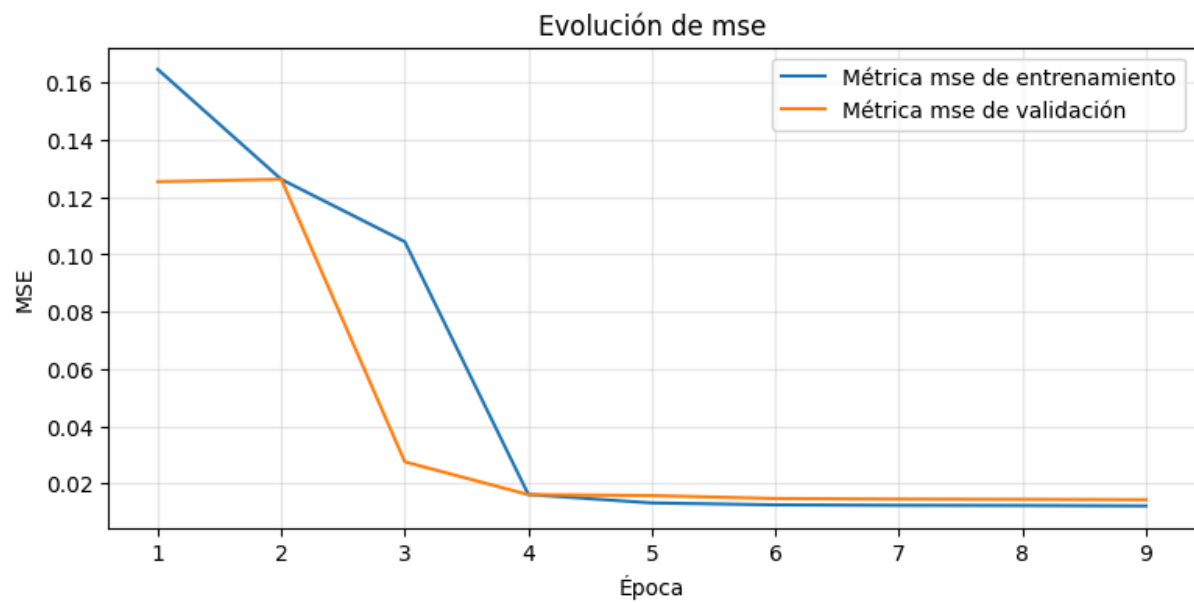
Figura 5.98. Evolución del MSE durante el entrenamiento del modelo basado en el mecanismo de Atención
