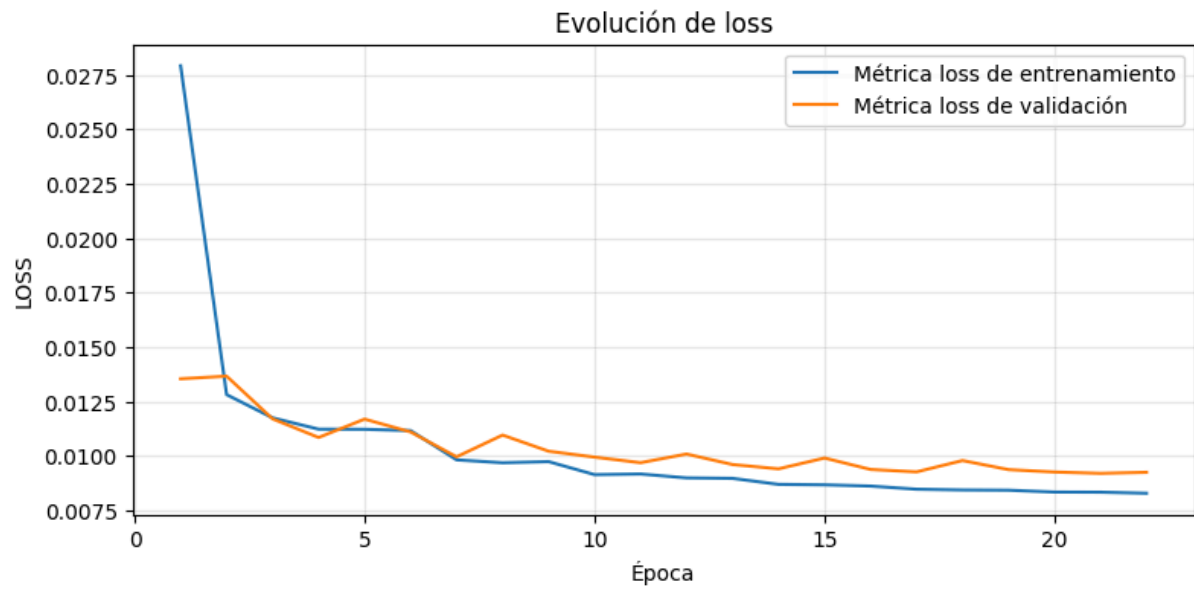
Figura 5.2. Evolución de la pérdida durante el entrenamiento
