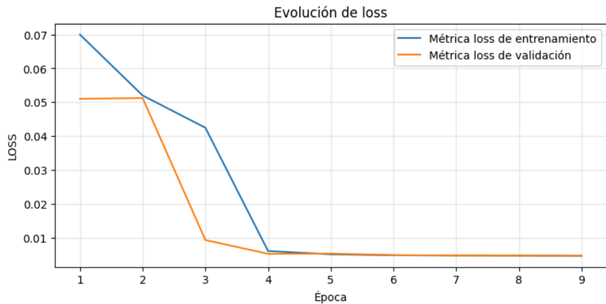
Figura 5.96. Evolución de la pérdida durante el entrenamiento del modelo basado en el mecanismo de Atención
