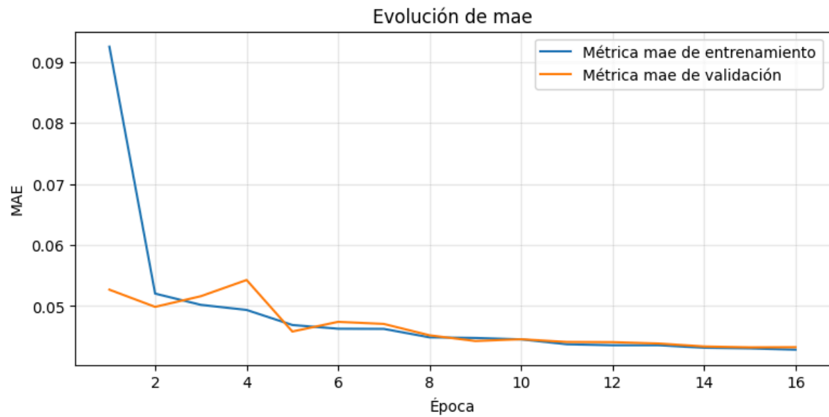
Figura 5.15. Evolución del MAE durante el entrenamiento de la red densa con normalización basada en la mediana
