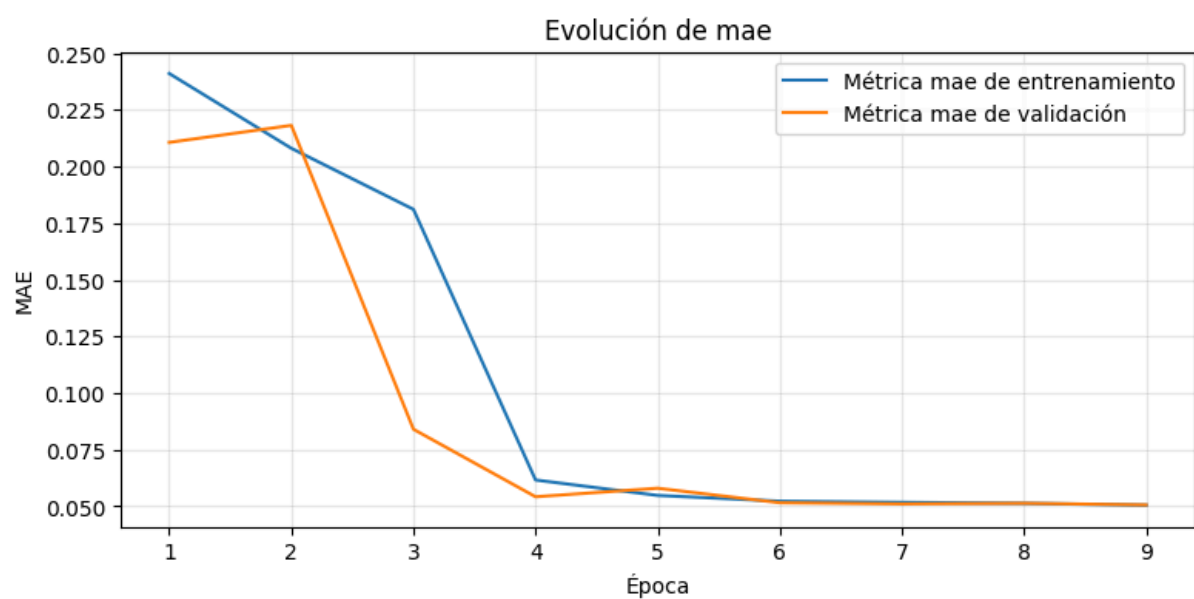
Figura 5.97. Evolución del MAE durante el entrenamiento del modelo basado en el mecanismo de Atención
