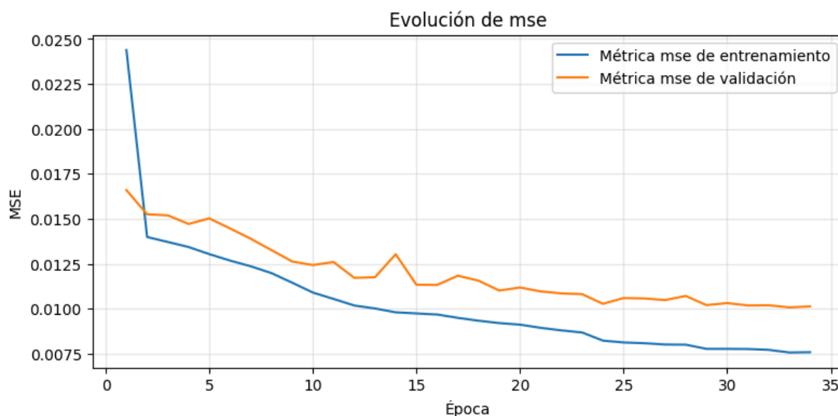
Figura 5.57. Evolución del MSE durante el entrenamiento del modelo convolucional U-Net
