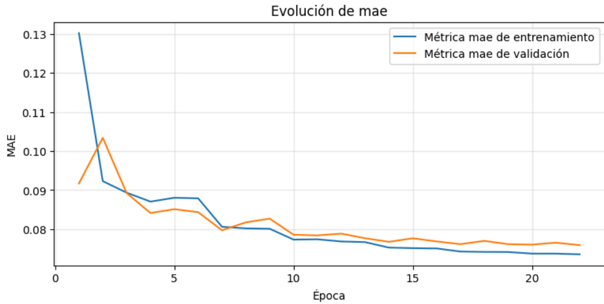
Figura 5.4. Evolución del MAE durante el entrenamiento
