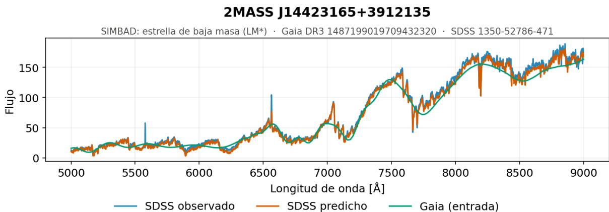
Figura 5.29. Secuencia central, baja luminosidad y baja temperatura, ejemplo 2. Espectro generado por el modelo de redes neuronales densas con normalización basada en el máximo de cada espectro para uno de los objetos del extremo frío de la secuencia, con estrellas de baja masa de unos 3 100 K y paralajes de entre 8 y 27 mas, es decir, objetos cercanos y poco luminosos.
