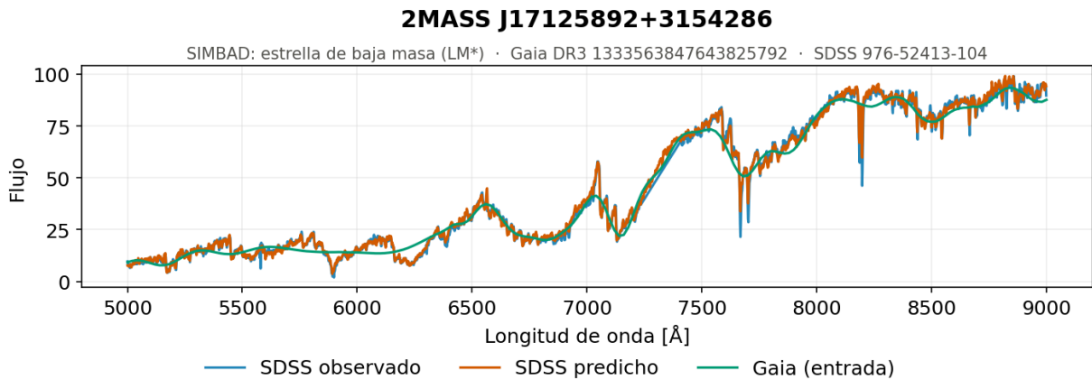
Figura 5.40. Secuencia central, baja luminosidad y baja temperatura, ejemplo 1. Espectro generado por el modelo de redes neuronales densas con la SNR de Gaia como entrada para uno de los objetos del extremo frío de la secuencia, con estrellas de baja masa de unos 3 100 K y paralajes de entre 8 y 27 mas, es decir, objetos cercanos y poco luminosos.
