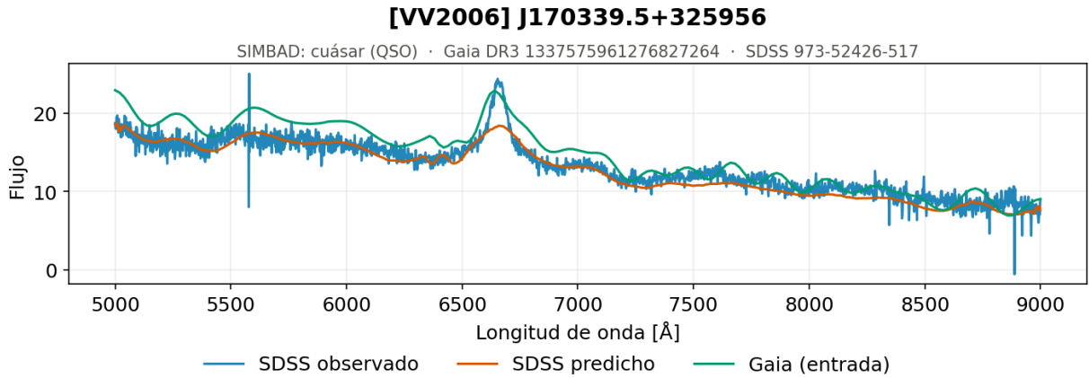
Figura 5.48. Secuencia central, alta luminosidad y alta temperatura, ejemplo 2. Espectro generado por el modelo convolucional 1D para uno de los objetos con paralaje no significativo, por debajo de 0,01 mas, cuya magnitud absoluta no es fiable: SIMBAD lo identifica como un QSO, y no como una estrella de la secuencia principal.
