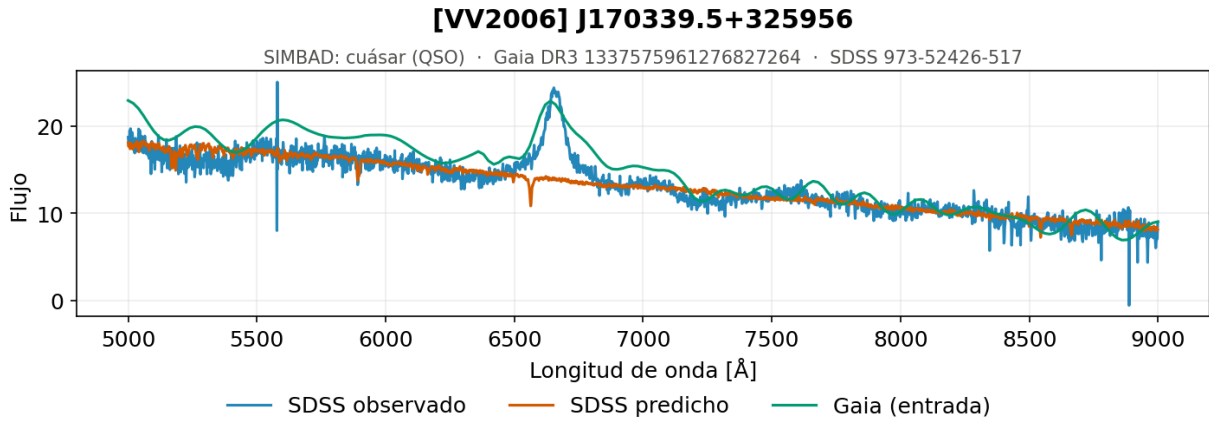
Figura 5.78. Secuencia central, alta luminosidad y alta temperatura, ejemplo 2. Espectro generado por el modelo de redes neuronales recurrentes con una capa bidireccional para uno de los objetos con paralaje no significativo, por debajo de 0,01 mas, cuya magnitud absoluta no es fiable: SIMBAD lo identifica como un QSO, y no como una estrella de la secuencia principal.
