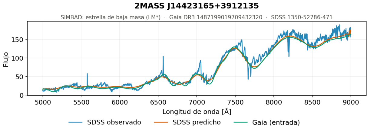
Figura 5.52. Secuencia central, baja luminosidad y baja temperatura, ejemplo 2. Espectro generado por el modelo convolucional 1D para uno de los objetos del extremo frío de la secuencia, con estrellas de baja masa de unos 3 100 K y paralajes de entre 8 y 27 mas, es decir, objetos cercanos y poco luminosos.
