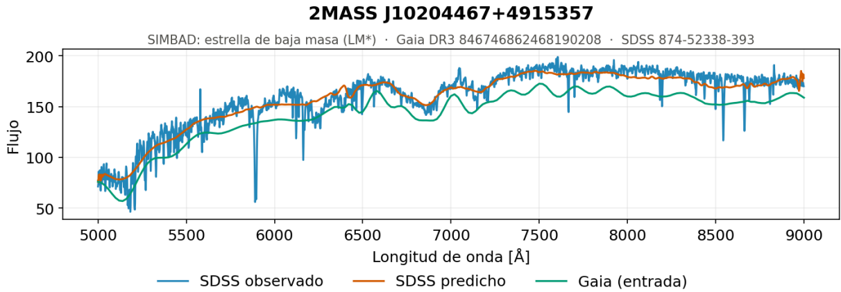
Figura 5.50. Secuencia central, ejemplo 2. Espectro generado por el modelo convolucional 1D para una de las estrellas del tramo central de la secuencia, el grupo más poblado de la muestra con 655 objetos, formado por estrellas de baja masa con temperaturas efectivas en torno a 4 500 K.
