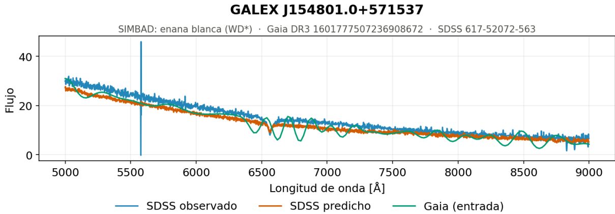
Figura 5.12. Enanas blancas, ejemplo 2. Espectro generado por el modelo de redes neuronales densas con normalización global para una de las enanas blancas, objetos calientes y poco luminosos cuyo espectro es un continuo decreciente con muy pocos rasgos.
