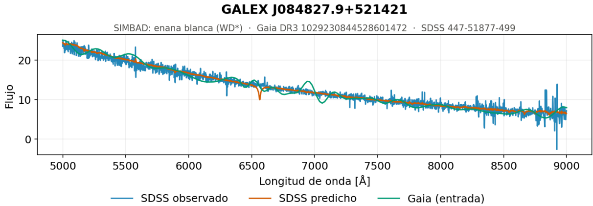
Figura 5.72. Enanas blancas, ejemplo 1. Espectro generado por el modelo de redes neuronales recurrentes con una capa de GRU para una de las enanas blancas, objetos calientes y poco luminosos cuyo espectro es un continuo decreciente con muy pocos rasgos.
