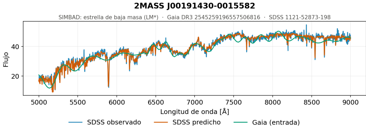
Figura 5.68. Secuencia central, ejemplo 1. Espectro generado por el modelo de redes neuronales recurrentes con una capa de GRU para una de las estrellas del tramo central de la secuencia, el grupo más poblado de la muestra con 655 objetos, formado por estrellas de baja masa con temperaturas efectivas en torno a 4 500 K.
