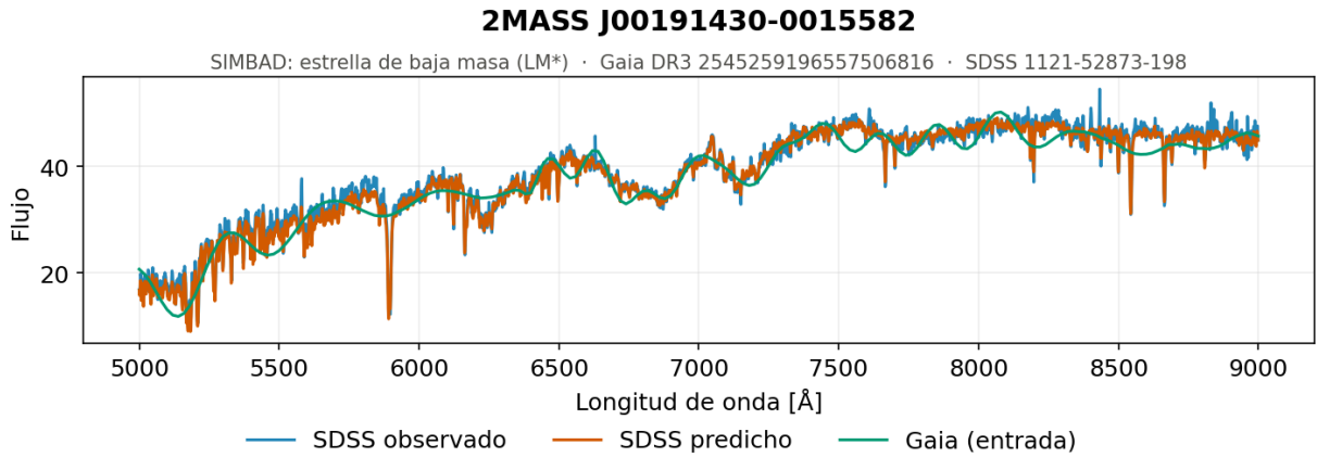
Figura 5.18. Secuencia central, ejemplo 1. Espectro generado por el modelo de redes neuronales densas con normalización basada en la mediana de cada espectro para una de las estrellas del tramo central de la secuencia, el grupo más poblado de la muestra con 655 objetos, formado por estrellas de baja masa con temperaturas efectivas en torno a 4 500 K.
