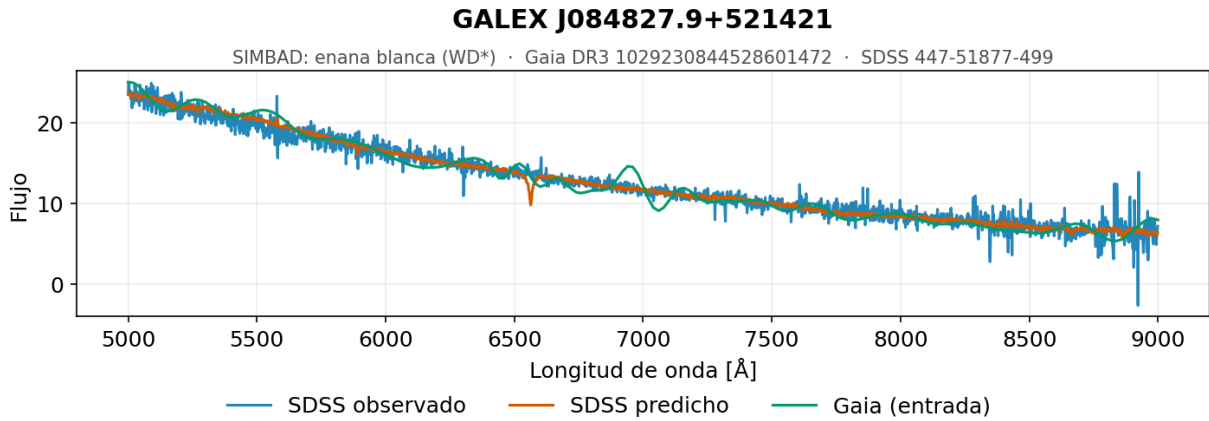
Figura 5.22. Enanas blancas, ejemplo 1. Espectro generado por el modelo de redes neuronales densas con normalización basada en la mediana de cada espectro para una de las enanas blancas, objetos calientes y poco luminosos cuyo espectro es un continuo decreciente con muy pocos rasgos.
