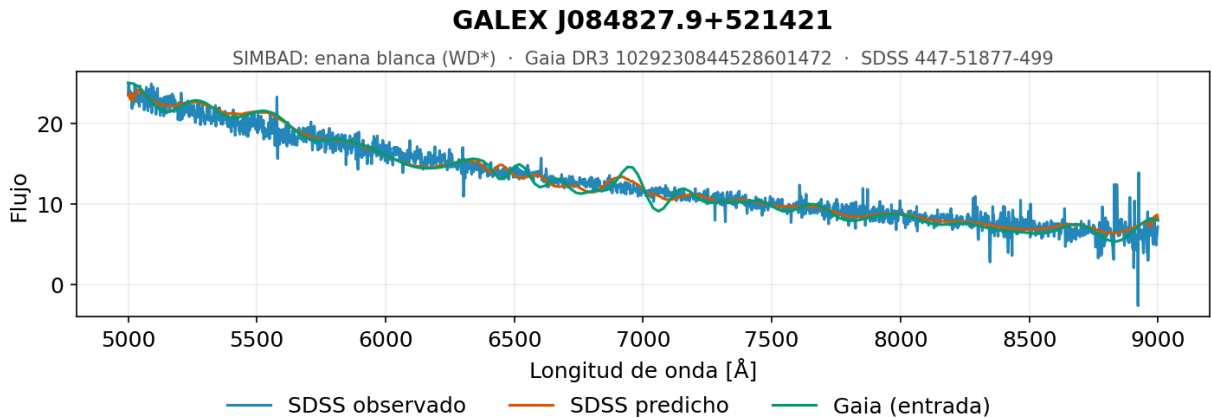
Figura 5.53. Enanas blancas, ejemplo 1. Espectro generado por el modelo convolucional 1D para una de las enanas blancas, objetos calientes y poco luminosos cuyo espectro es un continuo decreciente con muy pocos rasgos.
