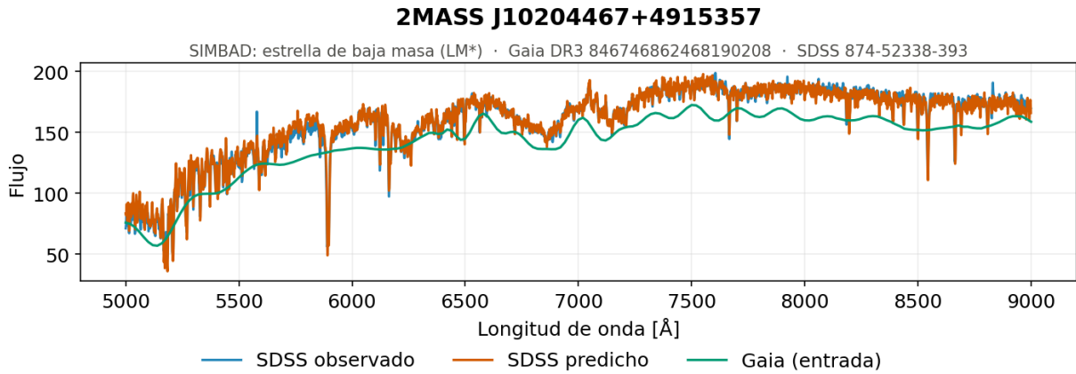
Figura 5.39. Secuencia central, ejemplo 2. Espectro generado por el modelo de redes neuronales densas con la SNR de Gaia como entrada para una de las estrellas del tramo central de la secuencia, el grupo más poblado de la muestra con 655 objetos, formado por estrellas de baja masa con temperaturas efectivas en torno a 4 500 K.
