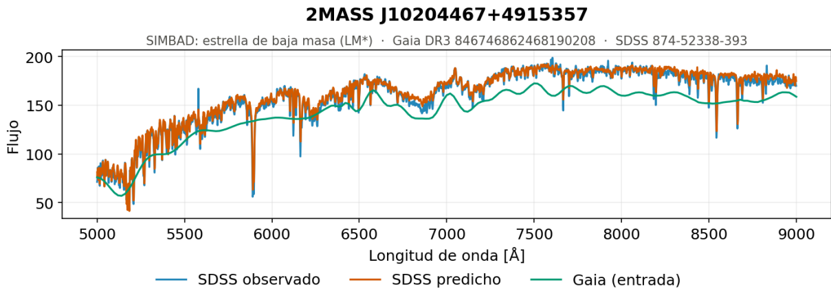
Figura 5.69. Secuencia central, ejemplo 2. Espectro generado por el modelo de redes neuronales recurrentes con una capa de GRU para una de las estrellas del tramo central de la secuencia, el grupo más poblado de la muestra con 655 objetos, formado por estrellas de baja masa con temperaturas efectivas en torno a 4 500 K.
