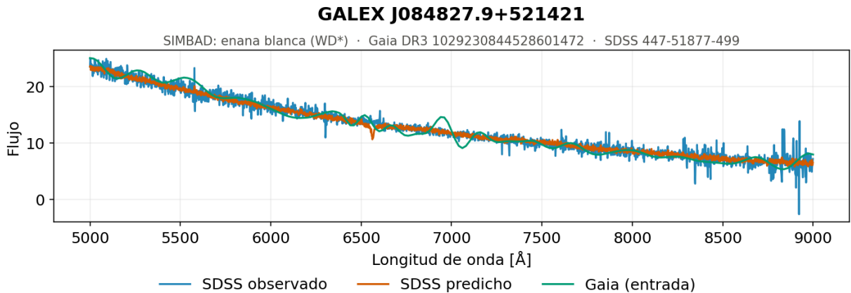
Figura 5.11. Enanas blancas, ejemplo 1. Espectro generado por el modelo de redes neuronales densas con normalización global para una de las enanas blancas, objetos calientes y poco luminosos cuyo espectro es un continuo decreciente con muy pocos rasgos.
