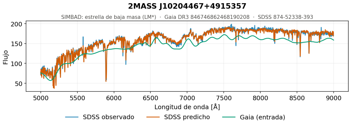
Figura 5.19. Secuencia central, ejemplo 2. Espectro generado por el modelo de redes neuronales densas con normalización basada en la mediana de cada espectro para una de las estrellas del tramo central de la secuencia, el grupo más poblado de la muestra con 655 objetos, formado por estrellas de baja masa con temperaturas efectivas en torno a 4 500 K.
