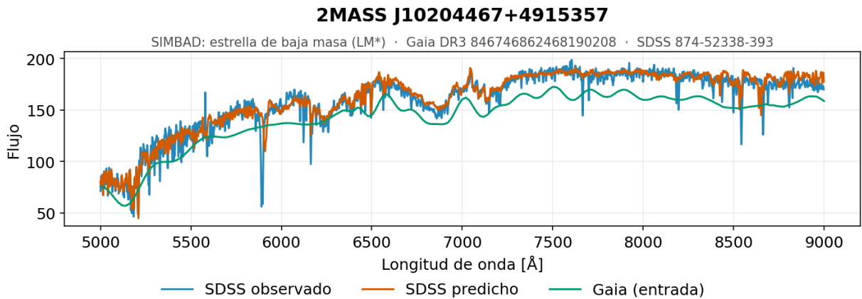
Figura 5.61. Secuencia central, ejemplo 2. Espectro generado por el modelo convolucional U-Net para una de las estrellas del tramo central de la secuencia, el grupo más poblado de la muestra con 655 objetos, formado por estrellas de baja masa con temperaturas efectivas en torno a 4 500 K.
