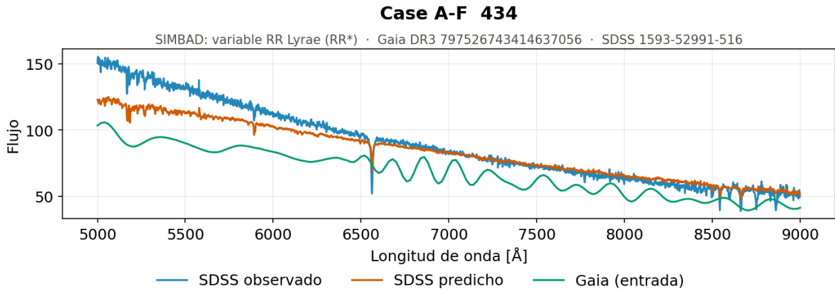
Figura 5.66. Secuencia central, alta luminosidad y alta temperatura, ejemplo 1. Espectro generado por el modelo de redes neuronales recurrentes con una capa de GRU para uno de los objetos con paralaje no significativo, por debajo de 0,01 mas, cuya magnitud absoluta no es fiable: SIMBAD lo identifica como una RR*, y no como una estrella de la secuencia principal.
