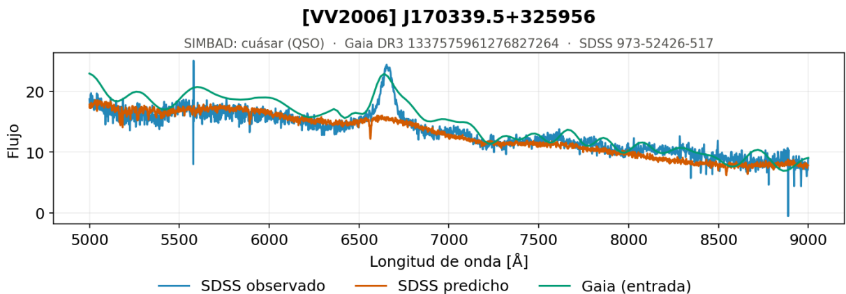
Figura 5.17. Secuencia central, alta luminosidad y alta temperatura, ejemplo 2. Espectro generado por el modelo de redes neuronales densas con normalización basada en la mediana de cada espectro para uno de los objetos con paralaje no significativo, por debajo de 0,01 mas, cuya magnitud absoluta no es fiable: SIMBAD lo identifica como un QSO, y no como una estrella de la secuencia principal.
