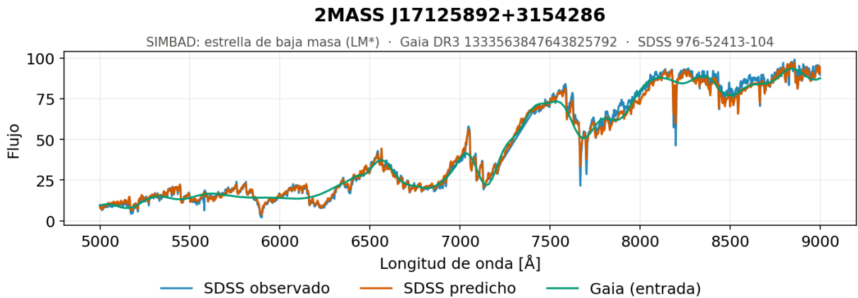
Figura 5.81. Secuencia central, baja luminosidad y baja temperatura, ejemplo 1. Espectro generado por el modelo de redes neuronales recurrentes con una capa bidireccional para uno de los objetos del extremo frío de la secuencia, con estrellas de baja masa de unos 3 100 K y paralajes de entre 8 y 27 mas, es decir, objetos cercanos y poco luminosos.
