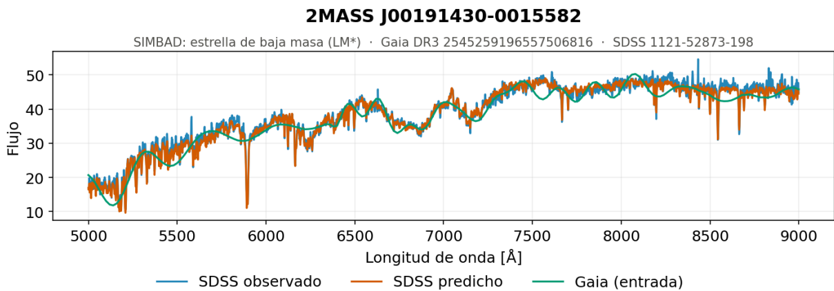
Figura 5.38. Secuencia central, ejemplo 1. Espectro generado por el modelo de redes neuronales densas con la SNR de Gaia como entrada para una de las estrellas del tramo central de la secuencia, el grupo más poblado de la muestra con 655 objetos, formado por estrellas de baja masa con temperaturas efectivas en torno a 4 500 K.
