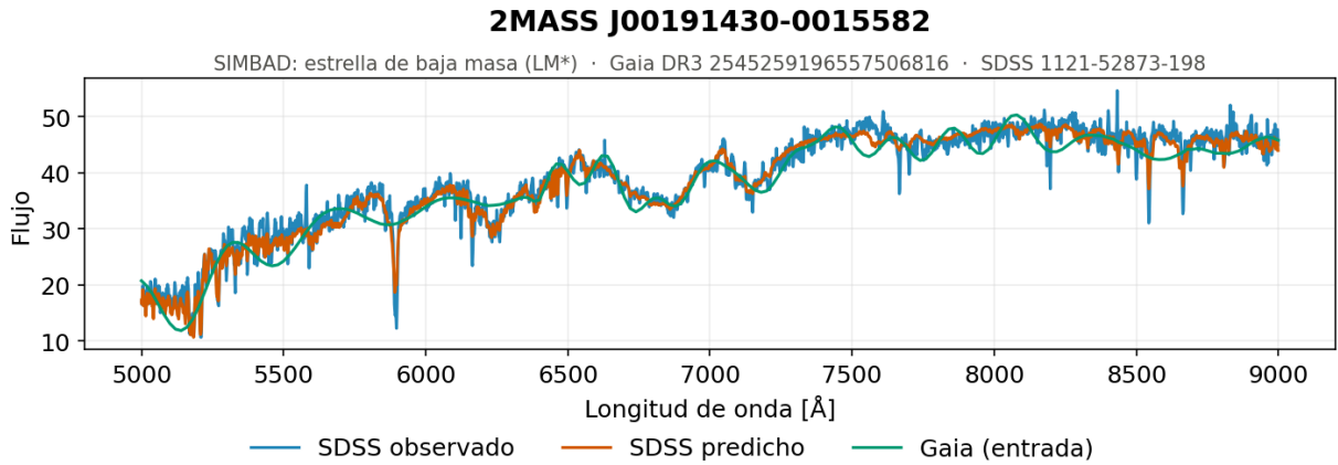
Figura 5.60. Secuencia central, ejemplo 1. Espectro generado por el modelo convolucional U-Net para una de las estrellas del tramo central de la secuencia, el grupo más poblado de la muestra con 655 objetos, formado por estrellas de baja masa con temperaturas efectivas en torno a 4 500 K.
