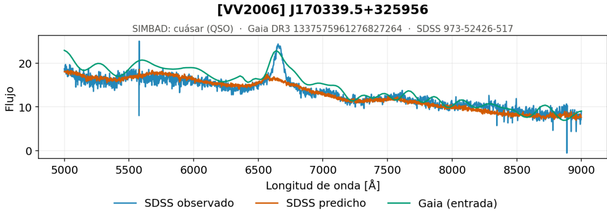
Figura 5.37. Secuencia central, alta luminosidad y alta temperatura, ejemplo 2. Espectro generado por el modelo de redes neuronales densas con la SNR de Gaia como entrada para uno de los objetos con paralaje no significativo, por debajo de 0,01 mas, cuya magnitud absoluta no es fiable: SIMBAD lo identifica como un QSO, y no como una estrella de la secuencia principal.
