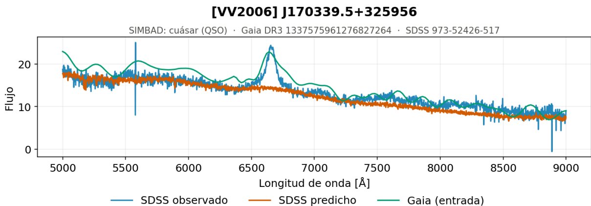
Figura 5.25. Secuencia central, alta luminosidad y alta temperatura, ejemplo 2. Espectro generado por el modelo de redes neuronales densas con normalización basada en el máximo de cada espectro para uno de los objetos con paralaje no significativo, por debajo de 0,01 mas, cuya magnitud absoluta no es fiable: SIMBAD lo identifica como un QSO, y no como una estrella de la secuencia principal.
