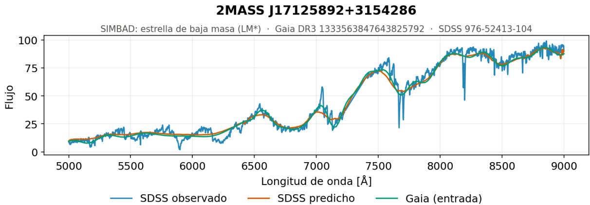
Figura 5.51. Secuencia central, baja luminosidad y baja temperatura, ejemplo 1. Espectro generado por el modelo convolucional 1D para uno de los objetos del extremo frío de la secuencia, con estrellas de baja masa de unos 3 100 K y paralajes de entre 8 y 27 mas, es decir, objetos cercanos y poco luminosos.
