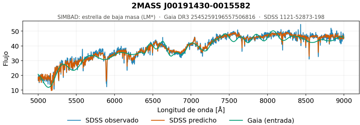
Figura 5.90. Secuencia central, ejemplo 1. Espectro generado por el modelo de redes neuronales recurrentes con una función de Atención para una de las estrellas del tramo central de la secuencia, el grupo más poblado de la muestra con 655 objetos, formado por estrellas de baja masa con temperaturas efectivas en torno a 4 500 K.
