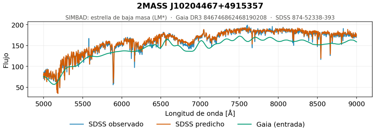
Figura 5.80. Secuencia central, ejemplo 2. Espectro generado por el modelo de redes neuronales recurrentes con una capa bidireccional para una de las estrellas del tramo central de la secuencia, el grupo más poblado de la muestra con 655 objetos, formado por estrellas de baja masa con temperaturas efectivas en torno a 4 500 K.
