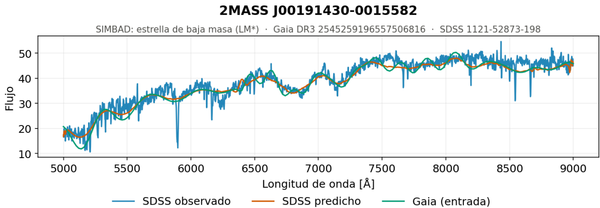
Figura 5.49. Secuencia central, ejemplo 1. Espectro generado por el modelo convolucional 1D para una de las estrellas del tramo central de la secuencia, el grupo más poblado de la muestra con 655 objetos, formado por estrellas de baja masa con temperaturas efectivas en torno a 4 500 K.
