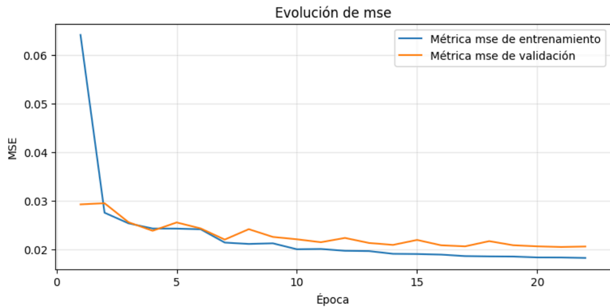
Figura 5.3. Evolución del MSE durante el entrenamiento
