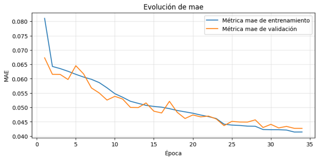
Figura 5.56. Evolución del MAE durante el entrenamiento del modelo convolucional U-Net
