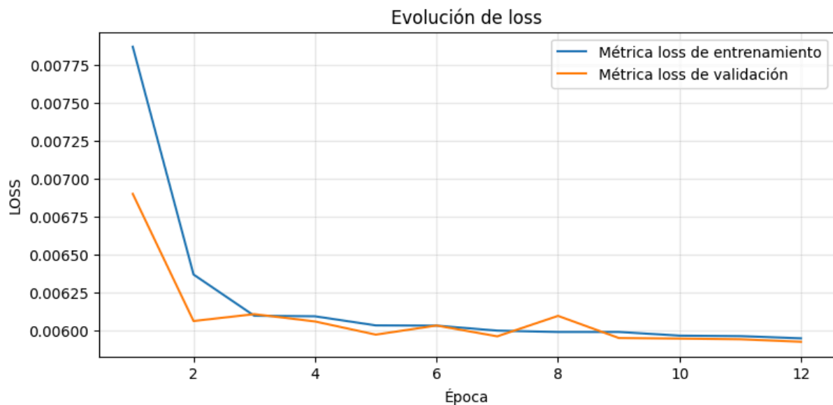
Figura 5.44. Evolución de la pérdida durante el entrenamiento del modelo convolucional 1D
