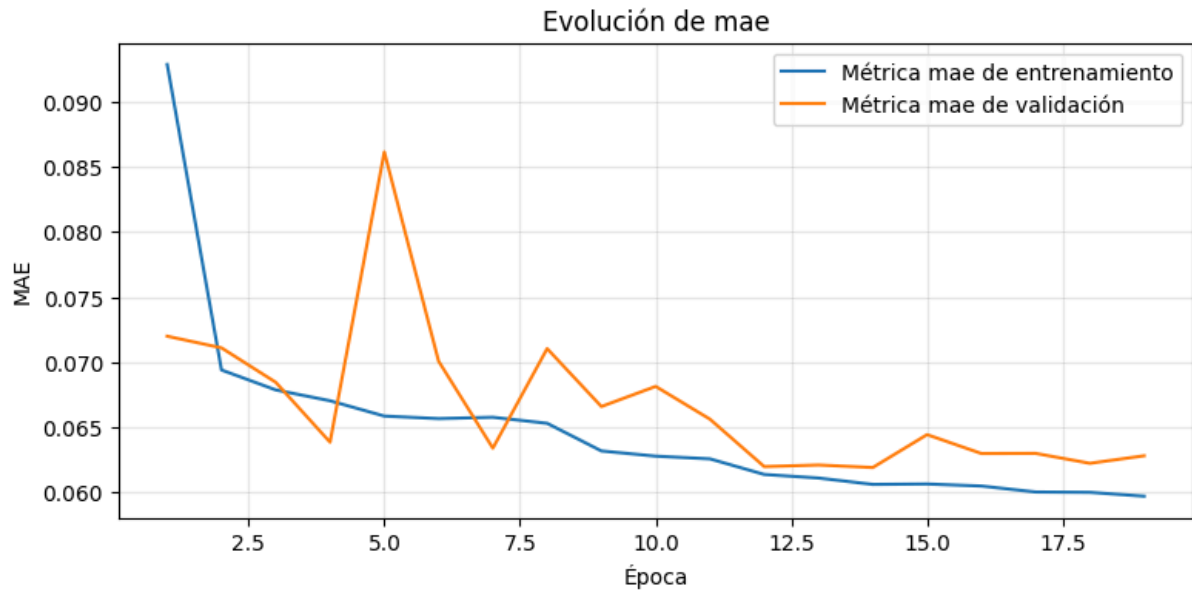
Figura 5.34. Evolución del MAE durante el entrenamiento de la red densa con normalización basada en el máximo de cada espectro
