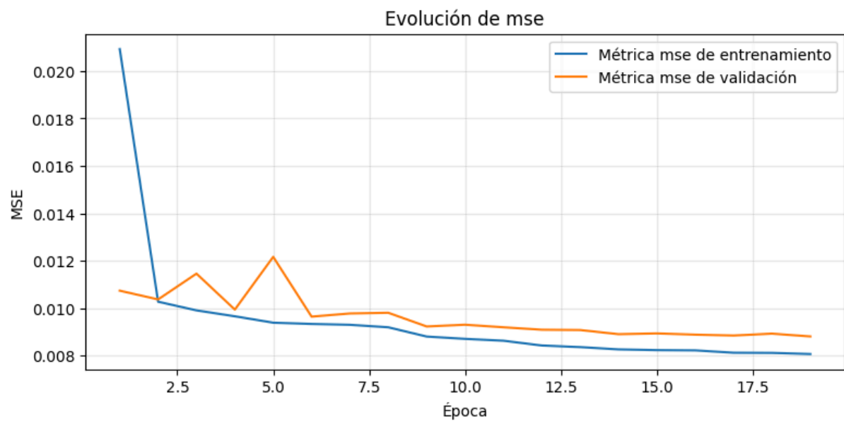
Figura 5.33. Evolución del MSE durante el entrenamiento de la red densa con normalización basada en el máximo de cada espectro
