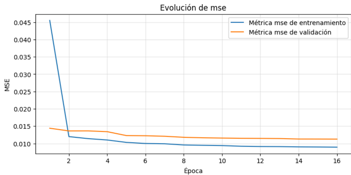
Figura 5.14. Evolución del MSE durante el entrenamiento de la red densa con normalización basada en la mediana
