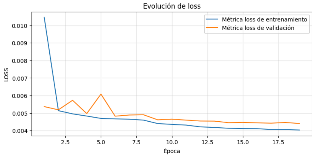
Figura 5.32. Evolución de la pérdida durante el entrenamiento de la red densa con normalización basada en el máximo de cada espectro
