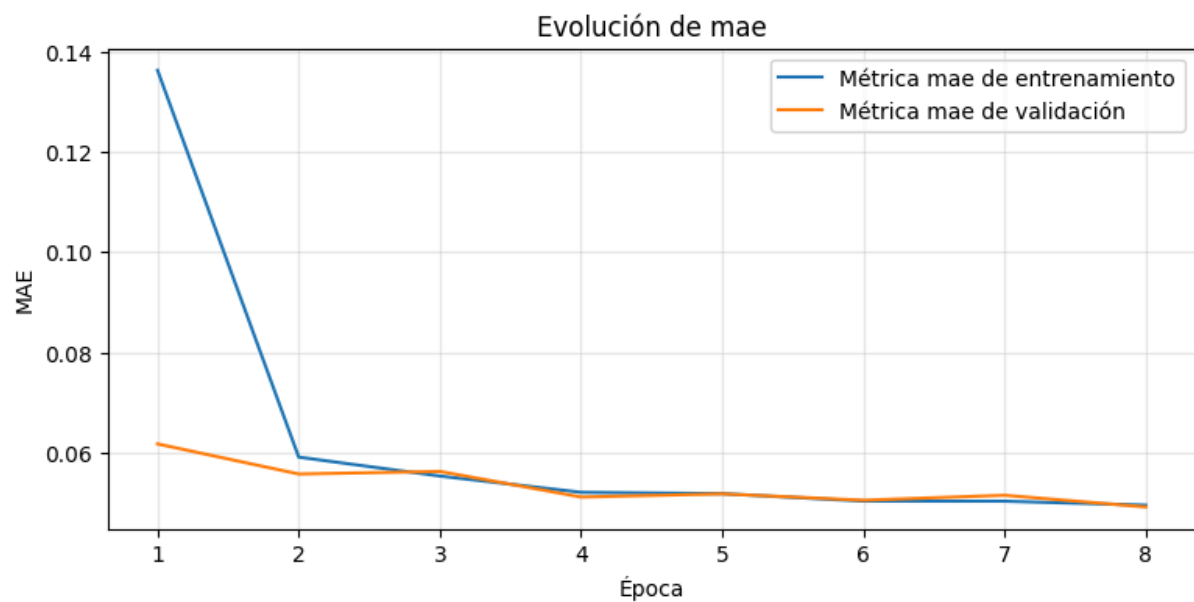
Figura 5.86. Evolución del MAE durante el entrenamiento del modelo basado en una capa Bidireccional
