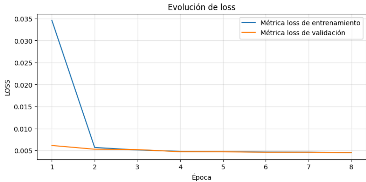
Figura 5.85. Evolución de la pérdida durante el entrenamiento del modelo basado en una capa Bidireccional
