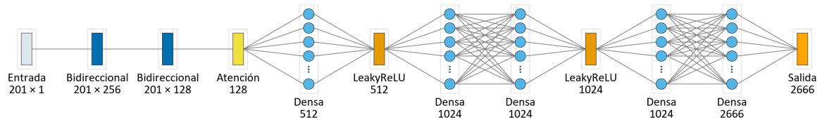
Figura 4.14. Arquitectura del modelo recurrente bidireccional con atención
