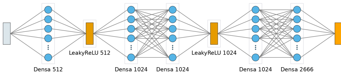
Figura 4.9. Arquitectura del modelo denso
