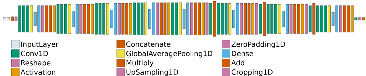
Figura 4.11. Arquitectura del modelo convolucional U-Net
