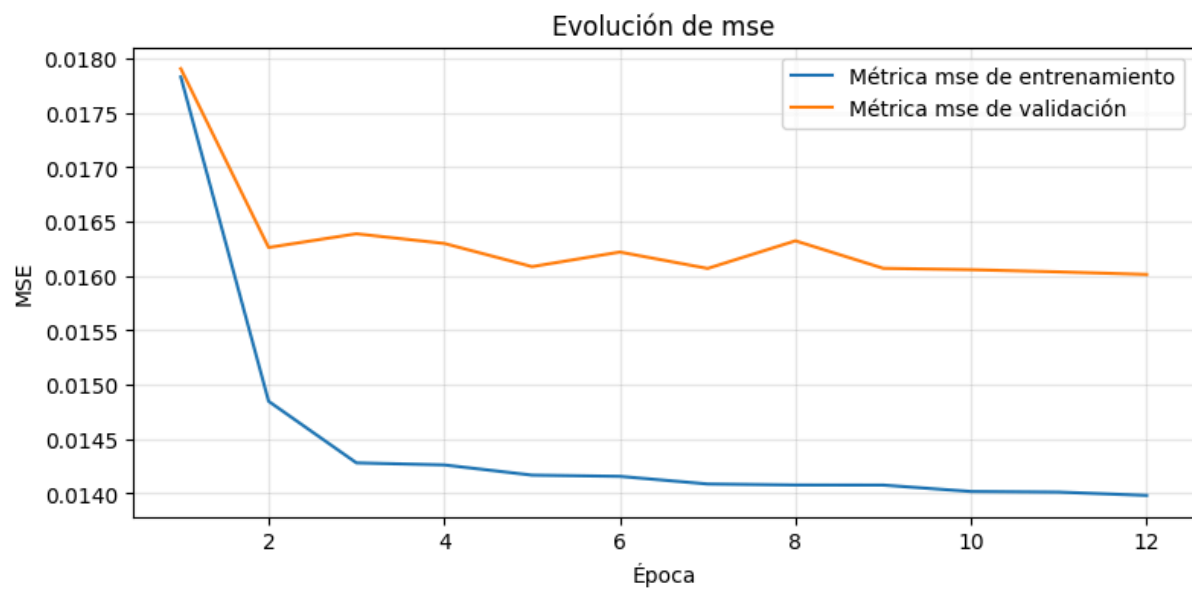
Figura 5.46. Evolución del MSE durante el entrenamiento del modelo convolucional 1D
