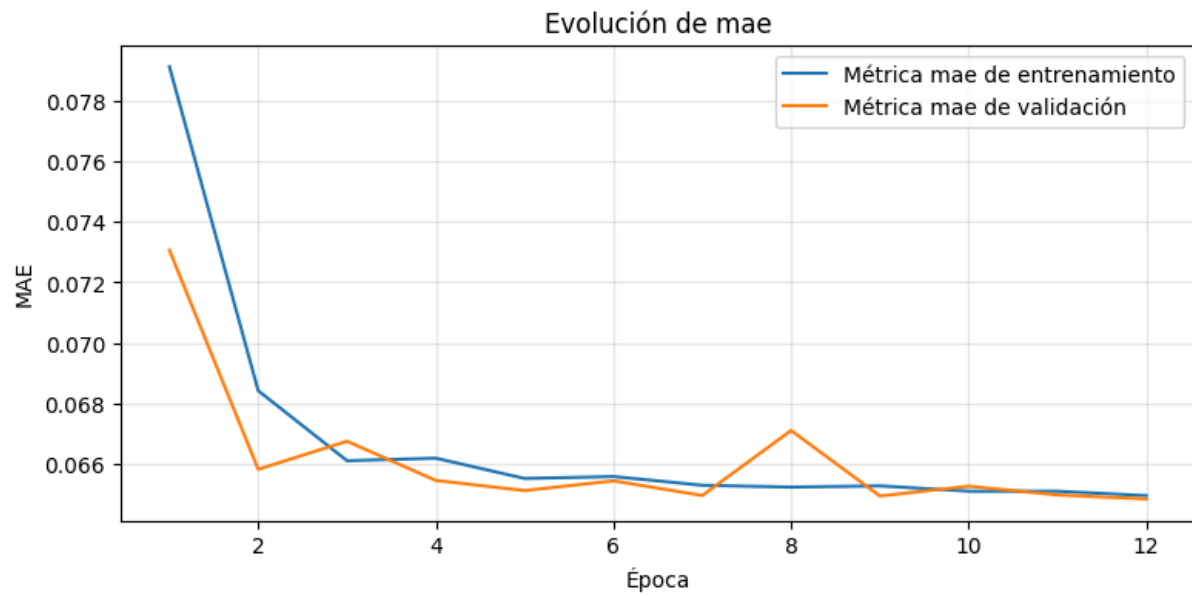
Figura 5.45. Evolución del MAE durante el entrenamiento del modelo convolucional 1D
