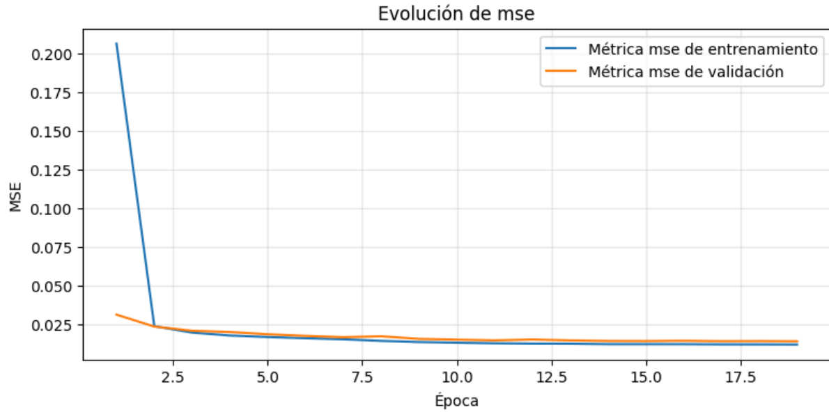
Figura 5.76. Evolución del MSE durante el entrenamiento del modelo basado en una capa GRU
