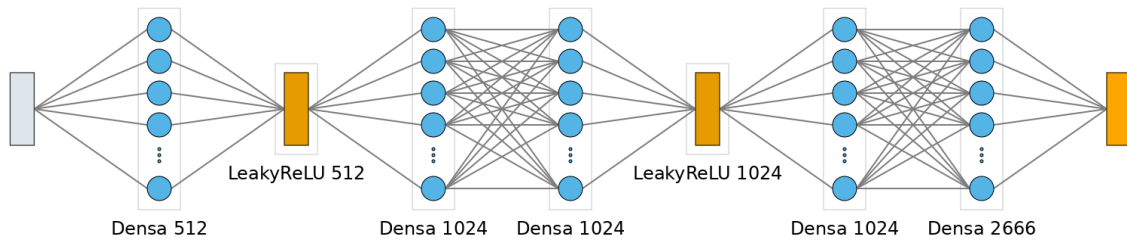
Figura 5.35. Arquitectura del modelo denso con la SNR
