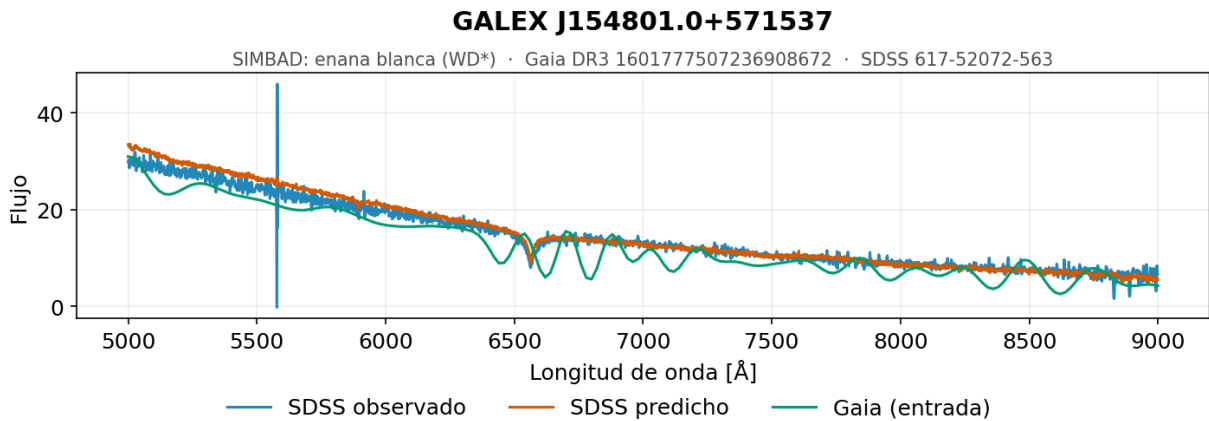
Figura 5.23. Enanas blancas, ejemplo 2. Espectro generado por el modelo de redes neuronales densas con normalización basada en la mediana de cada espectro para una de las enanas blancas, objetos calientes y poco luminosos cuyo espectro es un continuo decreciente con muy pocos rasgos.
