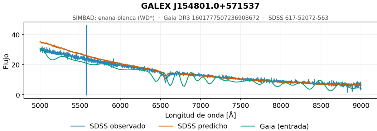
Figura 5.84. Enanas blancas, ejemplo 2. Espectro generado por el modelo de redes neuronales recurrentes con una capa bidireccional para una de las enanas blancas, objetos calientes y poco luminosos cuyo espectro es un continuo decreciente con muy pocos rasgos.
