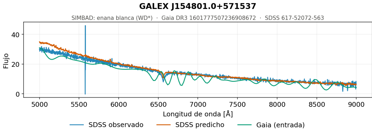
Figura 5.95. Enanas blancas, ejemplo 2. Espectro generado por el modelo de redes neuronales recurrentes con una función de Atención para una de las enanas blancas, objetos calientes y poco luminosos cuyo espectro es un continuo decreciente con muy pocos rasgos.
