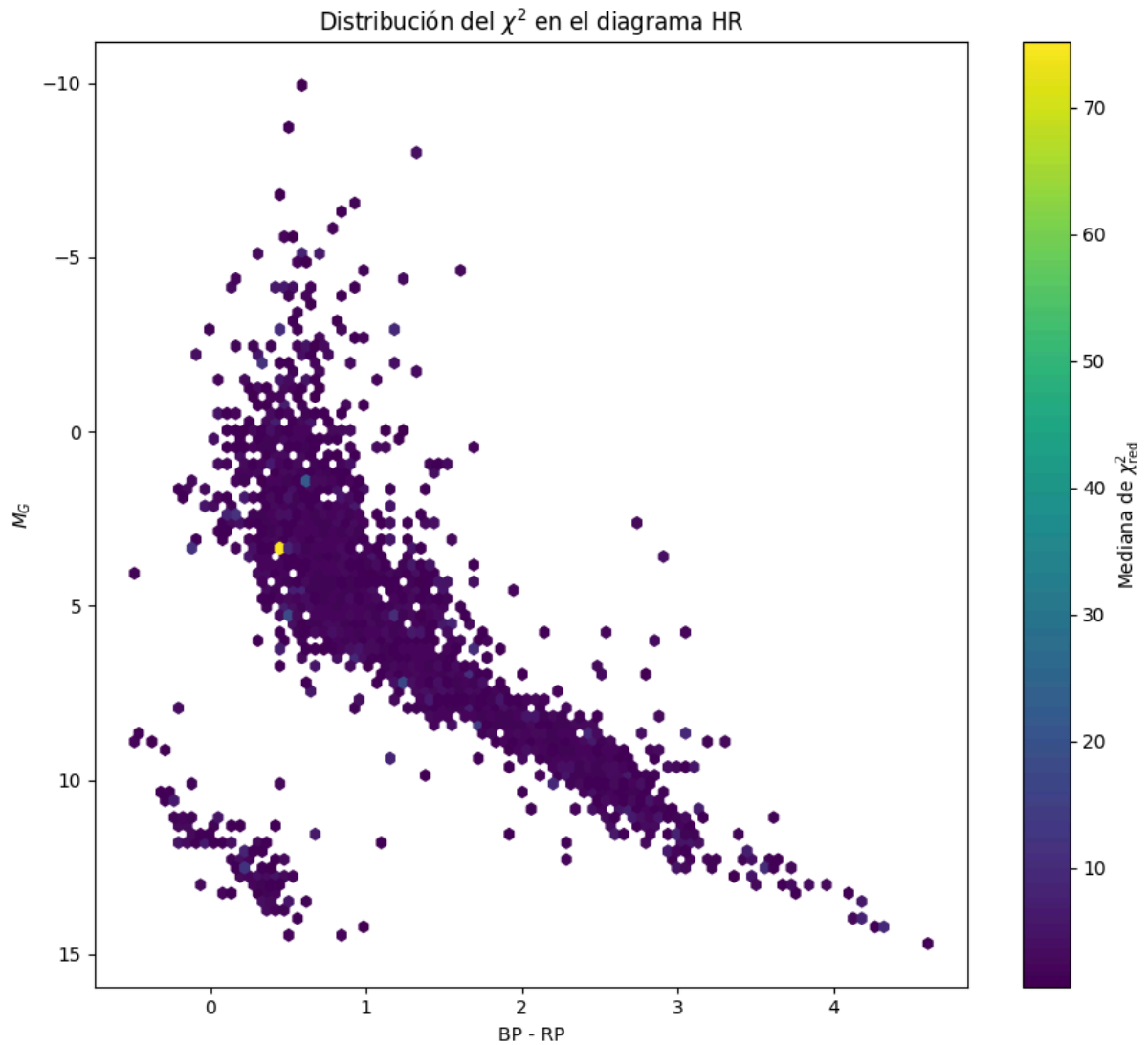
Figura 6.2. Diagrama HR del estadístico \chi^2 normalizado aplicado sobre la muestra de test en el modelo convolucional U-Net.
