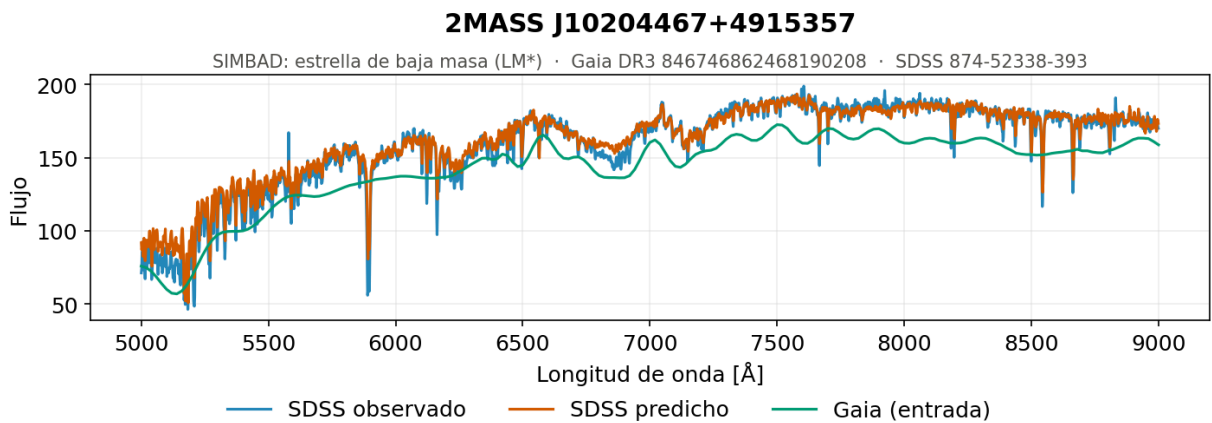
Figura 5.91. Secuencia central, ejemplo 2. Espectro generado por el modelo de redes neuronales recurrentes con una función de Atención para una de las estrellas del tramo central de la secuencia, el grupo más poblado de la muestra con 655 objetos, formado por estrellas de baja masa con temperaturas efectivas en torno a 4 500 K.
