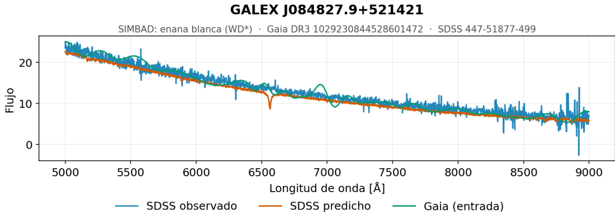
Figura 5.30. Enanas blancas, ejemplo 1. Espectro generado por el modelo de redes neuronales densas con normalización basada en el máximo de cada espectro para una de las enanas blancas, objetos calientes y poco luminosos cuyo espectro es un continuo decreciente con muy pocos rasgos.
