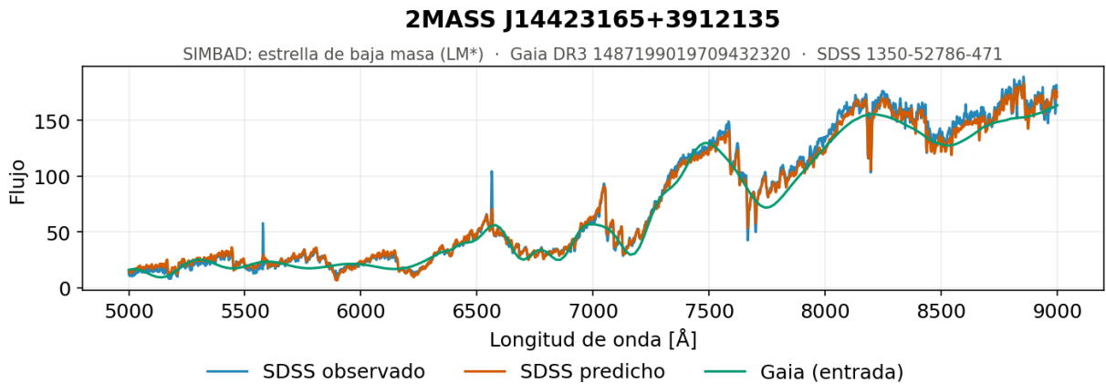
Figura 5.93. Secuencia central, baja luminosidad y baja temperatura, ejemplo 2. Espectro generado por el modelo de redes neuronales recurrentes con una función de Atención para uno de los objetos del extremo frío de la secuencia, con estrellas de baja masa de unos 3 100 K y paralajes de entre 8 y 27 mas, es decir, objetos cercanos y poco luminosos.
