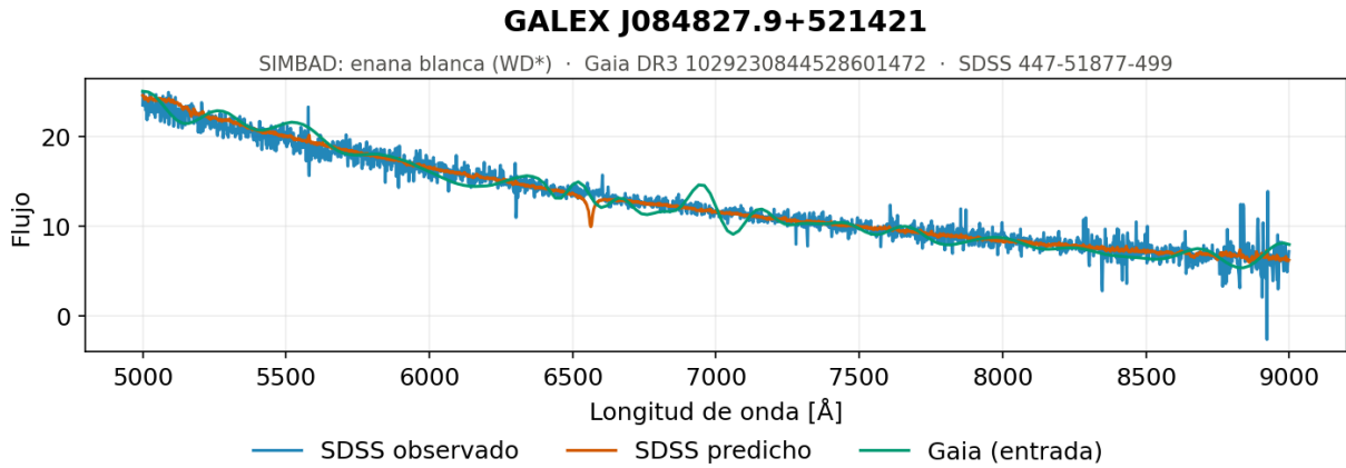
Figura 5.94. Enanas blancas, ejemplo 1. Espectro generado por el modelo de redes neuronales recurrentes con una función de Atención para una de las enanas blancas, objetos calientes y poco luminosos cuyo espectro es un continuo decreciente con muy pocos rasgos.
