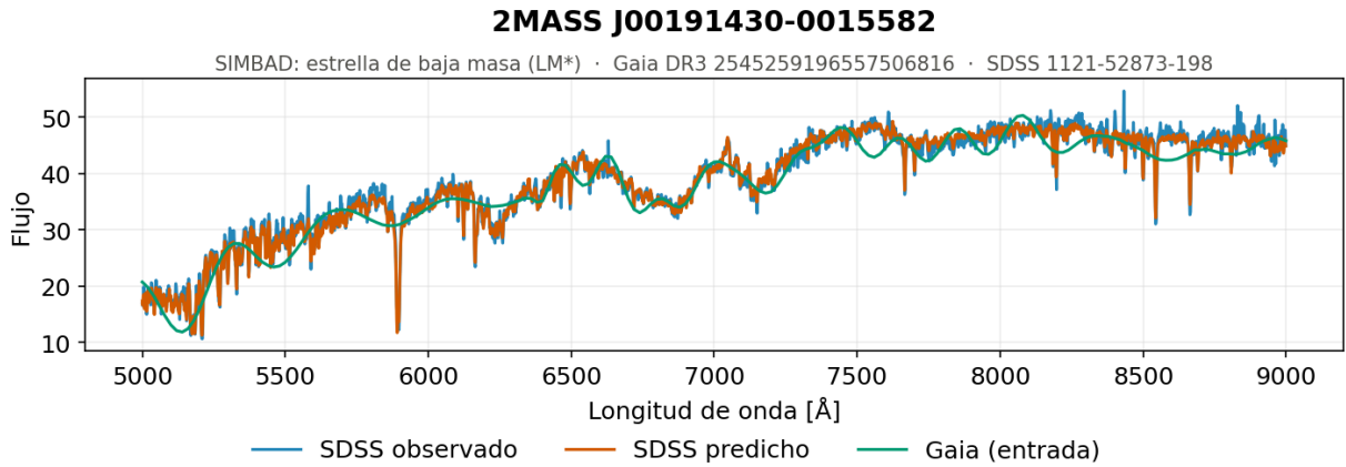
Figura 5.26. Secuencia central, ejemplo 1. Espectro generado por el modelo de redes neuronales densas con normalización basada en el máximo de cada espectro para una de las estrellas del tramo central de la secuencia, el grupo más poblado de la muestra con 655 objetos, formado por estrellas de baja masa con temperaturas efectivas en torno a 4 500 K.
