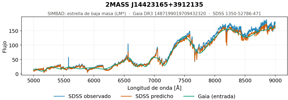
Figura 5.10. Secuencia central, baja luminosidad y baja temperatura, ejemplo 2. Espectro generado por el modelo de redes neuronales densas con normalización global para uno de los objetos del extremo frío de la secuencia, con estrellas de baja masa de unos 3 100 K y paralajes de entre 8 y 27 mas, es decir, objetos cercanos y poco luminosos.
