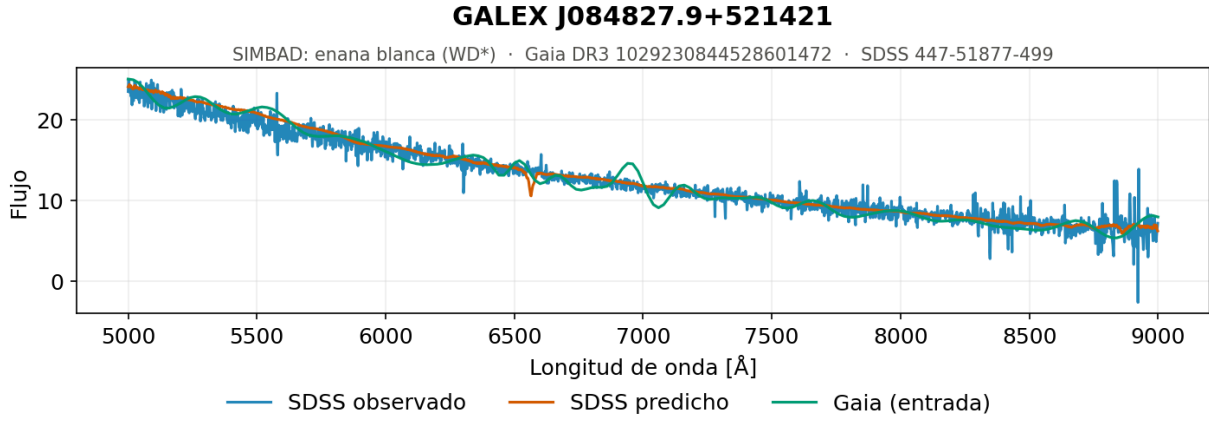
Figura 5.64. Enanas blancas, ejemplo 1. Espectro generado por el modelo convolucional U-Net para una de las enanas blancas, objetos calientes y poco luminosos cuyo espectro es un continuo decreciente con muy pocos rasgos.
