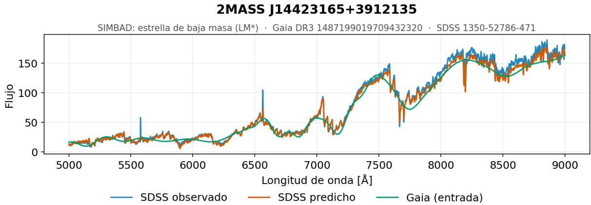
Figura 5.82. Secuencia central, baja luminosidad y baja temperatura, ejemplo 2. Espectro generado por el modelo de redes neuronales recurrentes con una capa bidireccional para uno de los objetos del extremo frío de la secuencia, con estrellas de baja masa de unos 3 100 K y paralajes de entre 8 y 27 mas, es decir, objetos cercanos y poco luminosos.
