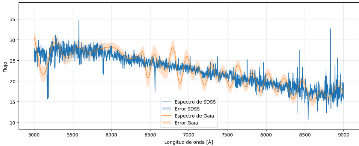
Figura 4.8. Ejemplo 2 de espectro observado por Gaia y SDSS con bandas de error
