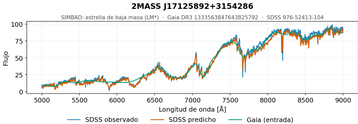
Figura 5.28. Secuencia central, baja luminosidad y baja temperatura, ejemplo 1. Espectro generado por el modelo de redes neuronales densas con normalización basada en el máximo de cada espectro para uno de los objetos del extremo frío de la secuencia, con estrellas de baja masa de unos 3 100 K y paralajes de entre 8 y 27 mas, es decir, objetos cercanos y poco luminosos.
