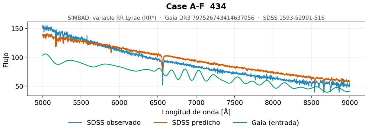
Figura 5.24. Secuencia central, alta luminosidad y alta temperatura, ejemplo 1. Espectro generado por el modelo de redes neuronales densas con normalización basada en el máximo de cada espectro para uno de los objetos con paralaje no significativo, por debajo de 0,01 mas, cuya magnitud absoluta no es fiable: SIMBAD lo identifica como una RR*, y no como una estrella de la secuencia principal.
