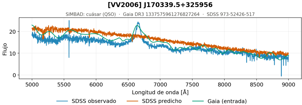
Figura 5.6. Secuencia central, alta luminosidad y alta temperatura, ejemplo 2. Espectro generado por el modelo de redes neuronales densas con normalización global para uno de los objetos con paralaje no significativo, por debajo de 0,01 mas, cuya magnitud absoluta no es fiable: SIMBAD lo identifica como un QSO, y no como una estrella de la secuencia principal.
