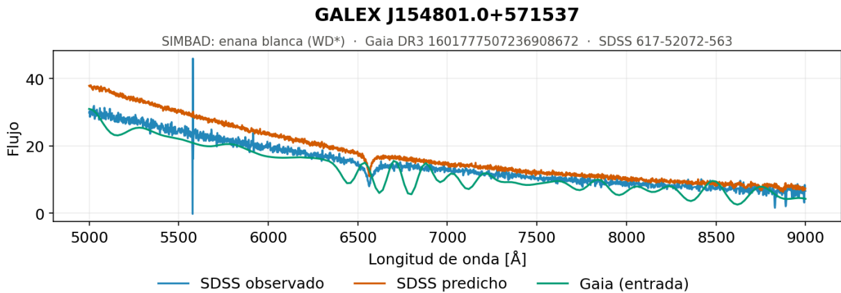
Figura 5.31. Enanas blancas, ejemplo 2. Espectro generado por el modelo de redes neuronales densas con normalización basada en el máximo de cada espectro para una de las enanas blancas, objetos calientes y poco luminosos cuyo espectro es un continuo decreciente con muy pocos rasgos.
