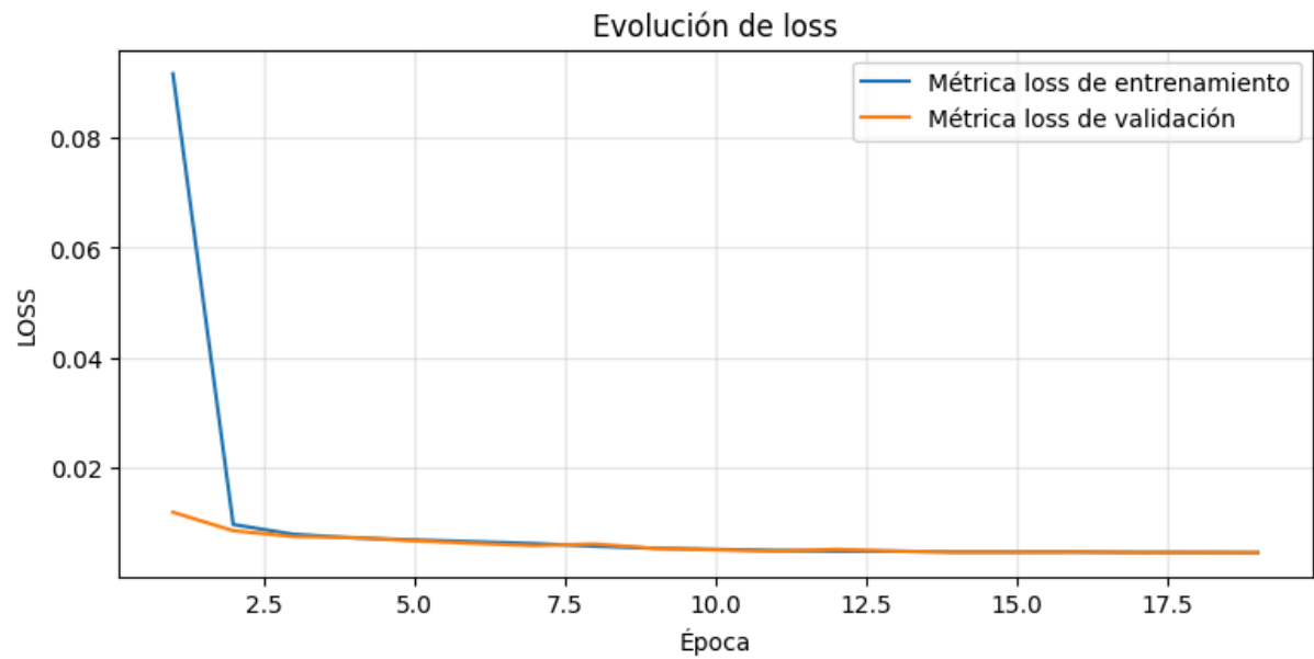
Figura 5.74. Evolución de la pérdida durante el entrenamiento del modelo basado en una capa GRU
