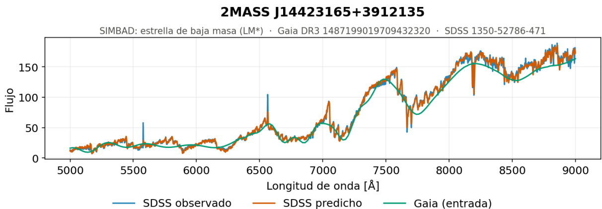
Figura 5.21. Secuencia central, baja luminosidad y baja temperatura, ejemplo 2. Espectro generado por el modelo de redes neuronales densas con normalización basada en la mediana de cada espectro para uno de los objetos del extremo frío de la secuencia, con estrellas de baja masa de unos 3 100 K y paralajes de entre 8 y 27 mas, es decir, objetos cercanos y poco luminosos.
