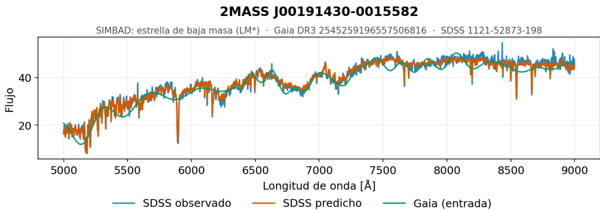
Figura 5.79. Secuencia central, ejemplo 1. Espectro generado por el modelo de redes neuronales recurrentes con una capa bidireccional para una de las estrellas del tramo central de la secuencia, el grupo más poblado de la muestra con 655 objetos, formado por estrellas de baja masa con temperaturas efectivas en torno a 4 500 K.
