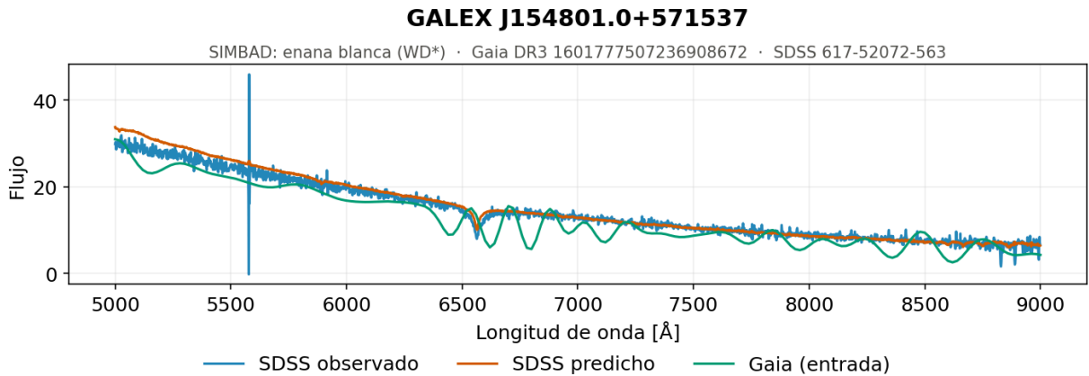
Figura 5.73. Enanas blancas, ejemplo 2. Espectro generado por el modelo de redes neuronales recurrentes con una capa de GRU para una de las enanas blancas, objetos calientes y poco luminosos cuyo espectro es un continuo decreciente con muy pocos rasgos.
