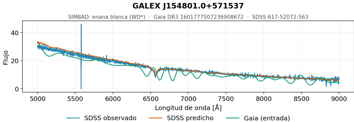
Figura 5.65. Enanas blancas, ejemplo 2. Espectro generado por el modelo convolucional U-Net para una de las enanas blancas, objetos calientes y poco luminosos cuyo espectro es un continuo decreciente con muy pocos rasgos.
