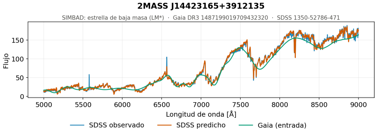
Figura 5.41. Secuencia central, baja luminosidad y baja temperatura, ejemplo 2. Espectro generado por el modelo de redes neuronales densas con la SNR de Gaia como entrada para uno de los objetos del extremo frío de la secuencia, con estrellas de baja masa de unos 3 100 K y paralajes de entre 8 y 27 mas, es decir, objetos cercanos y poco luminosos.
