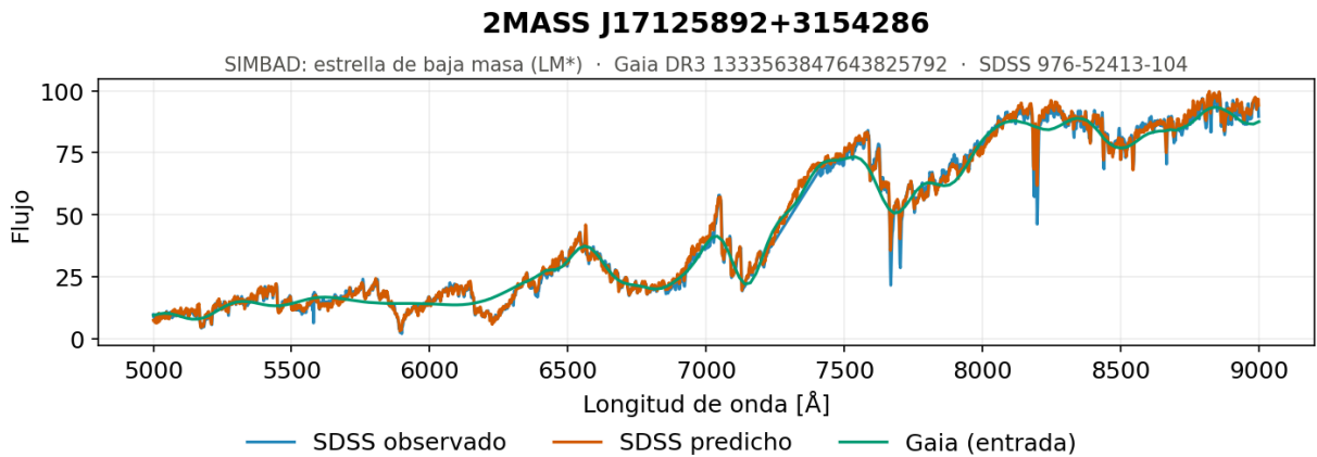
Figura 5.9. Secuencia central, baja luminosidad y baja temperatura, ejemplo 1. Espectro generado por el modelo de redes neuronales densas con normalización global para uno de los objetos del extremo frío de la secuencia, con estrellas de baja masa de unos 3 100 K y paralajes de entre 8 y 27 mas, es decir, objetos cercanos y poco luminosos.
