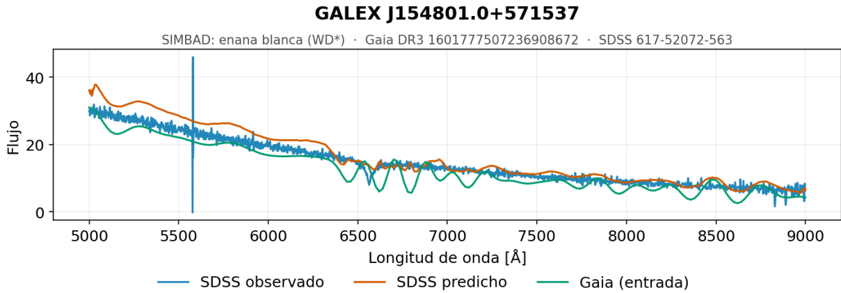
Figura 5.54. Enanas blancas, ejemplo 2. Espectro generado por el modelo convolucional 1D para una de las enanas blancas, objetos calientes y poco luminosos cuyo espectro es un continuo decreciente con muy pocos rasgos.
