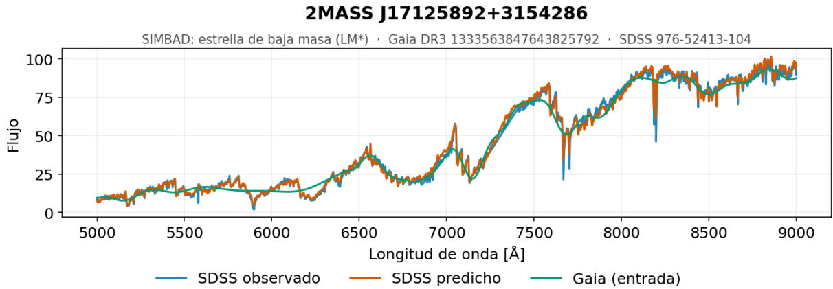
Figura 5.70. Secuencia central, baja luminosidad y baja temperatura, ejemplo 1. Espectro generado por el modelo de redes neuronales recurrentes con una capa de GRU para uno de los objetos del extremo frío de la secuencia, con estrellas de baja masa de unos 3 100 K y paralajes de entre 8 y 27 mas, es decir, objetos cercanos y poco luminosos.
