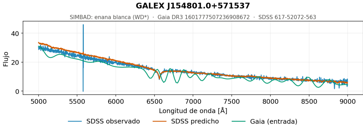
Figura 5.43. Enanas blancas, ejemplo 2. Espectro generado por el modelo de redes neuronales densas con la SNR de Gaia como entrada para una de las enanas blancas, objetos calientes y poco luminosos cuyo espectro es un continuo decreciente con muy pocos rasgos.
