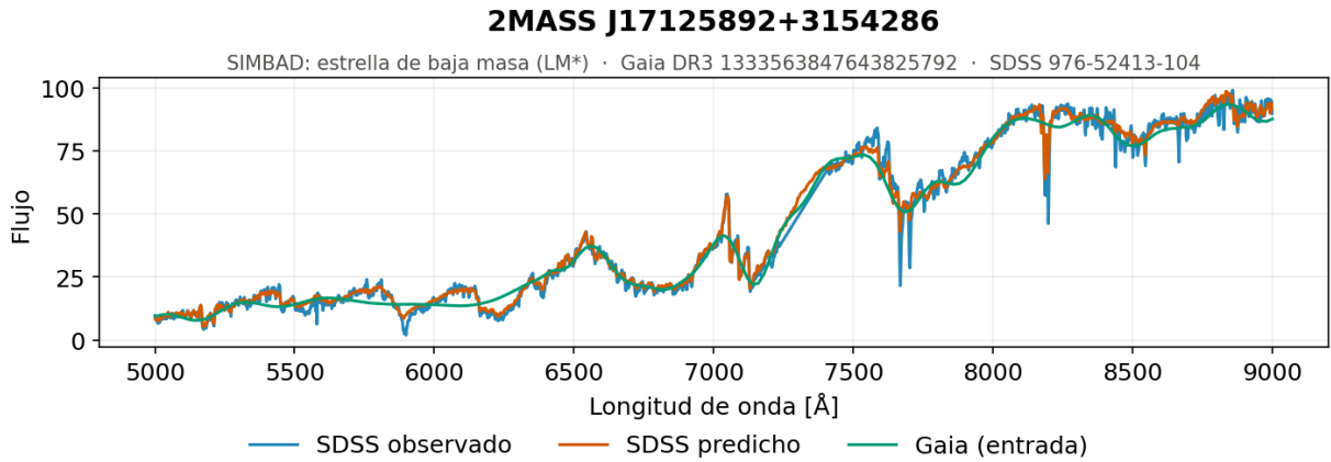
Figura 5.62. Secuencia central, baja luminosidad y baja temperatura, ejemplo 1. Espectro generado por el modelo convolucional U-Net para uno de los objetos del extremo frío de la secuencia, con estrellas de baja masa de unos 3 100 K y paralajes de entre 8 y 27 mas, es decir, objetos cercanos y poco luminosos.
