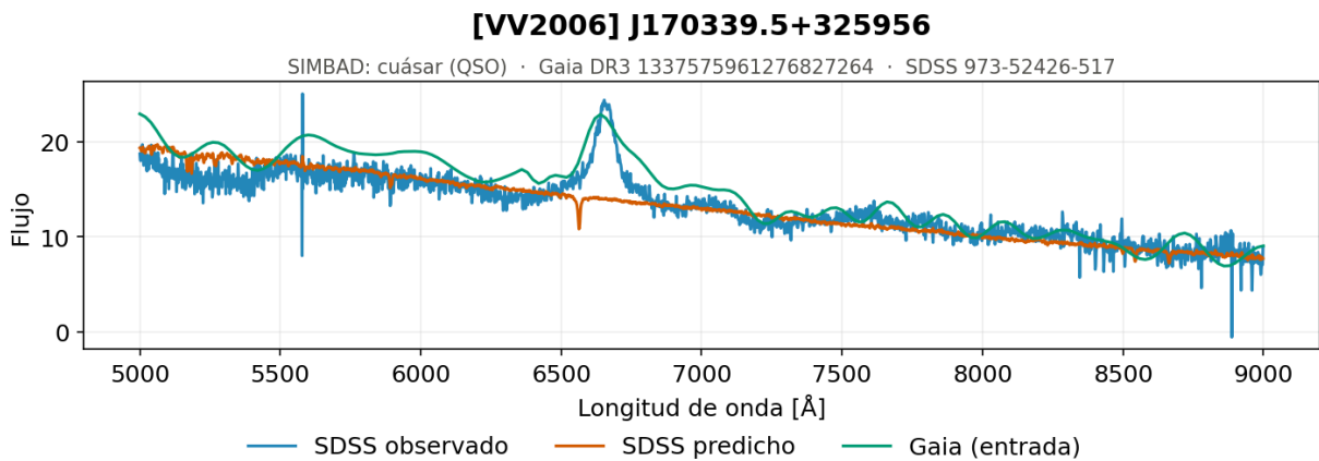
Figura 5.67. Secuencia central, alta luminosidad y alta temperatura, ejemplo 2. Espectro generado por el modelo de redes neuronales recurrentes con una capa de GRU para uno de los objetos con paralaje no significativo, por debajo de 0,01 mas, cuya magnitud absoluta no es fiable: SIMBAD lo identifica como un QSO, y no como una estrella de la secuencia principal.
