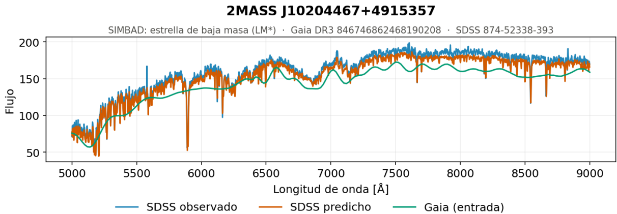
Figura 5.27. Secuencia central, ejemplo 2. Espectro generado por el modelo de redes neuronales densas con normalización basada en el máximo de cada espectro para una de las estrellas del tramo central de la secuencia, el grupo más poblado de la muestra con 655 objetos, formado por estrellas de baja masa con temperaturas efectivas en torno a 4 500 K.
