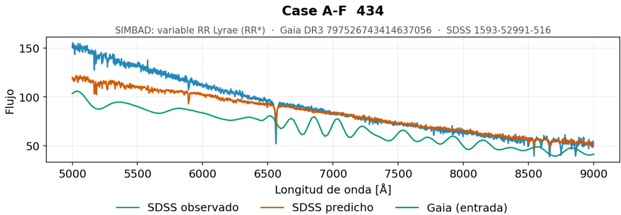
Figura 5.16. Secuencia central, alta luminosidad y alta temperatura, ejemplo 1. Espectro generado por el modelo de redes neuronales densas con normalización basada en la mediana de cada espectro para uno de los objetos con paralaje no significativo, por debajo de 0,01 mas, cuya magnitud absoluta no es fiable: SIMBAD lo identifica como una RR*, y no como una estrella de la secuencia principal.
