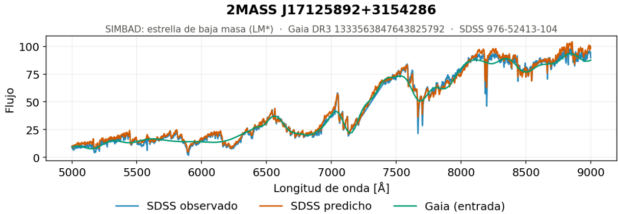
Figura 5.92. Secuencia central, baja luminosidad y baja temperatura, ejemplo 1. Espectro generado por el modelo de redes neuronales recurrentes con una función de Atención para uno de los objetos del extremo frío de la secuencia, con estrellas de baja masa de unos 3 100 K y paralajes de entre 8 y 27 mas, es decir, objetos cercanos y poco luminosos.
