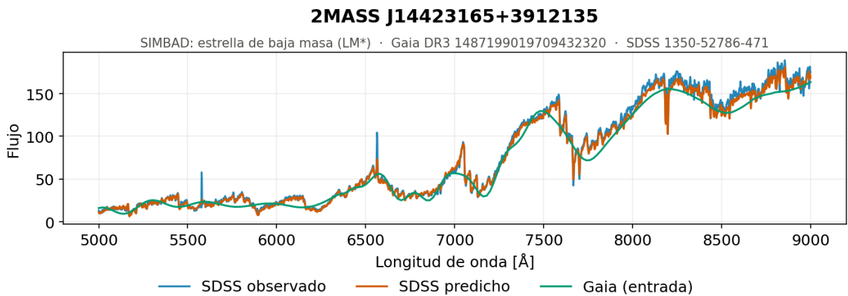
Figura 5.71. Secuencia central, baja luminosidad y baja temperatura, ejemplo 2. Espectro generado por el modelo de redes neuronales recurrentes con una capa de GRU para uno de los objetos del extremo frío de la secuencia, con estrellas de baja masa de unos 3 100 K y paralajes de entre 8 y 27 mas, es decir, objetos cercanos y poco luminosos.
