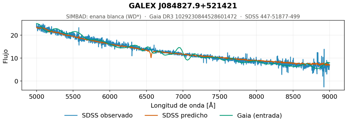
Figura 5.83. Enanas blancas, ejemplo 1. Espectro generado por el modelo de redes neuronales recurrentes con una capa bidireccional para una de las enanas blancas, objetos calientes y poco luminosos cuyo espectro es un continuo decreciente con muy pocos rasgos.
