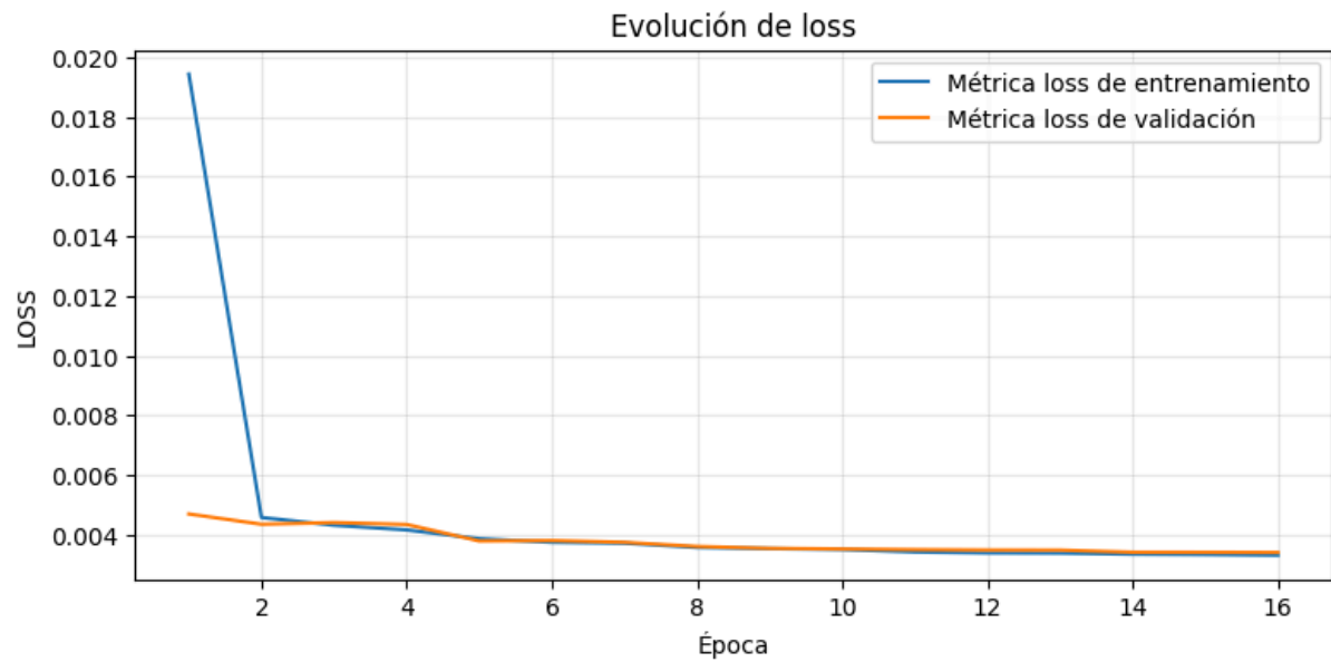
Figura 5.13. Evolución de la pérdida durante el entrenamiento de la red densa con normalización basada en la mediana
