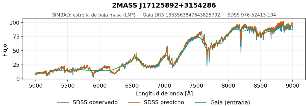
Figura 5.20. Secuencia central, baja luminosidad y baja temperatura, ejemplo 1. Espectro generado por el modelo de redes neuronales densas con normalización basada en la mediana de cada espectro para uno de los objetos del extremo frío de la secuencia, con estrellas de baja masa de unos 3 100 K y paralajes de entre 8 y 27 mas, es decir, objetos cercanos y poco luminosos.
