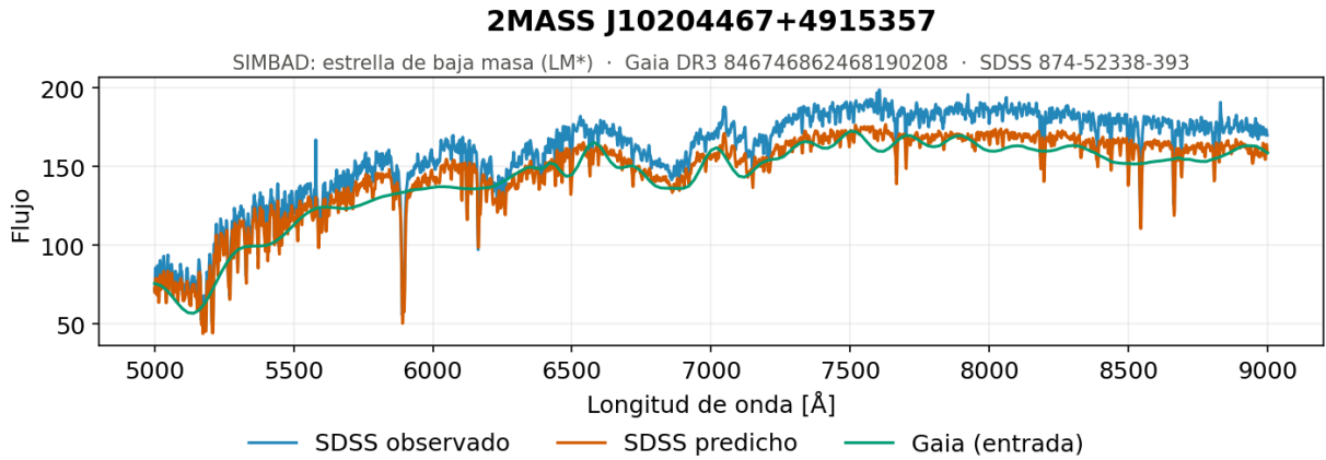
Figura 5.8. Secuencia central, ejemplo 2. Espectro generado por el modelo de redes neuronales densas con normalización global para una de las estrellas del tramo central de la secuencia, el grupo más poblado de la muestra con 655 objetos, formado por estrellas de baja masa con temperaturas efectivas en torno a 4 500 K.
