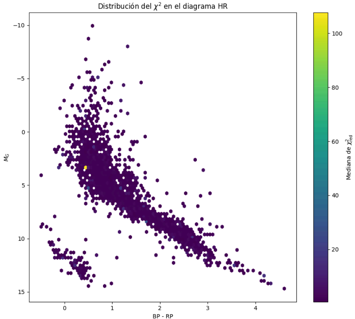
Figura 6.1. Diagrama HR del estadístico \chi^2 normalizado aplicado sobre la muestra de test en el modelo denso.
