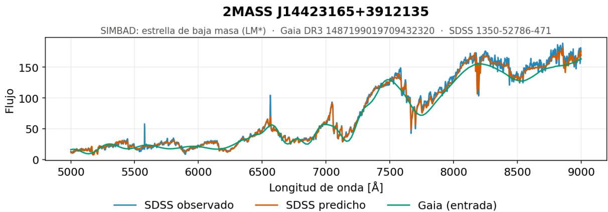
Figura 5.63. Secuencia central, baja luminosidad y baja temperatura, ejemplo 2. Espectro generado por el modelo convolucional U-Net para uno de los objetos del extremo frío de la secuencia, con estrellas de baja masa de unos 3 100 K y paralajes de entre 8 y 27 mas, es decir, objetos cercanos y poco luminosos.
