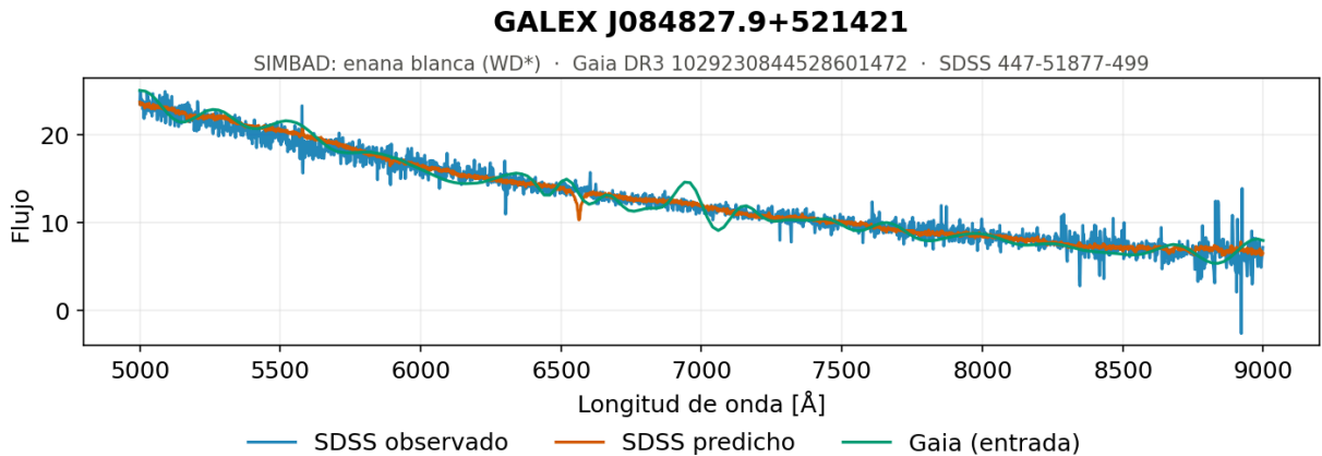
Figura 5.42. Enanas blancas, ejemplo 1. Espectro generado por el modelo de redes neuronales densas con la SNR de Gaia como entrada para una de las enanas blancas, objetos calientes y poco luminosos cuyo espectro es un continuo decreciente con muy pocos rasgos.
