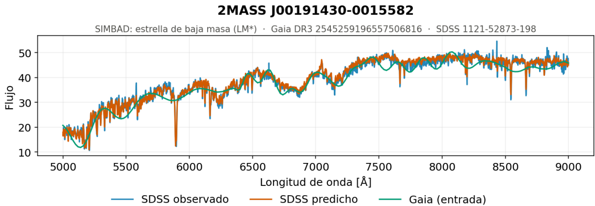
Figura 5.7. Secuencia central, ejemplo 1. Espectro generado por el modelo de redes neuronales densas con normalización global para una de las estrellas del tramo central de la secuencia, el grupo más poblado de la muestra con 655 objetos, formado por estrellas de baja masa con temperaturas efectivas en torno a 4 500 K.
