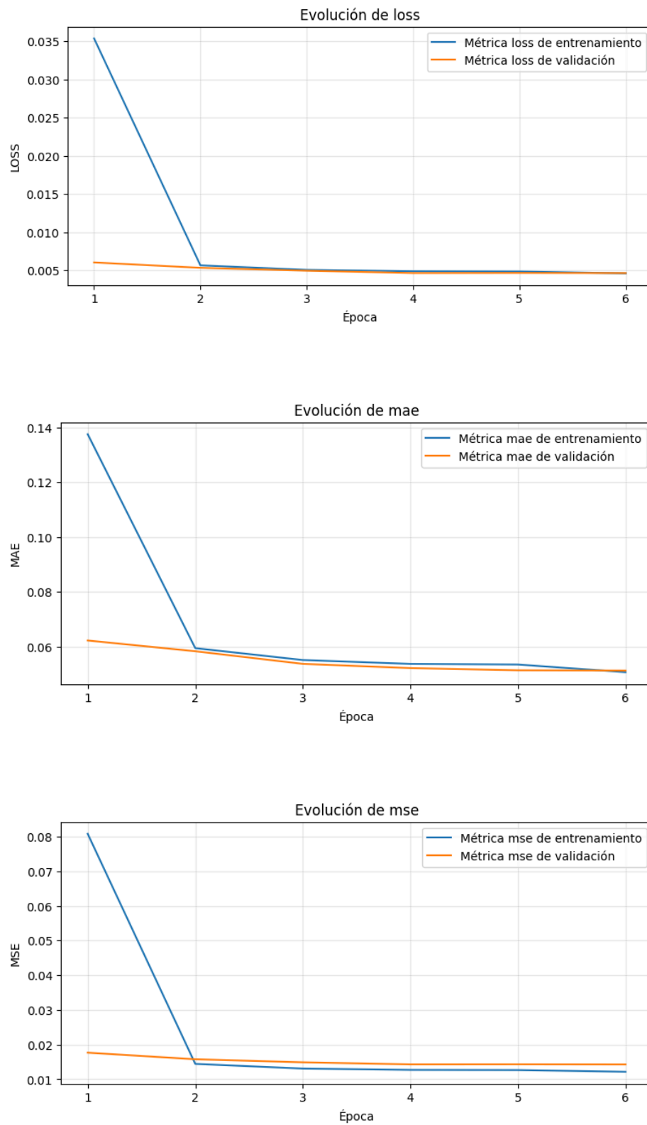
Figura 5.16. Gráficas de la evolución de las métricas de entrenamiento del modelo basado en una capa Bidireccional
