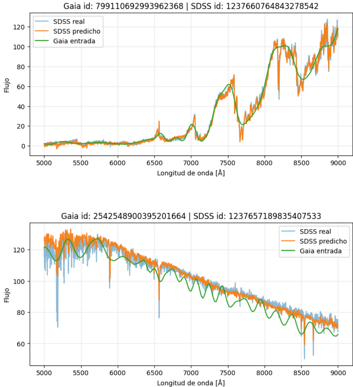
Figura 5.17. Ejemplos de espectros generados por el modelo de redes neuronales recurrentes con una función de Atención.
