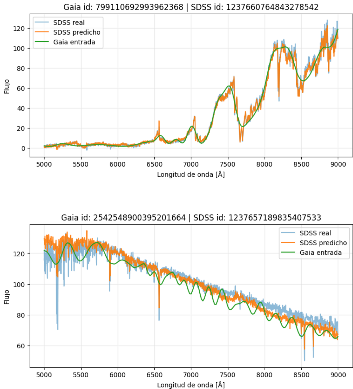
Figura 5.15. Ejemplos de espectros generados por el modelo de redes neuronales recurrentes con una capa bidireccional.
