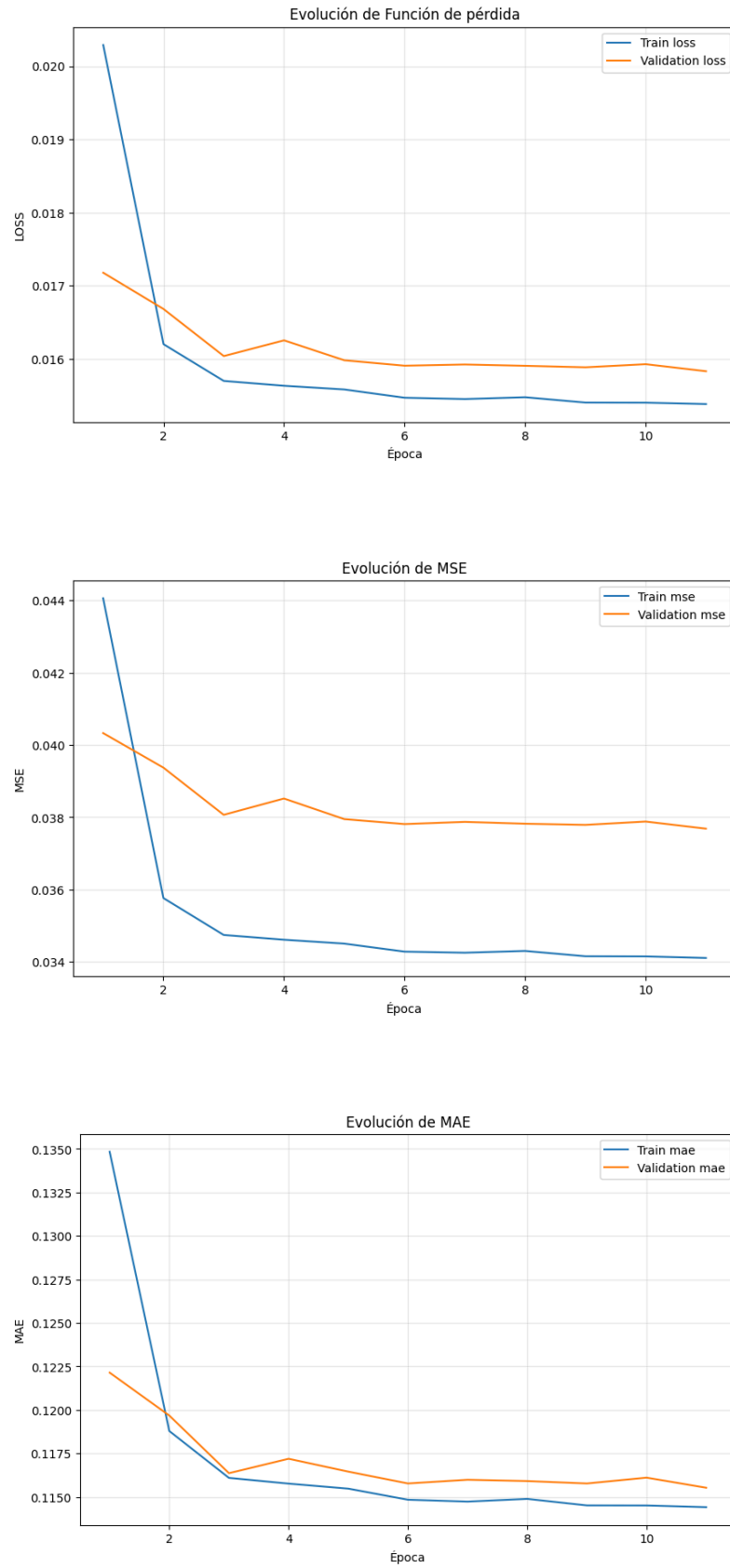
Figura 5.8. Gráficas de las métricas de evolución de entranamiento en modelo convolucional 1D
