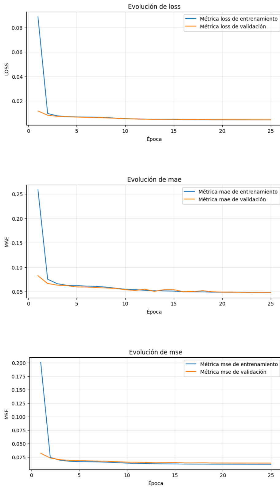
Figura 5.14. Gráficas de la evolución de las métricas de entrenamiento del modelo basado en una capa GRU
