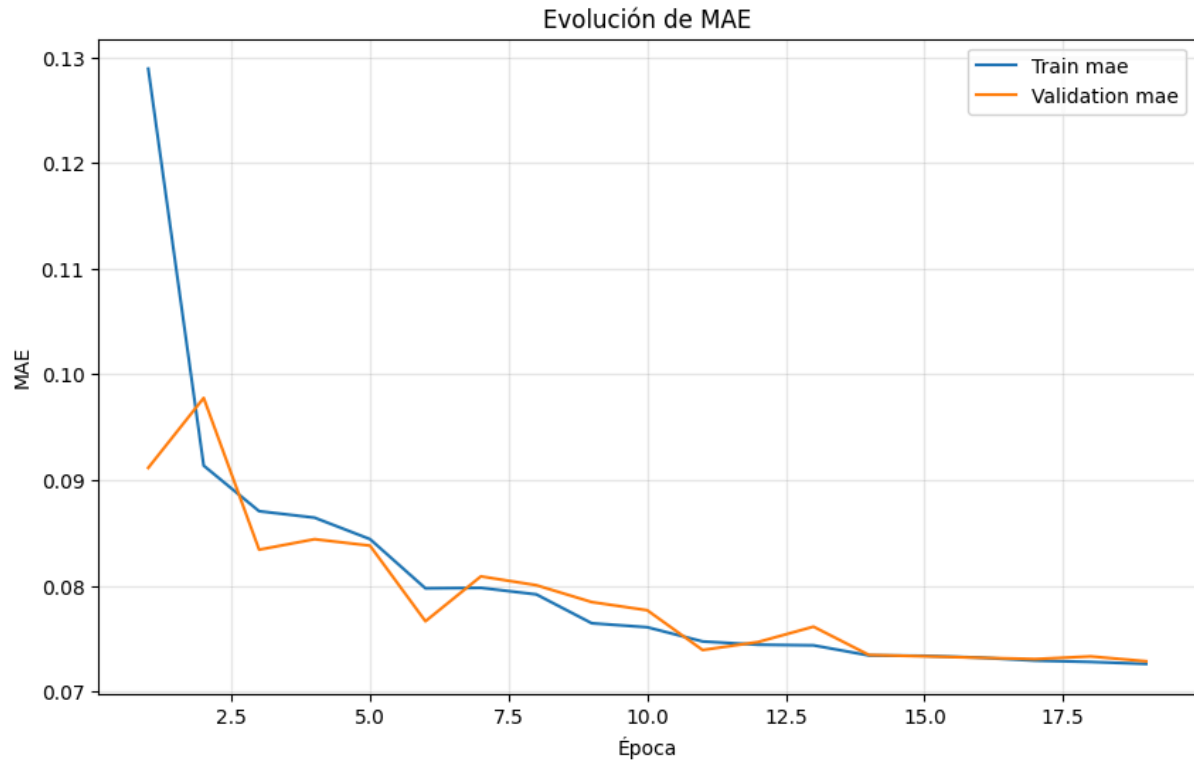
Figura 6.3. Gráfica de la evolución del MAE
