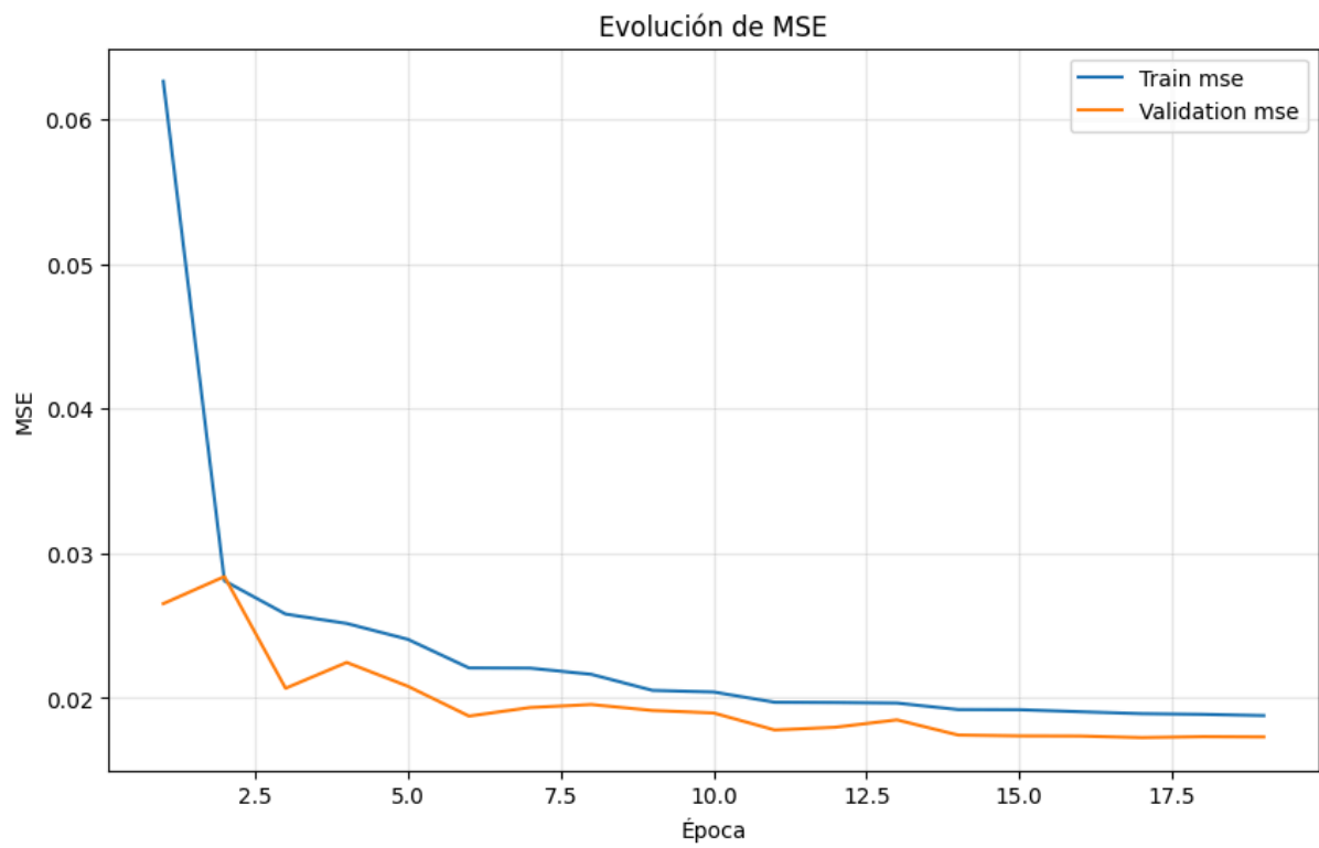
Figura 6.2. Gráfica de la evolución del MSE
