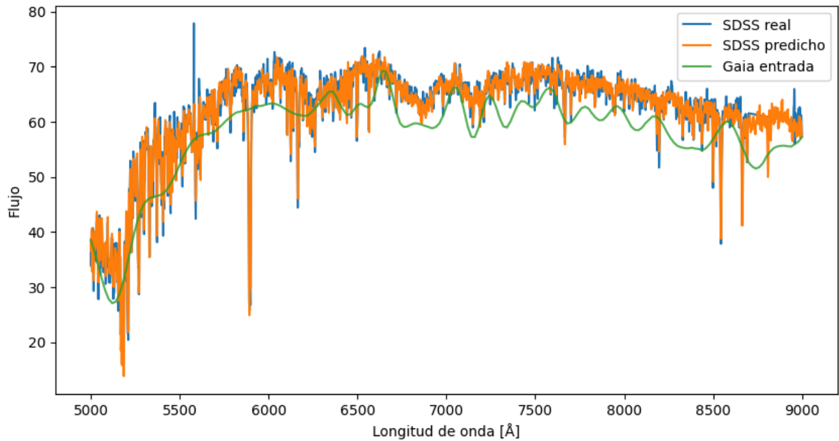
Figura 6.11. Ejemplo 2 del espectro generado por el modelo de redes neuronales densas con la variable SNR como entrada.
