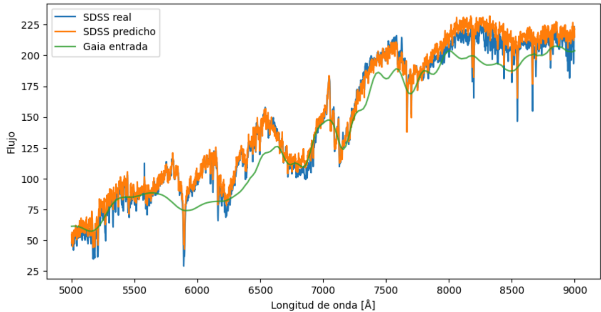
Figura 6.10. Ejemplo 1 del espectro generado por el modelo de redes neuronales densas con la variable SNR como entrada.
