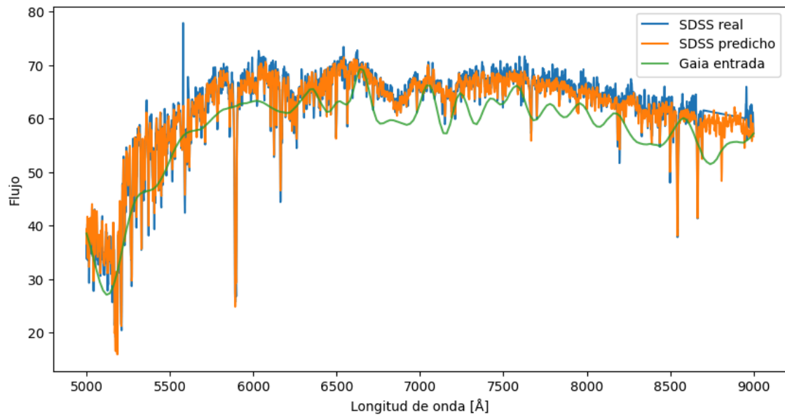
Figura 6.9: Ejemplo 2 del espectro generado por el modelo de redes neuronales densas y una normalización basada en el máximo de cada espectro.
