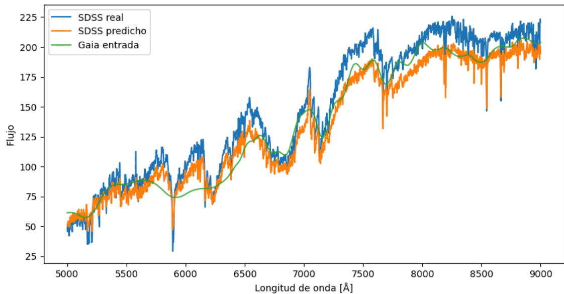
Figura 6.8: Ejemplo 1 del espectro generado por el modelo de redes neuronales densas y una normalización basada en el máximo de cada espectro.
