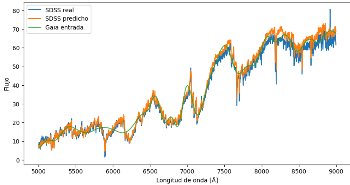
Figura 6.4: Ejemplo 1 del espectro generado por el modelo de redes neuronales densas y una normalización basada en la mediana del conjunto de entrenamiento.
