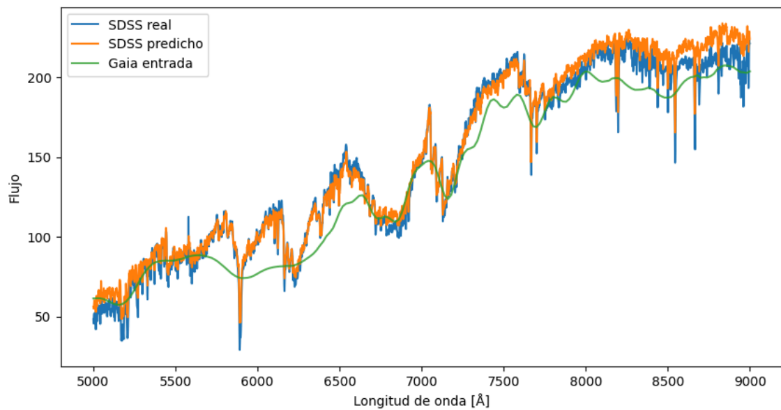
Figura 6.6: Ejemplo 1 del espectro generado por el modelo de redes neuronales densas y una normalización basada en la mediana de cada espectro.
