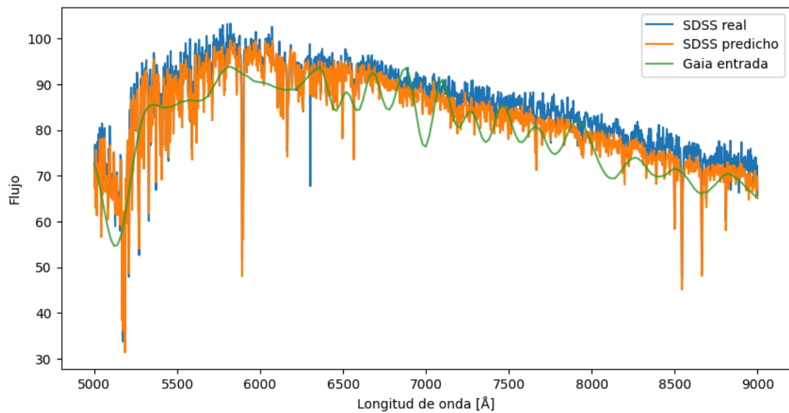
Figura 6.5: Ejemplo 2 del espectro generado por el modelo de redes neuronales densas y una normalización basada en la mediana del conjunto de entrenamiento.
