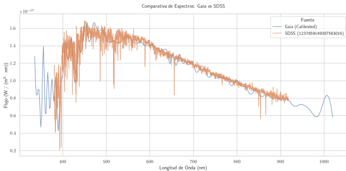
Figura 3.2: Ejemplo aleatorio del espectro captado de un mismo cuerpo por Gaia y SDSS. Podemos observar como claramente el intervalo que SDSS cubre es muy similar a Gaia, pero existe una gran diferencia en cuanto a la suavidad de las curvas representadas. Como vemos, SDSS incluye muchos más detalles que Gaia, su espectro tiene una calidad superior. Por otro lado, si nos fijamos en los datos captados en los extremos de visión de Gaia, notamos la posibilidad de que en rangos inferiores a 400 nm estemos observando artefactos u obteniendo mediciones muy poco precisas. Lo mismo sucede en valores superiores a 950 nm.
