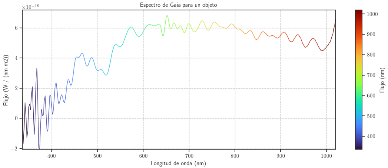
Figura 1: Ejemplo de espectro aleatorio captado por Gaia
