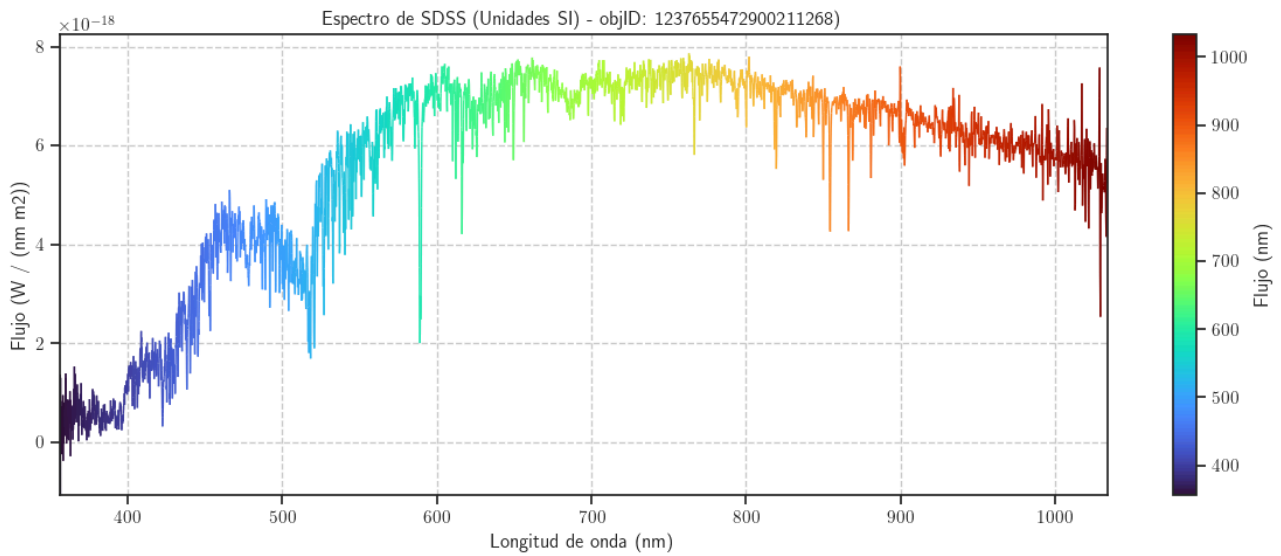
Figura 2: Espectro captado por SDSS del mismo cuerpo
