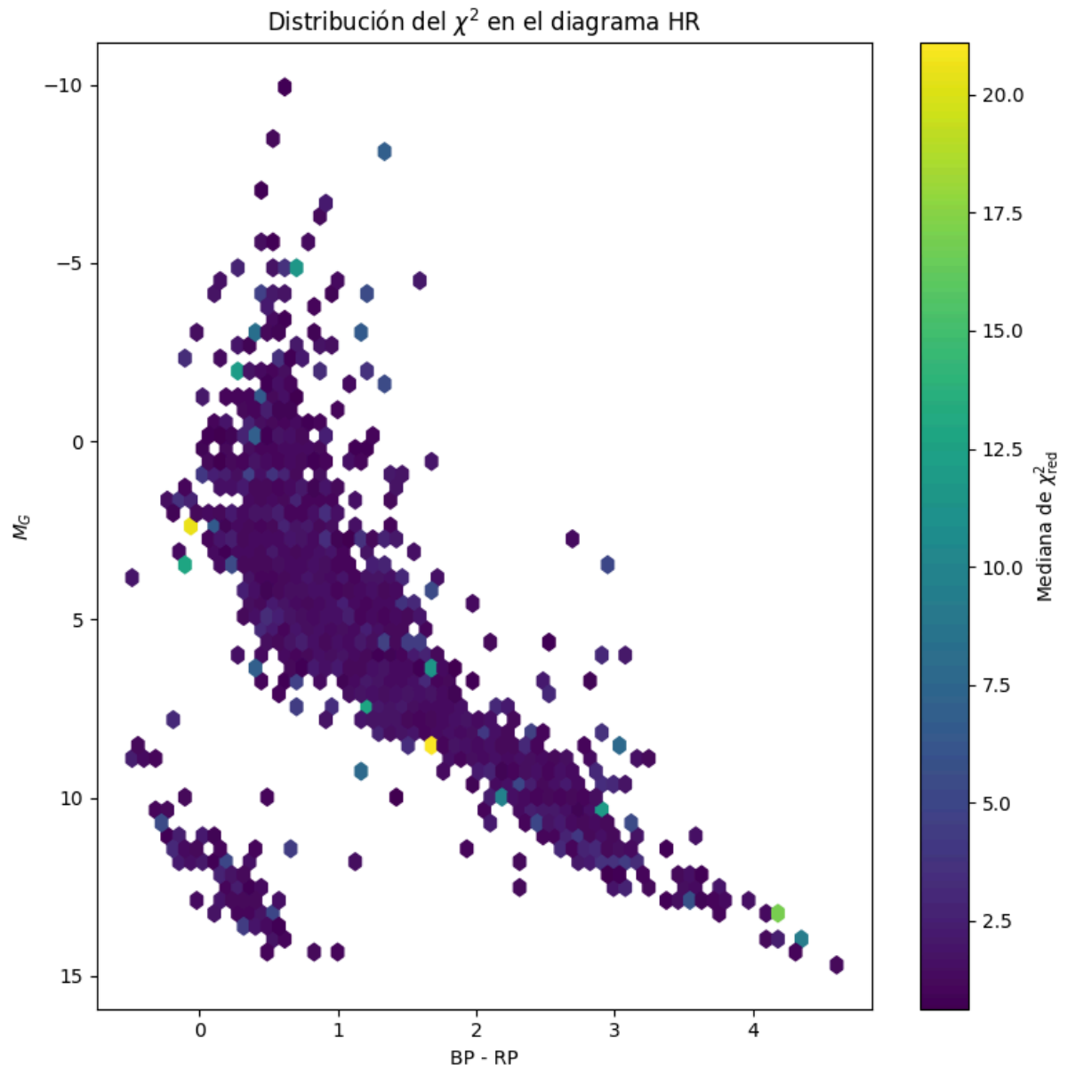
Figura 6.1. Diagrama HR del estadístico Chi-cuadrado aplicado sobre la muestra de test en el modelo denso.
