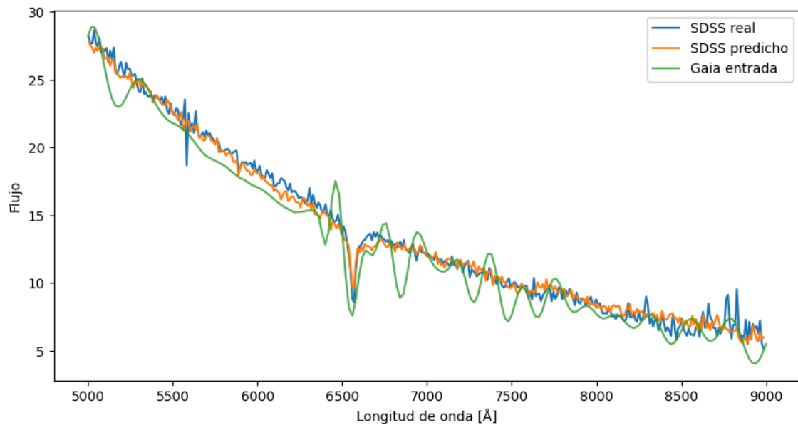
Figura 5.2: Ejemplo 2 del espectro generado por el modelo y los de Gaia y SDSS originales
