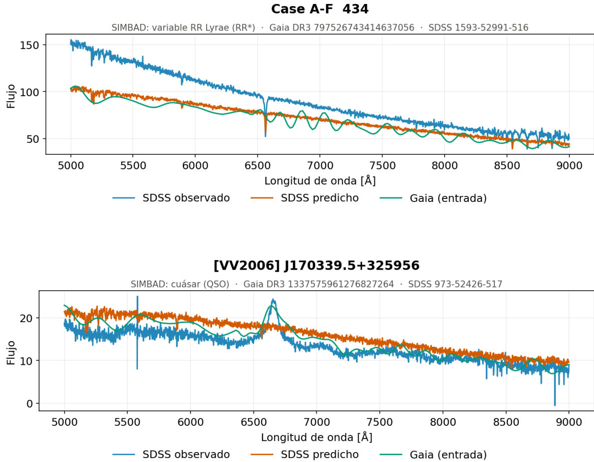
Figura 5.3. Secuencia central, alta luminosidad y alta temperatura. Espectros generados por el modelo de redes neuronales densas con normalización global para los objetos con paralaje no significativo, por debajo de 0,01 mas, cuya magnitud absoluta no es fiable: SIMBAD identifica la pareja como una RR* y un QSO, y no como estrellas de la secuencia principal.
