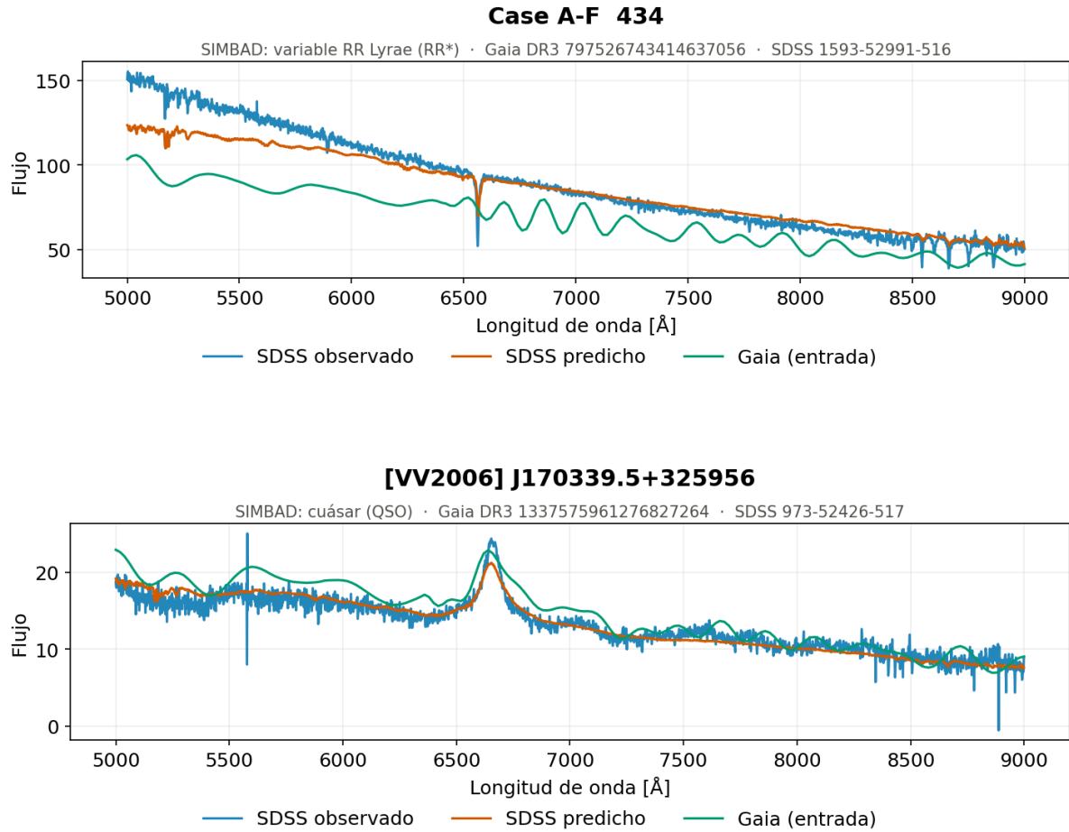
Figura 5.28. Secuencia central, alta luminosidad y alta temperatura. Espectros generados por el modelo convolucional U-Net para los objetos con paralaje no significativo, por debajo de 0,01 mas, cuya magnitud absoluta no es fiable: SIMBAD identifica la pareja como una RR* y un QSO, y no como estrellas de la secuencia principal.
