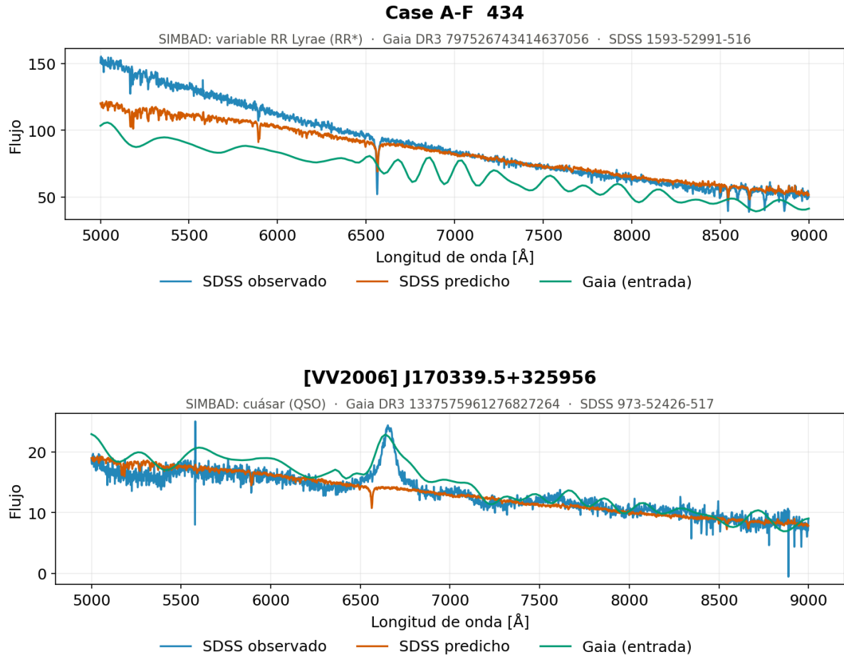
Figura 5.42. Secuencia central, alta luminosidad y alta temperatura. Espectros generados por el modelo de redes neuronales recurrentes con una función de Atención para los objetos con paralaje no significativo, por debajo de 0,01 mas, cuya magnitud absoluta no es fiable: SIMBAD identifica la pareja como una RR* y un QSO, y no como estrellas de la secuencia principal.
