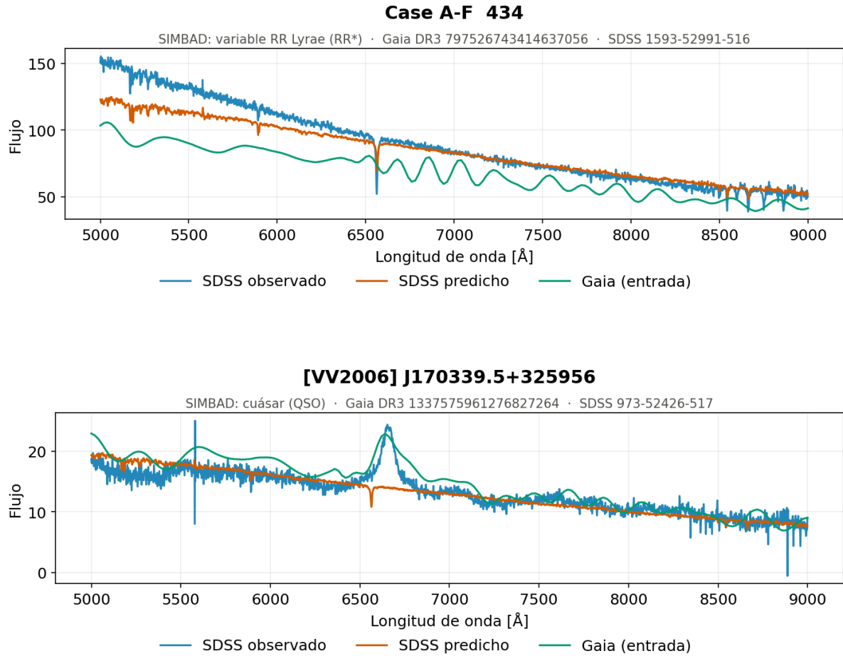
Figura 5.32. Secuencia central, alta luminosidad y alta temperatura. Espectros generados por el modelo de redes neuronales recurrentes con una capa de GRU para los objetos con paralaje no significativo, por debajo de 0,01 mas, cuya magnitud absoluta no es fiable: SIMBAD identifica la pareja como una RR* y un QSO, y no como estrellas de la secuencia principal.
