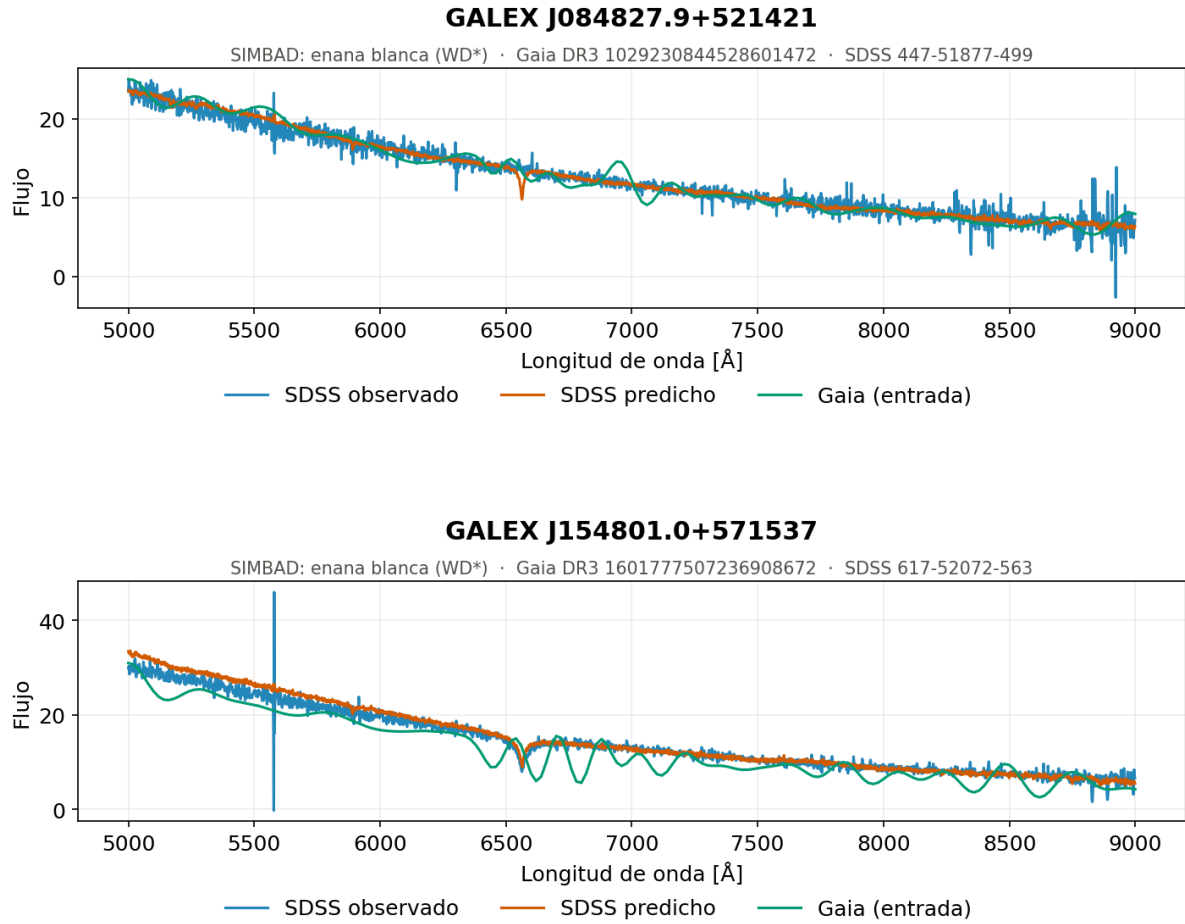
Figura 5.11. Enanas blancas. Espectros generados por el modelo de redes neuronales densas con normalización basada en la mediana de cada espectro para las enanas blancas, objetos calientes y poco luminosos cuyo espectro es un continuo decreciente con muy pocos rasgos.
