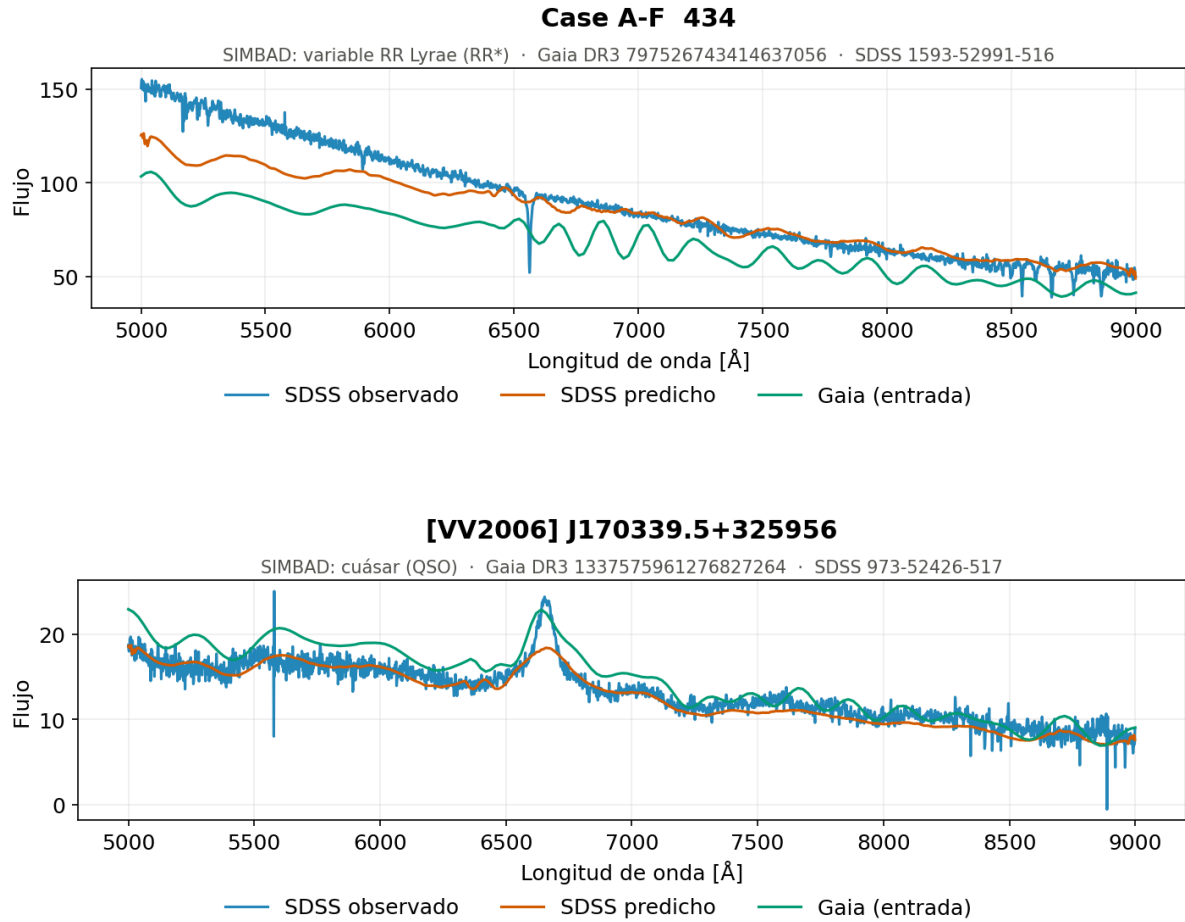
Figura 5.23. Secuencia central, alta luminosidad y alta temperatura. Espectros generados por el modelo convolucional 1D para los objetos con paralaje no significativo, por debajo de 0,01 mas, cuya magnitud absoluta no es fiable: SIMBAD identifica la pareja como una RR* y un QSO, y no como estrellas de la secuencia principal.
