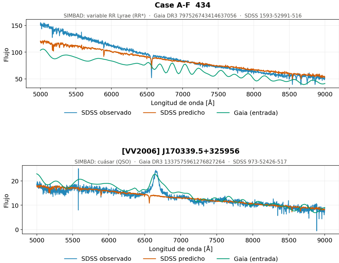
Figura 5.37. Secuencia central, alta luminosidad y alta temperatura. Espectros generados por el modelo de redes neuronales recurrentes con una capa bidireccional para los objetos con paralaje no significativo, por debajo de 0,01 mas, cuya magnitud absoluta no es fiable: SIMBAD identifica la pareja como una RR* y un QSO, y no como estrellas de la secuencia principal.
