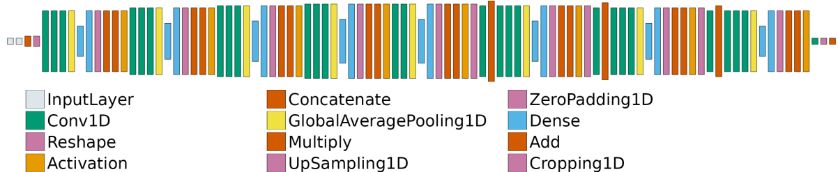
Figura 4.10. Arquitectura del modelo convolucional U-Net
