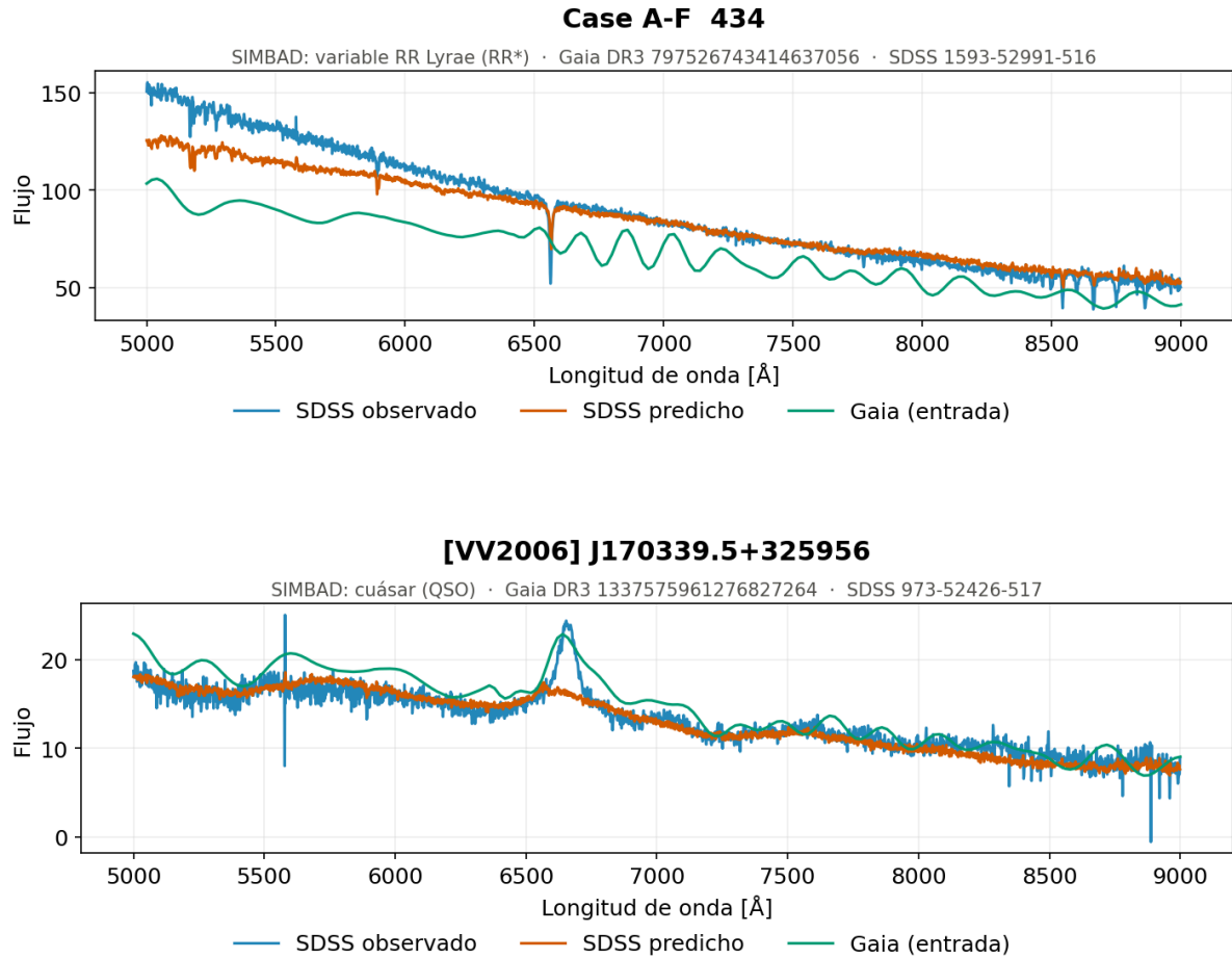
Figura 5.18. Secuencia central, alta luminosidad y alta temperatura. Espectros generados por el modelo de redes neuronales densas con la SNR de Gaia como entrada para los objetos con paralaje no significativo, por debajo de 0,01 mas, cuya magnitud absoluta no es fiable: SIMBAD identifica la pareja como una RR* y un QSO, y no como estrellas de la secuencia principal.
