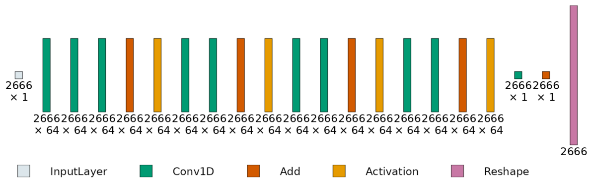
Figura 4.9. Arquitectura del modelo convolucional 1D
