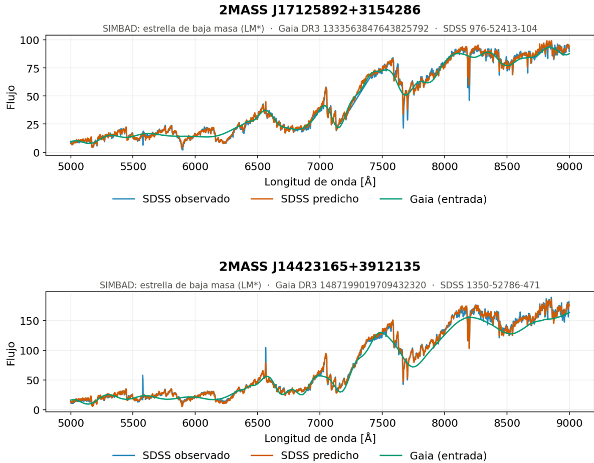
Figura 5.20. Secuencia central, baja luminosidad y baja temperatura. Espectros generados por el modelo de redes neuronales densas con la SNR de Gaia como entrada para el extremo frío de la secuencia, con estrellas de baja masa de unos 3 100 K y paralajes de entre 8 y 27 mas, es decir, objetos cercanos y poco luminosos.
