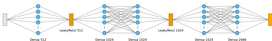
Figura 4.8. Arquitectura del modelo denso
