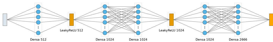
Figura 5.17. Arquitectura del modelo denso con la SNR
