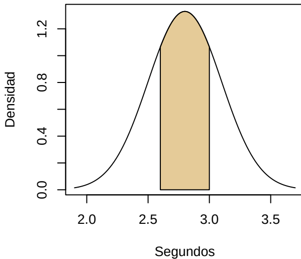
D. Normal(2.8, 0.3): P(2.6 < X < 3.0)
