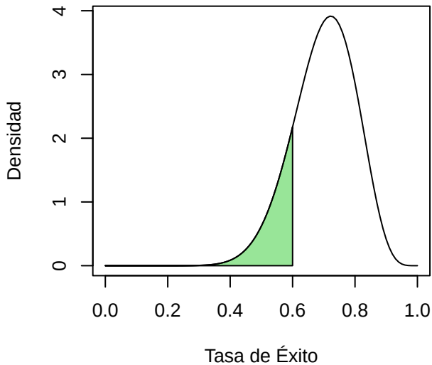
C. Beta(14,6): P(X < 0.60)
