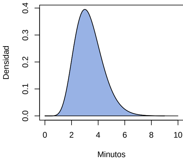
A. Gamma(10,3): P(X < 9)
