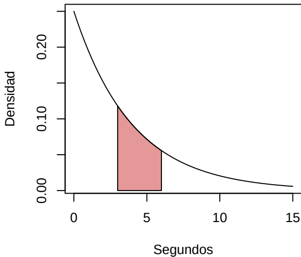
B. Exponencial(0.25): P(3 < X < 6)
