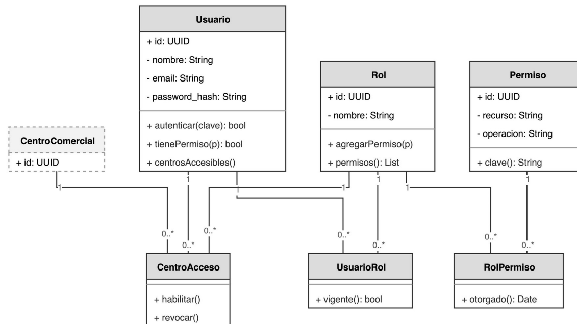
Figura 10.4. Clases de identidad y permisos: usuarios, roles, permisos y acceso multicentro. Fuente: elaboración propia (draw.io).
