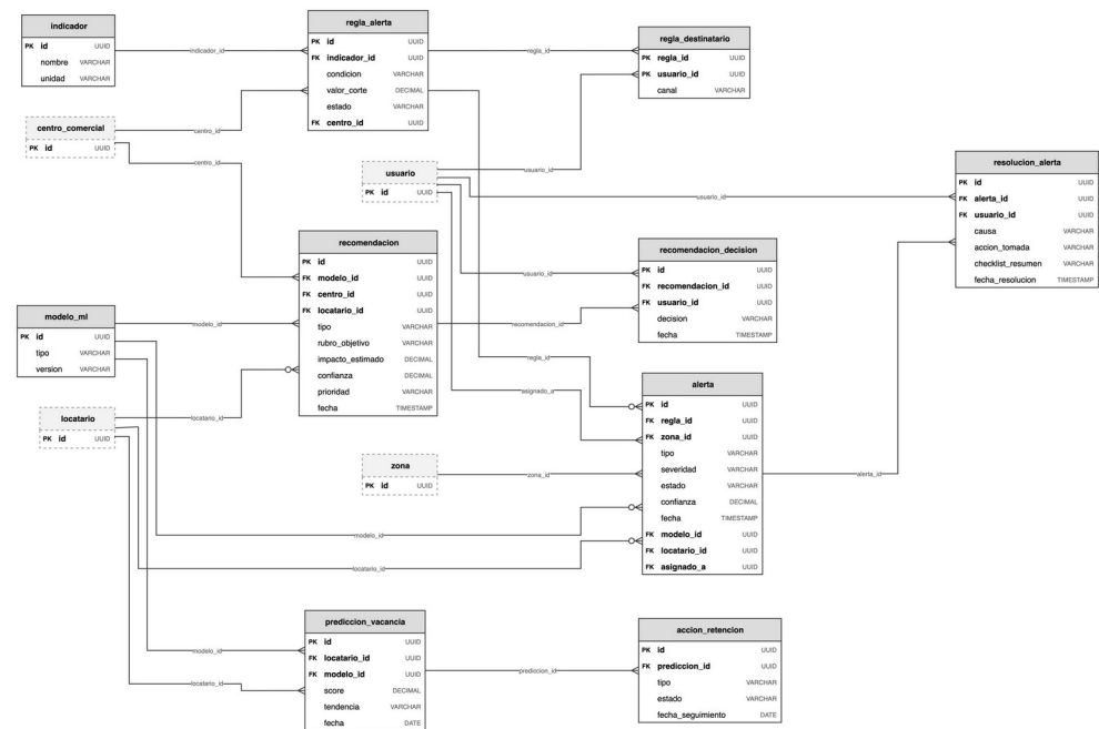
Figura 10.11. Indicadores, alertas y aprendizaje automático. Fuente: elaboración propia (draw.io).
