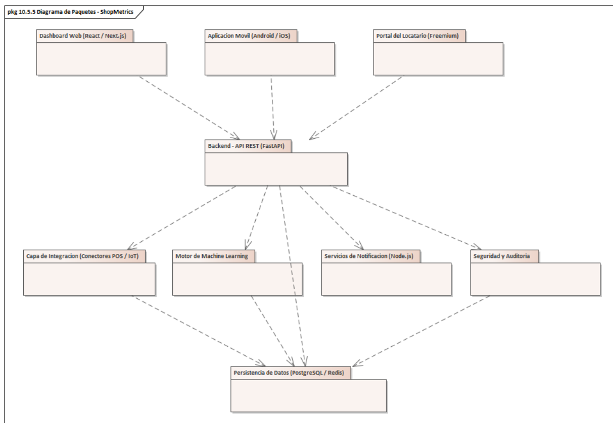
Figura 10.1. Diagrama de paquetes de ShopMetrics. Fuente: Enterprise Architect.
