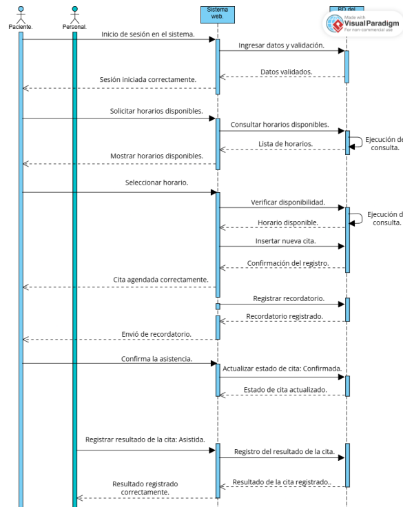
Ilustración 2: Flujo Principal
