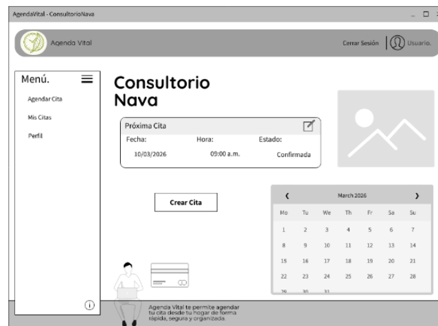
Ilustración 4: Pantalla Dashboard
