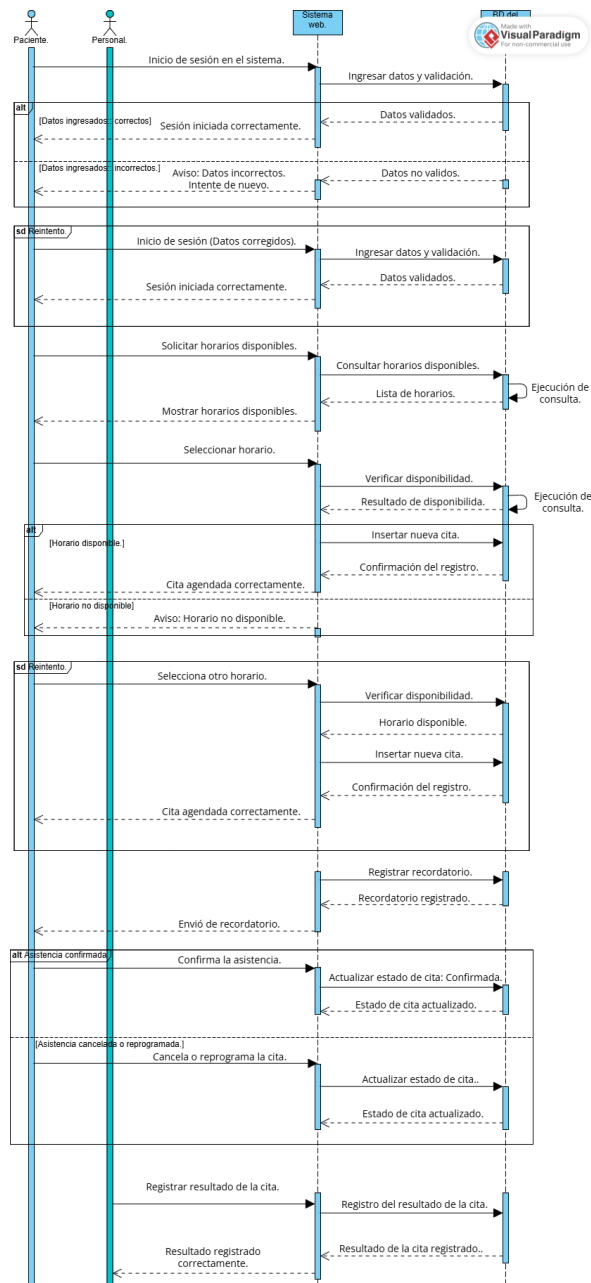
Ilustración 3: Flujo Crítico
