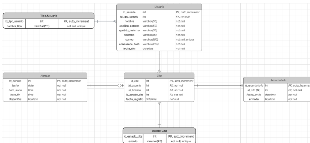
Ilustración 1: Diagrama ER
