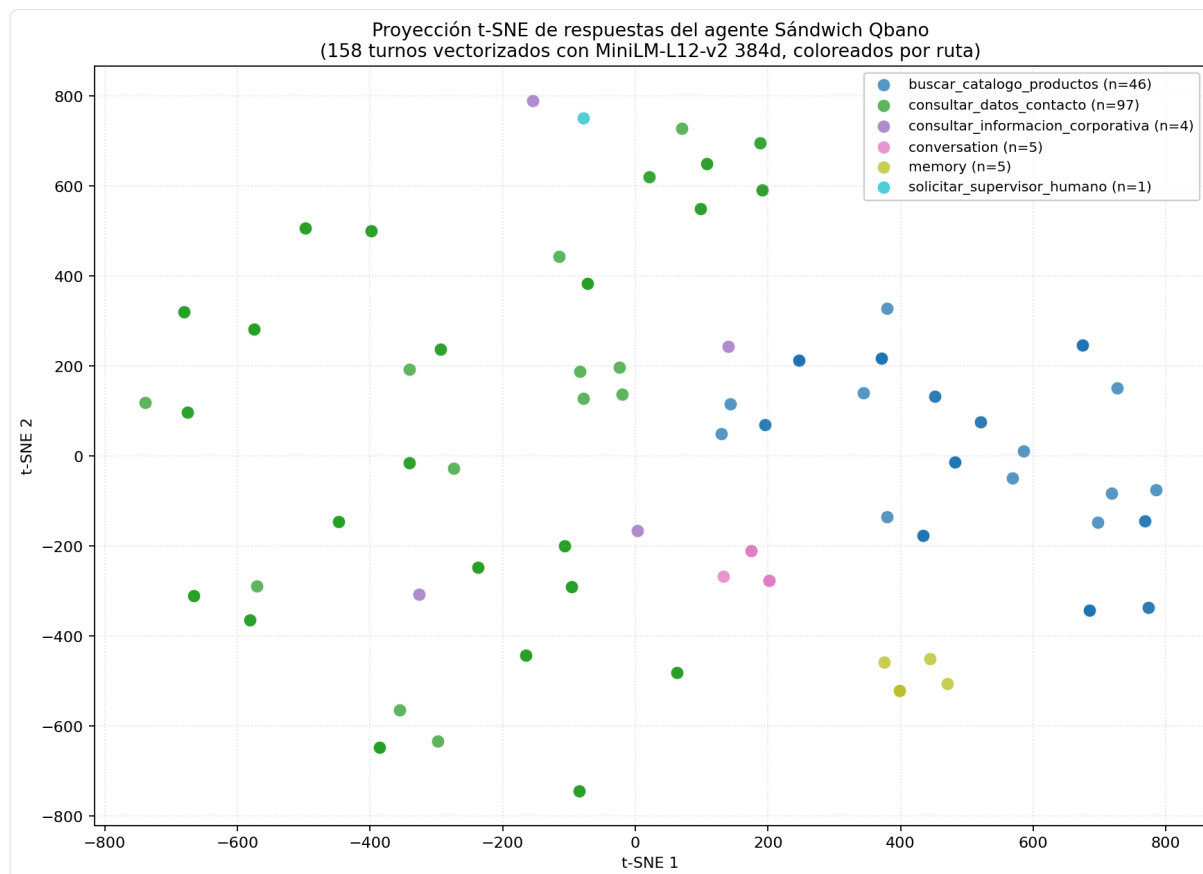
Proyección t-SNE 2D de las 158 respuestas del agente, coloreadas por ruta
