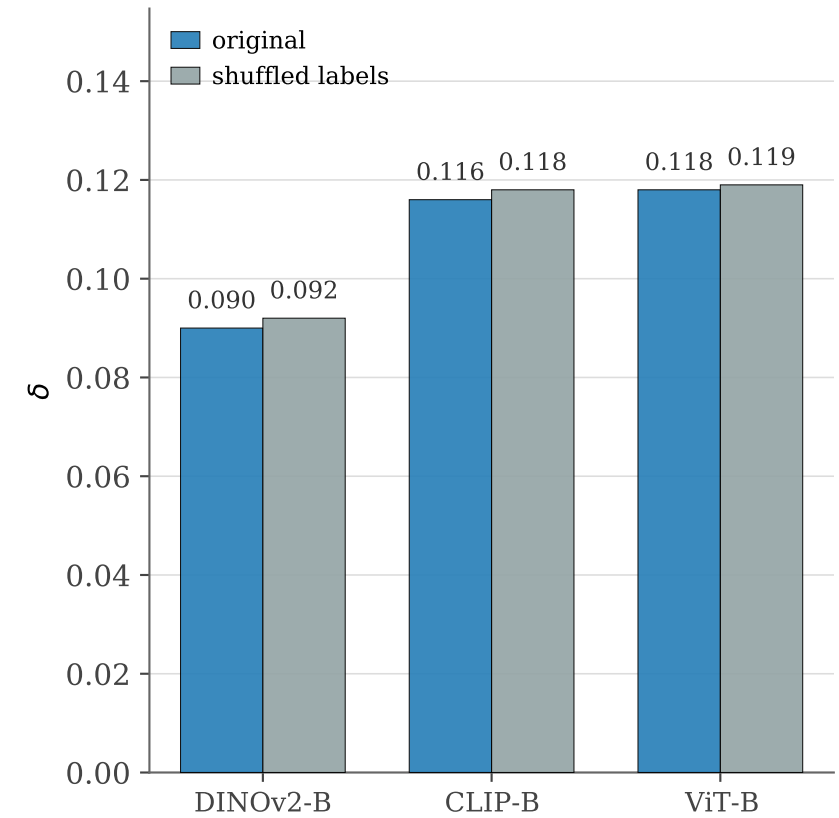
(d) Label shuffle preserves \delta
