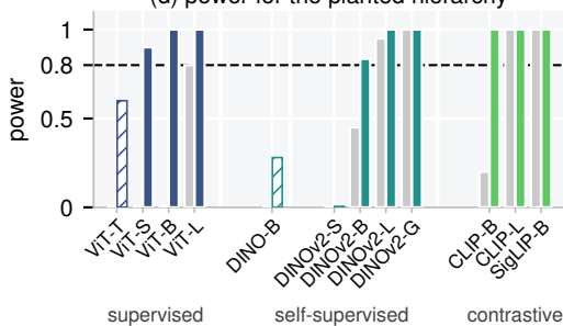
(d) power for the planted hierarchy
