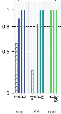
(d) power for a planted hierarchy
