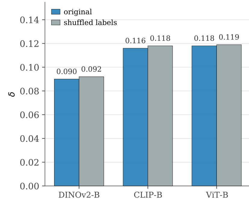
(d) Label shuffle preserves \delta
