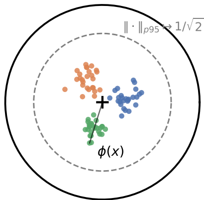
Poincaré ball (unit disk)
