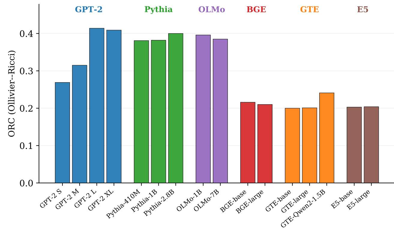
(d) Text: ORC by family
