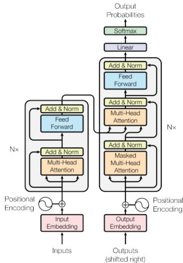
Figura 2.1: Arquitectura de un Transformer. Extraído de [?].
