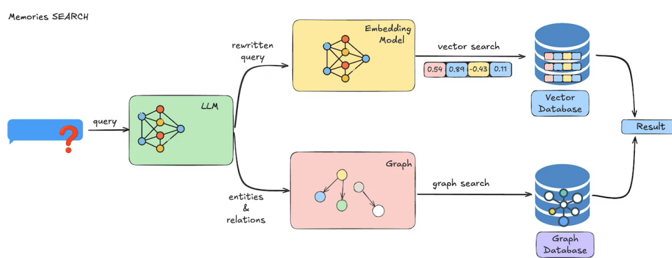
Figura 2.6: Pipeline de búsqueda de Mem0. Extraído de [?].
