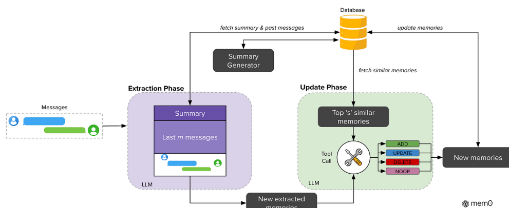
Figura 2.1: Pipeline de Mem0. Extraído de [1].
