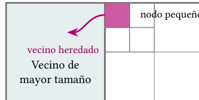
Figura 5.10: Enlazado de la vecindad mediante herencia del nodo padre. Cuando un nodo pequeño carece de un vecino de su mismo tamaño en una dirección, hereda como vecino el nodo de mayor tamaño adyacente a su padre, evitando una búsqueda exhaustiva entre celdas de distinto tamaño.
