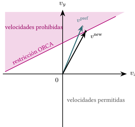
Figura 5.21: Resolución de la velocidad segura en el espacio de velocidades de ORCA. Cada agente vecino y la geometría inducen un semiplano de velocidades prohibidas (zona sombreada). Como la velocidad preferida v^{\text{pref}} cae en una región prohibida, el algoritmo escoge la velocidad factible v^{\text{new}} más próxima, sobre la frontera de la región segura.
