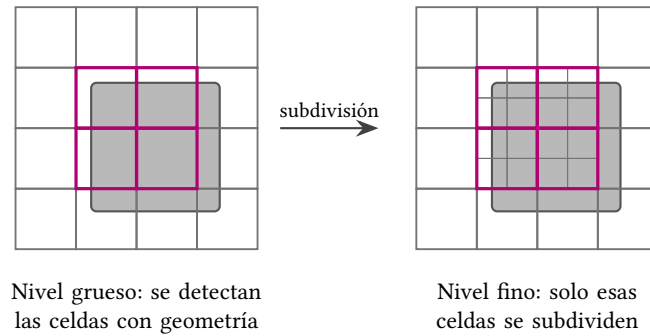
Figura 5.7: Barrido jerárquico de lo grueso a lo fino durante la rasterización. Las celdas vacías se descartan por completo; únicamente las que contienen geometría (resaltadas en rosa) se subdividen en el siguiente nivel de resolución.
