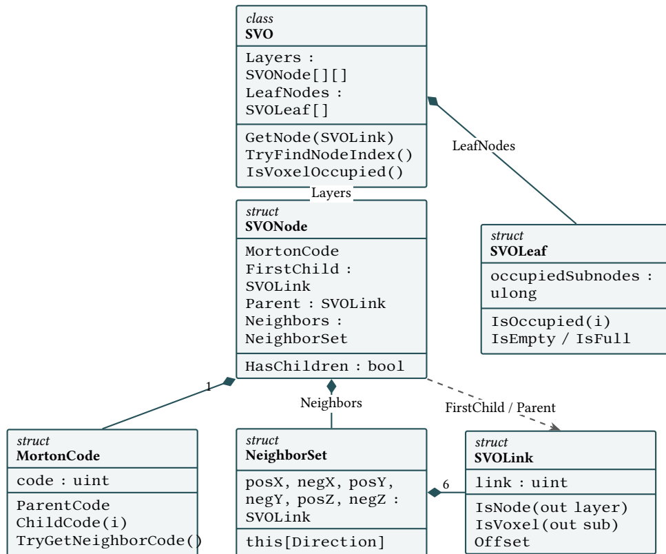
Figura 5.5: Estructuras de datos del espacio de nombres Core y sus relaciones. Los rombos denotan composición (propiedad de un valor) y las flechas discontinuas, referencias mediante enlaces. El SVO agrega las capas de SVONode y el vector paralelo de SVOLeaf ; cada nodo referencia a su primer hijo y a su padre, y agrega su conjunto de seis vecinos, todos ellos codificados como SVOLink (el puntero compacto de la Sección 5.2.4).
