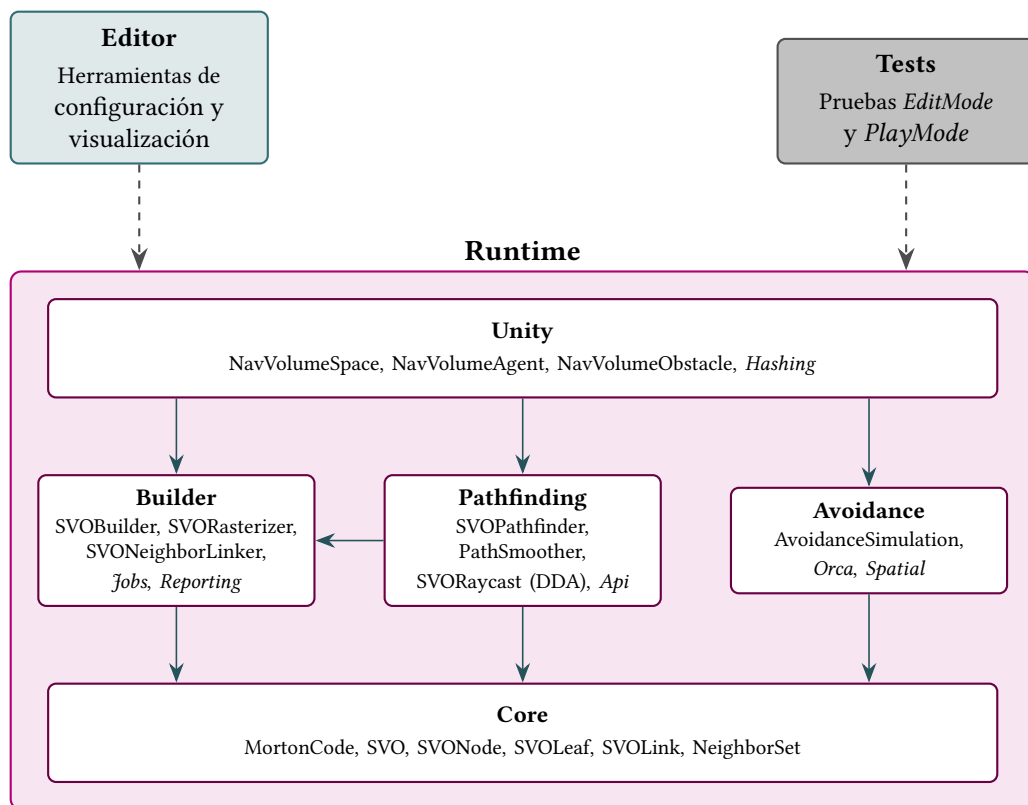
Figura 5.23: Arquitectura final del módulo Runtime y sus dependencias internas. Sobre el cimiento común Core se asientan Builder , Pathfinding y Avoidance (este último incorporado en la última iteración), y Unity orquesta a todos ellos exponiendo el sistema al motor. Las flechas señalan las dependencias principales entre espacios de nombres; los módulos Editor y Tests siguen dependiendo únicamente de Runtime (cf. Figura 5.1).
