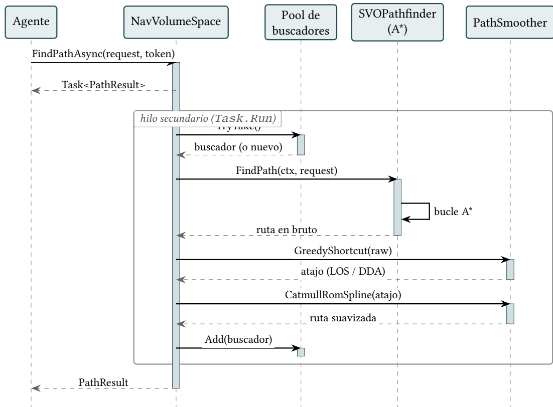
Figura 5.20: Secuencia de una petición de ruta asíncrona. Tras devolver de inmediato una Task, el cálculo prosigue en un hilo secundario: se toma un buscador de la reserva, se ejecuta la búsqueda A^* , se postprocesa la ruta (atajo por línea de visión y suavizado por spline ) y se devuelve el buscador a la reserva antes de entregar el resultado. La variante síncrona reutiliza un único buscador y prescinde del hilo secundario.
