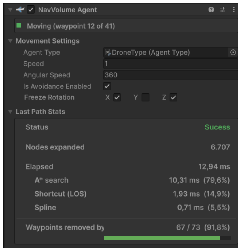
Figura B.4: Estadísticas en tiempo de ejecución de un agente. Imagen obtenida por medio de una captura de pantalla.
