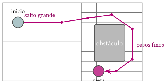
Figura 5.11: Expansión de A* sobre un grafo de resolución heterogénea. En el espacio abierto la búsqueda avanza con saltos grandes entre nodos de gran tamaño; al aproximarse al obstáculo, se ramifica en nodos y vóxeles cada vez más pequeños para rodearlo con precisión.
