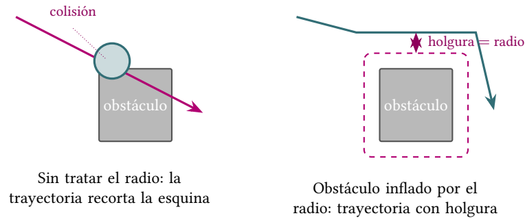
Figura 5.16: Corrección del clipping mediante el inflado de obstáculos por el radio del agente. Si no se considera el tamaño del agente, una trayectoria que recorta una esquina provoca colisión (izquierda). Al inflar el obstáculo por el radio del agente (margen discontinuo), la trayectoria conserva siempre la holgura necesaria (derecha).
