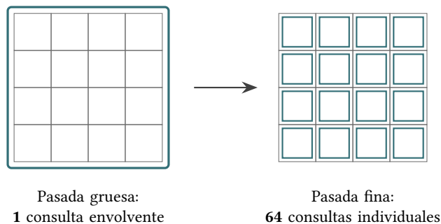
Figura 5.9: Pasada gruesa de descarte frente a pasada fina de muestreo. La pasada gruesa resuelve la hoja entera con una única consulta envolvente; solo si esta detecta geometría se ejecuta la pasada fina, con una consulta por vóxel (64 en una hoja de 4 \times 4 \times 4 ).
