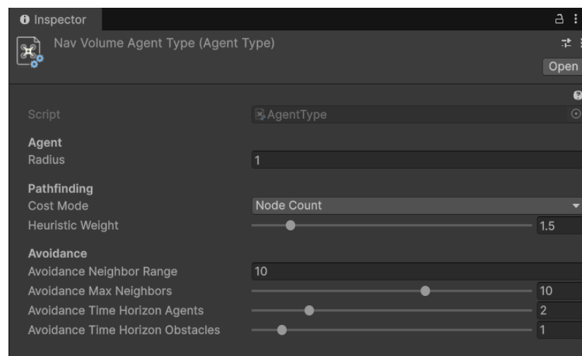
Figura B.2: Parámetros de configuración para un agente. Imagen obtenida por medio de una captura de pantalla.
