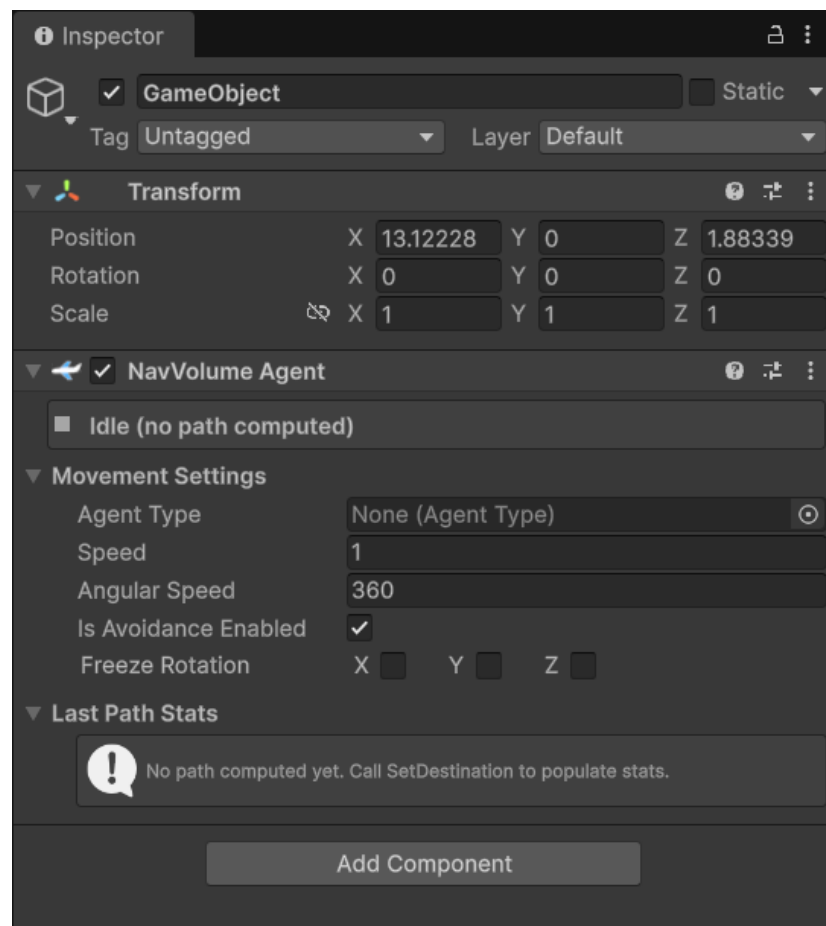
Figura B.3: Parámetros del componente NavVolumeAgent. Imagen obtenida por medio de una captura de pantalla.
