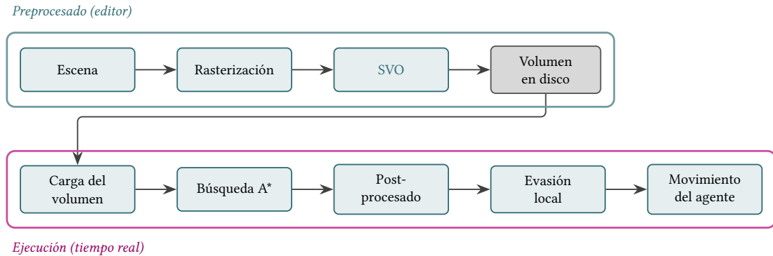
Figura 5.22: Flujo de datos global del sistema, del preprocesado a la ejecución. En el editor, la escena se rasteriza para construir el SVO, que se serializa en disco. En tiempo de ejecución, el volumen se carga y, sobre él, se resuelven las consultas de ruta (búsqueda, postprocesado y evasión local) que culminan en el movimiento del agente.
