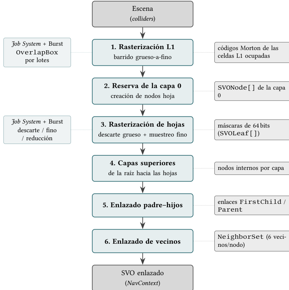
Figura 5.6: Canalización de construcción del SVO durante el bake . Cada etapa (centro) consume el producto de datos de la anterior (derecha); las etapas 1 y 3, dominadas por consultas físicas, se aceleran mediante el Job System y Burst (izquierda) y se detallan en las Figuras 5.7 y 5.9, mientras que el enlazado de la vecindad (etapa 6) se ilustra en la Figura 5.10.
