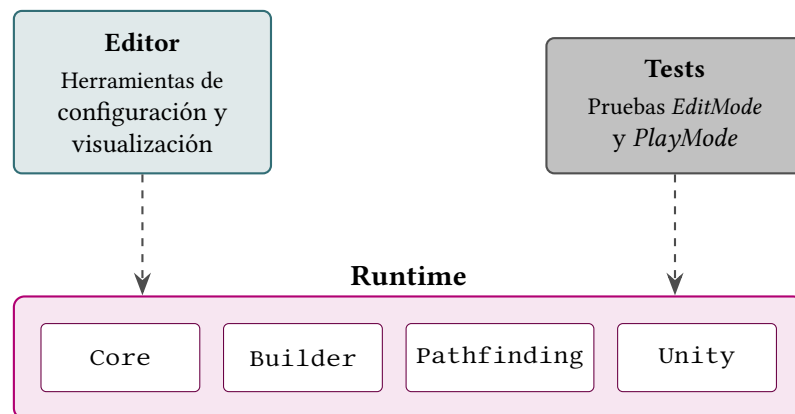
Figura 5.1: Arquitectura modular del sistema y sus dependencias. Los módulos Editor y Tests dependen del módulo Runtime (flechas discontinuas), pero nunca a la inversa; únicamente Runtime se incluye en la versión final del producto.
