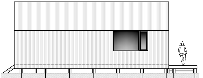
Elevacion Lateral Escala 1:50
