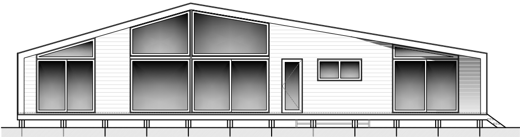
Elevacion Frontal Escala 1:50
