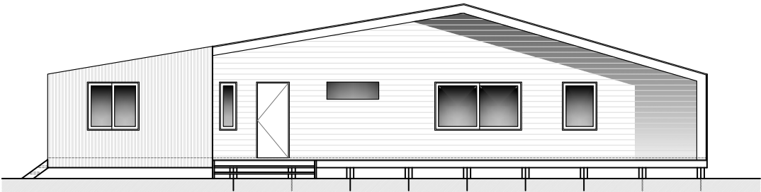
Elevacion Acceso Escala 1:50
