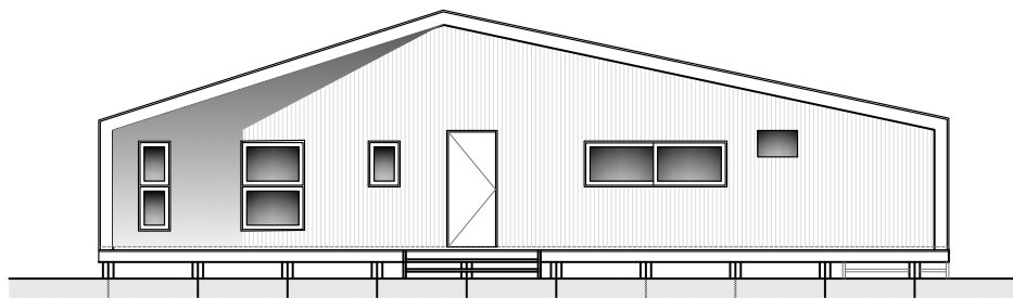
Elevacion Acceso Escala 1:50
