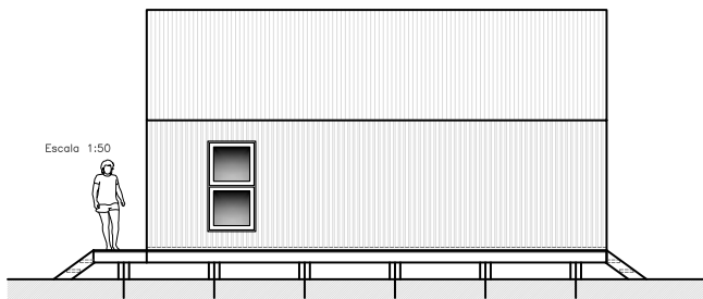
Elevacion Lateral Escala 1:50
