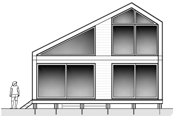
Elevacion Frontal Escala 1:50
