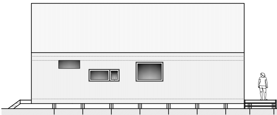
Elevacion Lateral Escala 1:50
