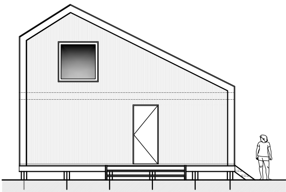
Elevacion Acceso Escala 1:50
