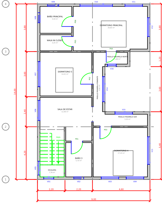
PLANTA SEGUNDO PISO 1:50
