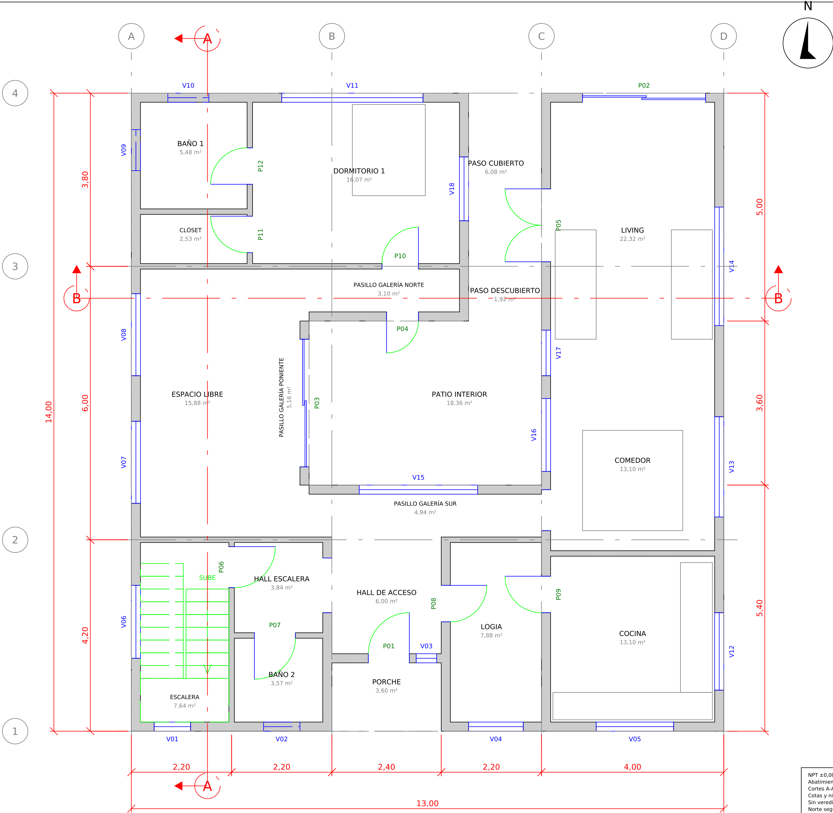
CUADRO DE SUPERFICIES — Primer Piso
