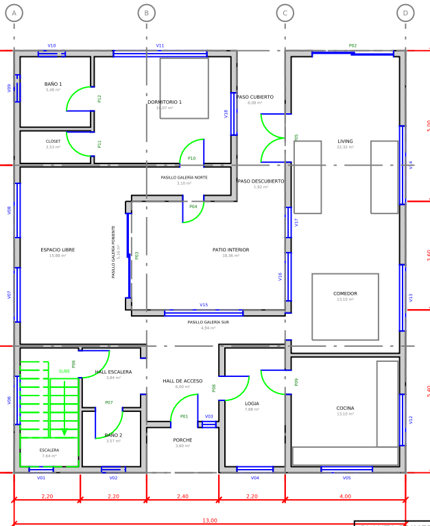
PLANTA PRIMER PISO 1:50
