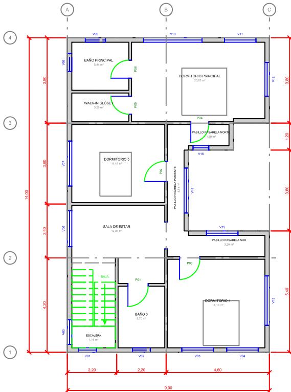
PLANTA SEGUNDO PISO 1:50
