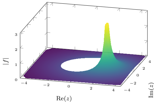
(d) Laurent: 2 < |z| < \infty
