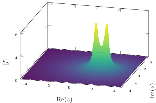
(a) Función original: \frac{1}{(1-z)(2-z)}
