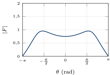
|F(e^{j\theta})| Circ. unit.
