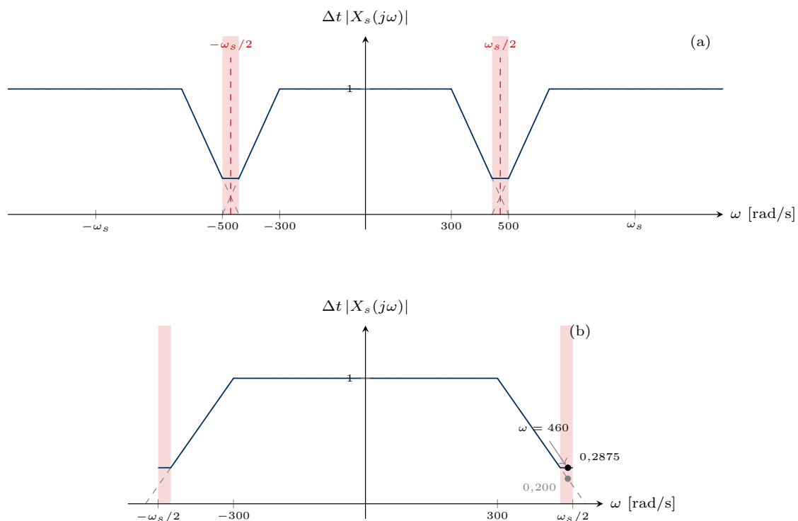
Figura 11: Ejercicio 16. (a) Espectro muestreado (azul) como suma de las copias (punteado gris) espaciadas \omega_s = 942,5 \text{ rad/s} ; en las zonas sombreadas las copias se solapan. (b) Detalle de la banda base: en punteado, el espectro original; en azul, lo que el muestreo entrega. Difieren solo en la zona sombreada, donde el espectro medido queda por encima del verdadero. La componente de 460 rad/s debería valer 0,200 y se mide 0,2875. Las alturas están normalizadas por 1/\Delta t .
