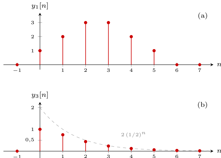
Figura 3: Ejercicio 3. (a) y_1[n] , el trapezio que producen dos pulsos rectangulares, soporte [0, 5] . (b) y_3[n] , junto con la exponencial 2(1/2)^n punteada, que gobierna el decaimiento para n grande.
