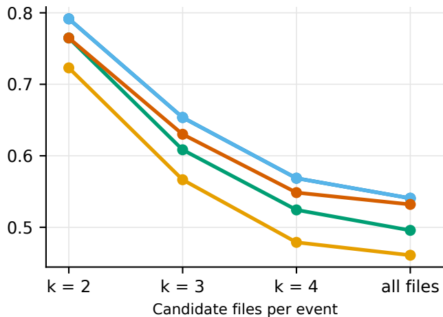
Precision@1
