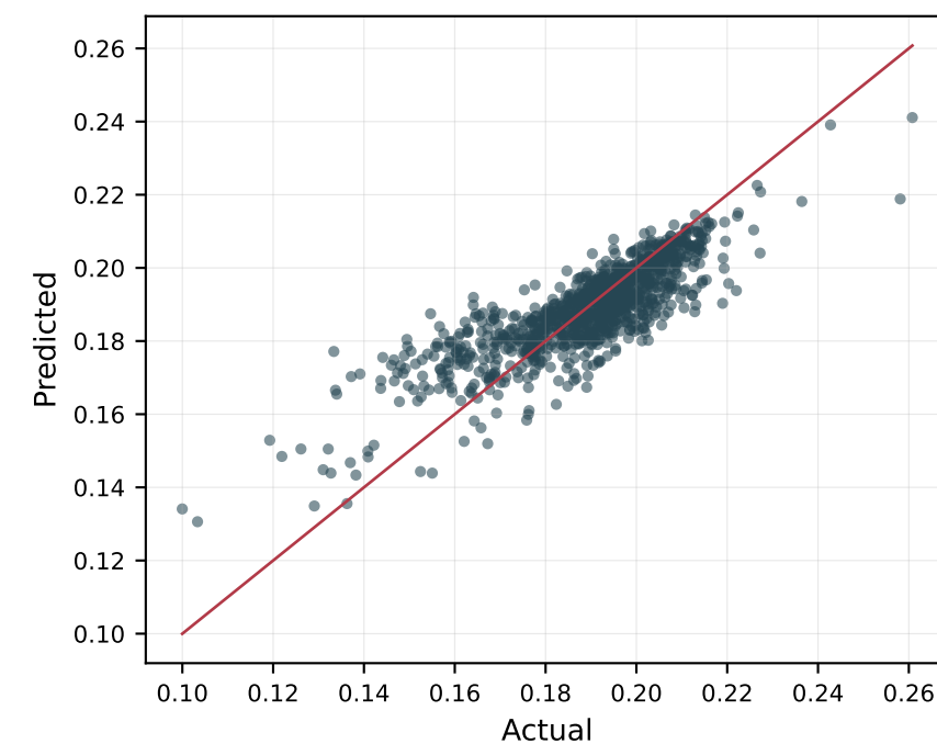
SVR RBF
