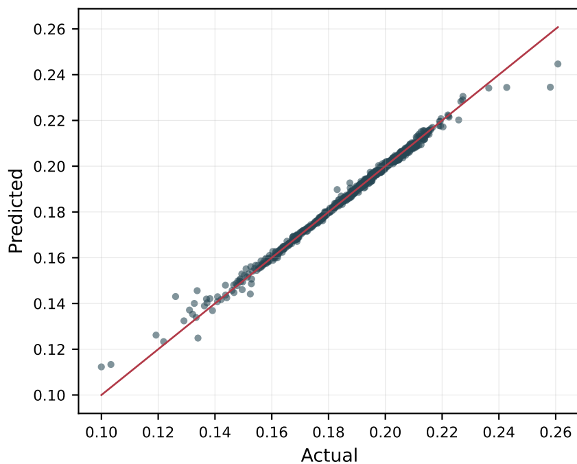
ANN Deep MLP
