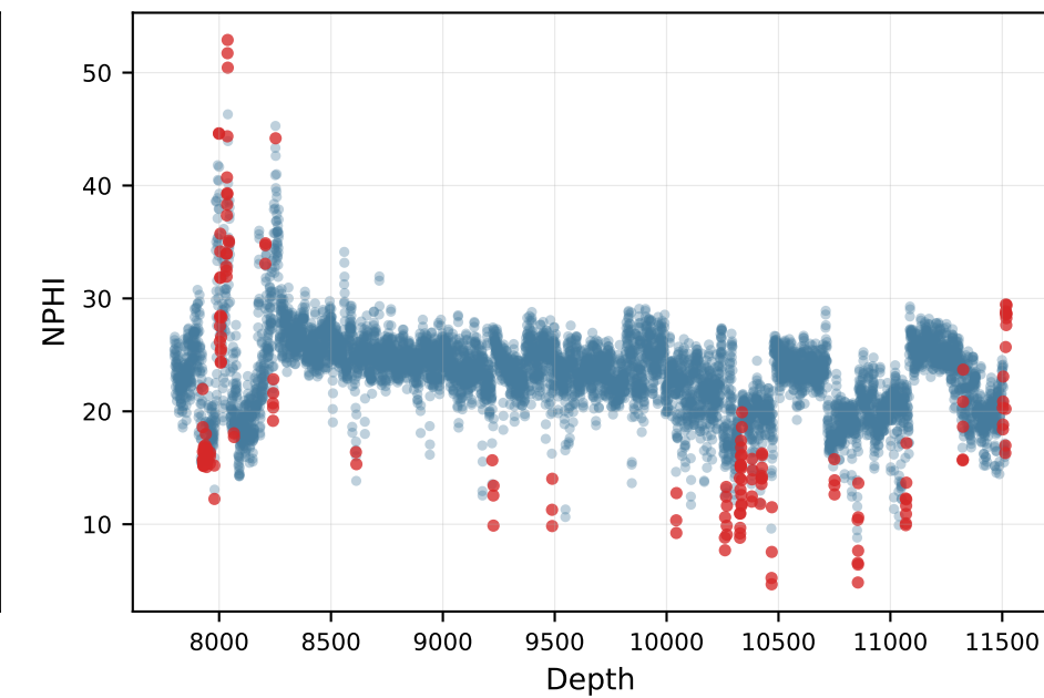
NPHI
