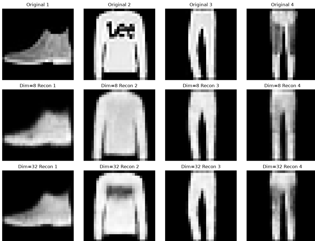
Figure 2: Perbandingan rekonstruksi antar latent dimension
