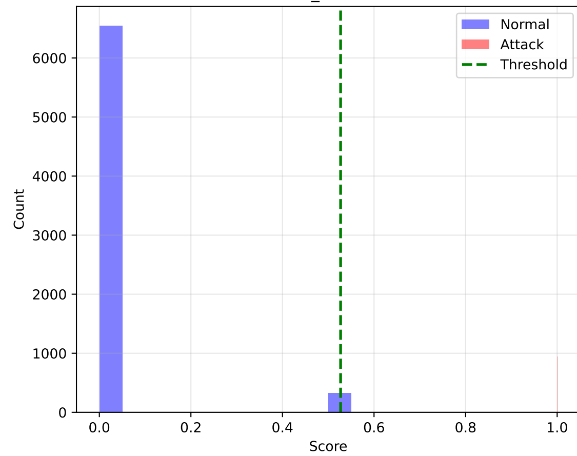
E_GRU
