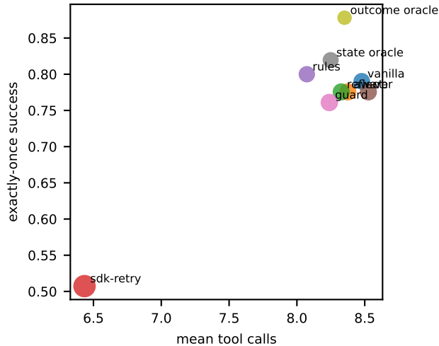
gpt-6-sol
