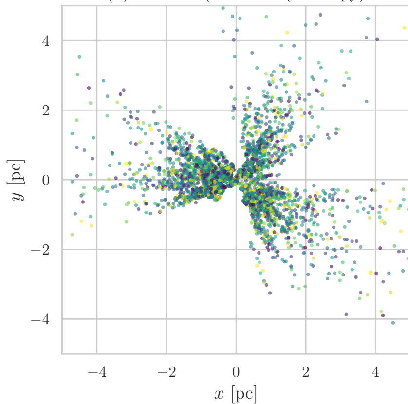
(d) D = 3.0 (uniform)
