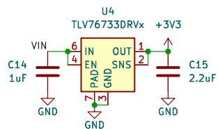
LDO
