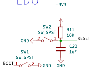
Buttons
