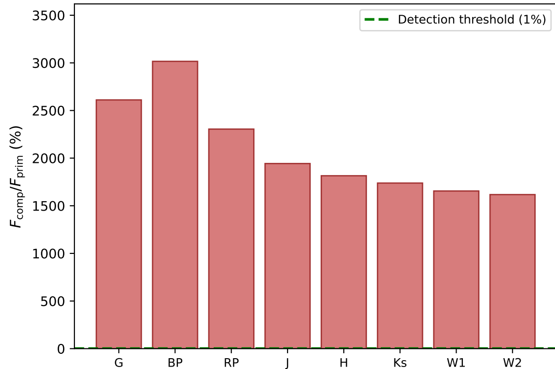
Companion flux if M_2 = 6.62 M_\odot (MS)
