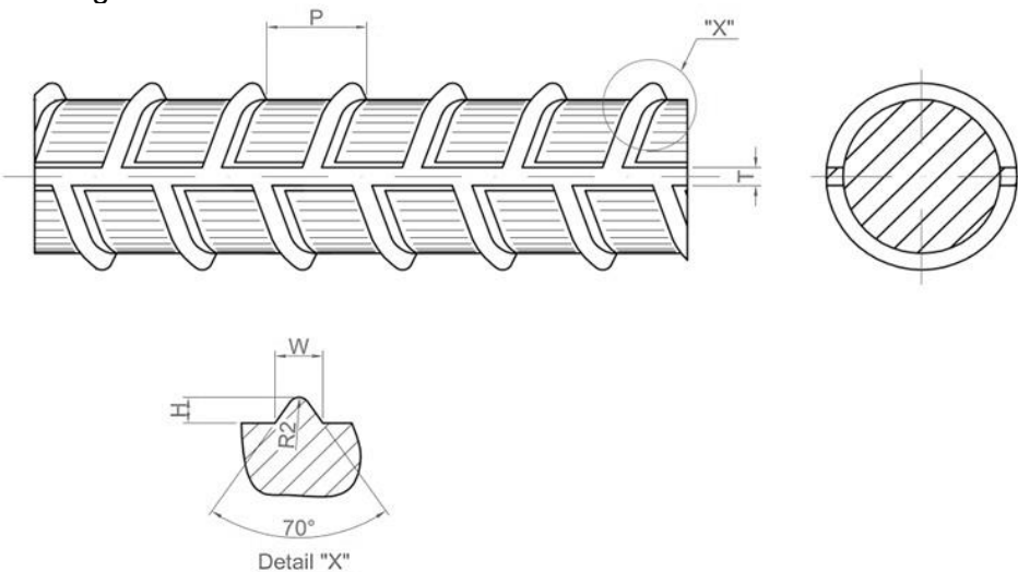
Gambar 3 – Jenis baja tulangan beton sirip/ulir curam
