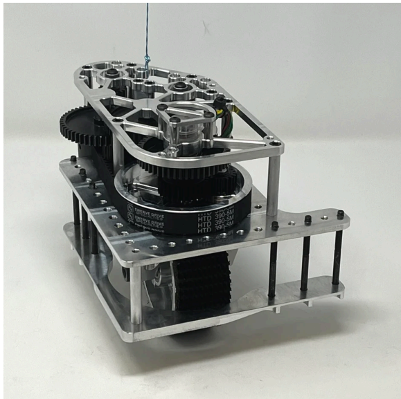
MK4n Swerve Module:
