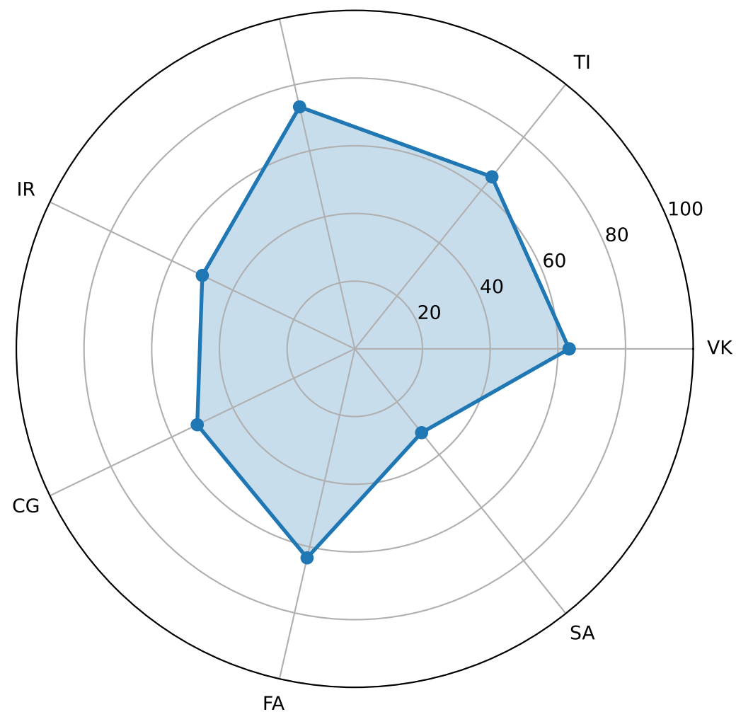
DeepSeek-V2
