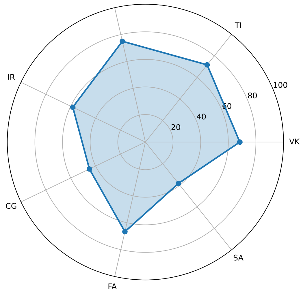
Gemini-1.5-Pro
