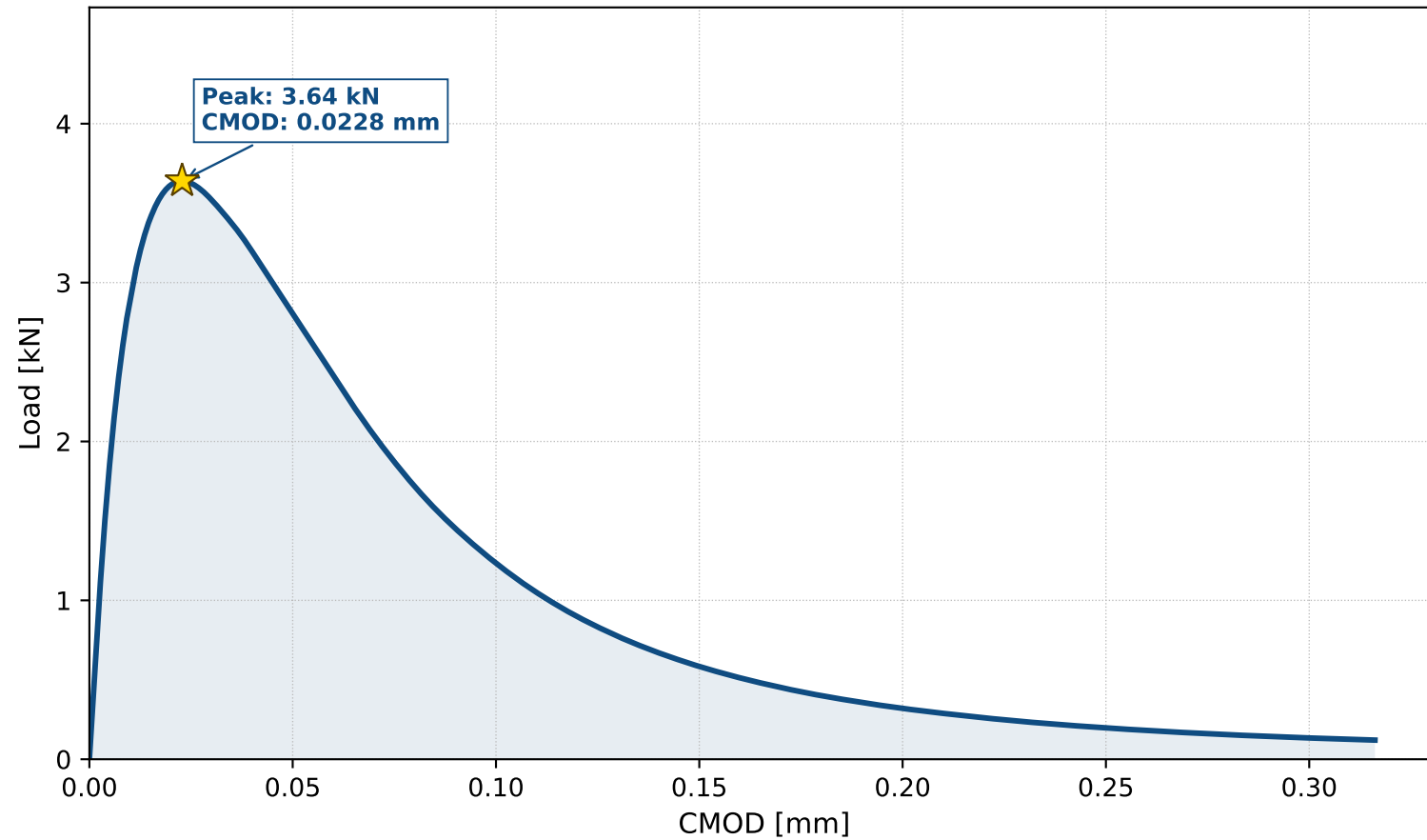
MATLAB - FRACMATH
