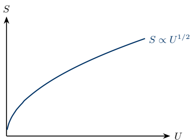
S-U-mitad
