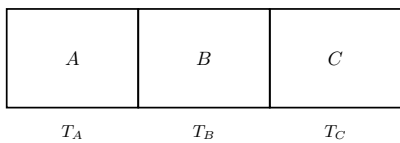
ley-cero
