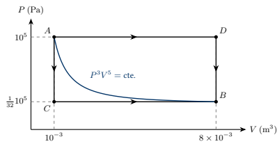
PV-ejemplo
