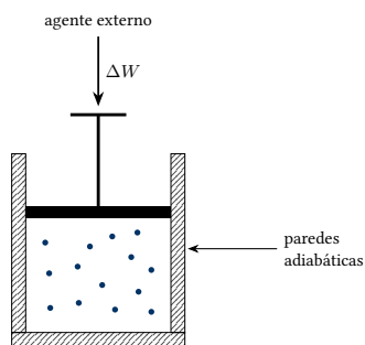
trabajo-adiabático
