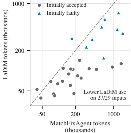
(b) Tokens per input
